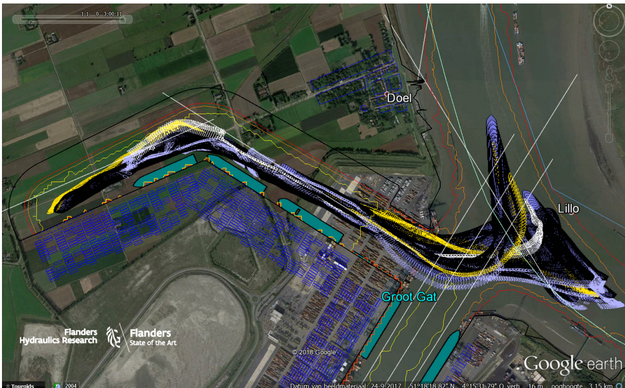
Figuur 7 – Samengestelde tracks van runs VP9_3000 en VP9_3001 voor SIM360+ en SIM225
