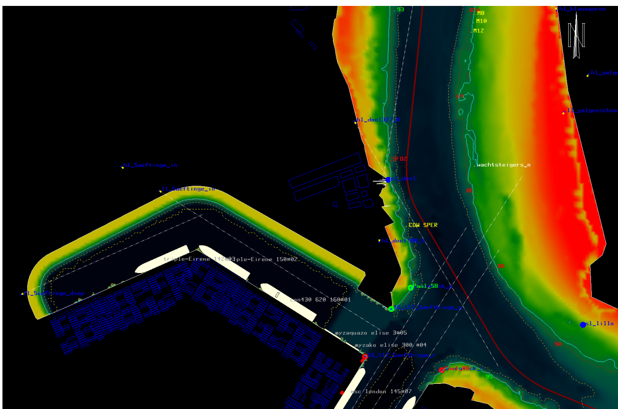
Figuur 2 - Variant P9-3 voor het tweede getijdendok
