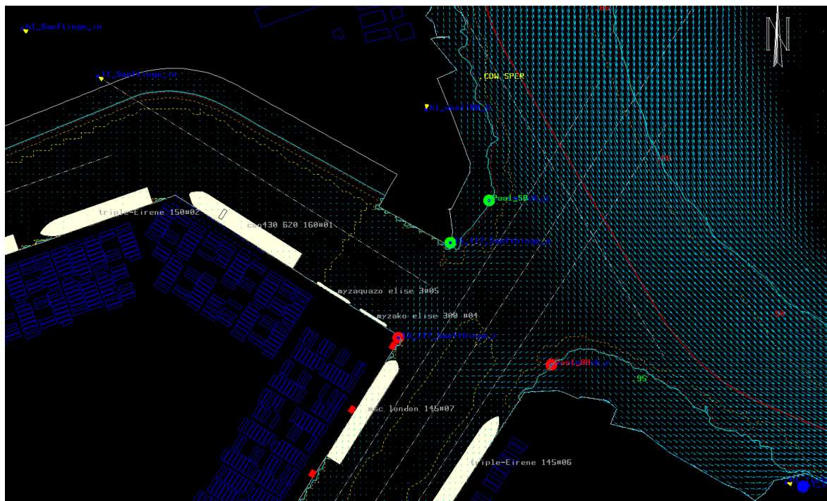
Maximale vloedstroom, Vloed_115
