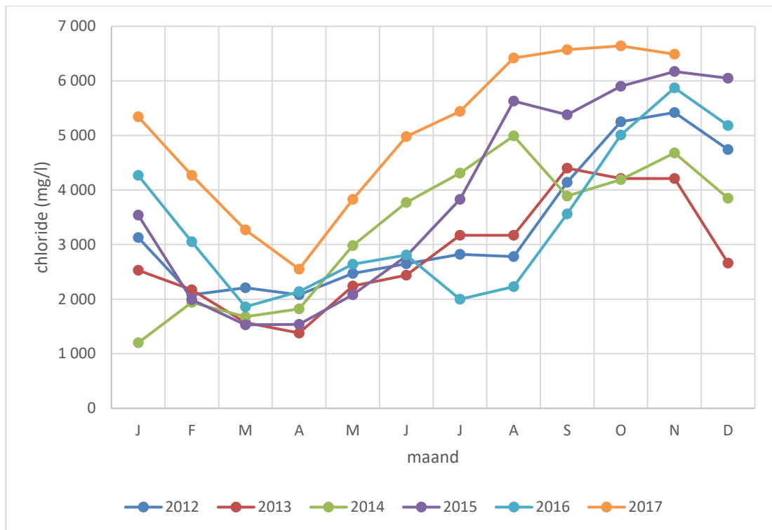
Figuur 75 Seizoensale evolutie van het chloridegehalte in het Kanaaldok op Rechteroever, van 2012 tot 2017
