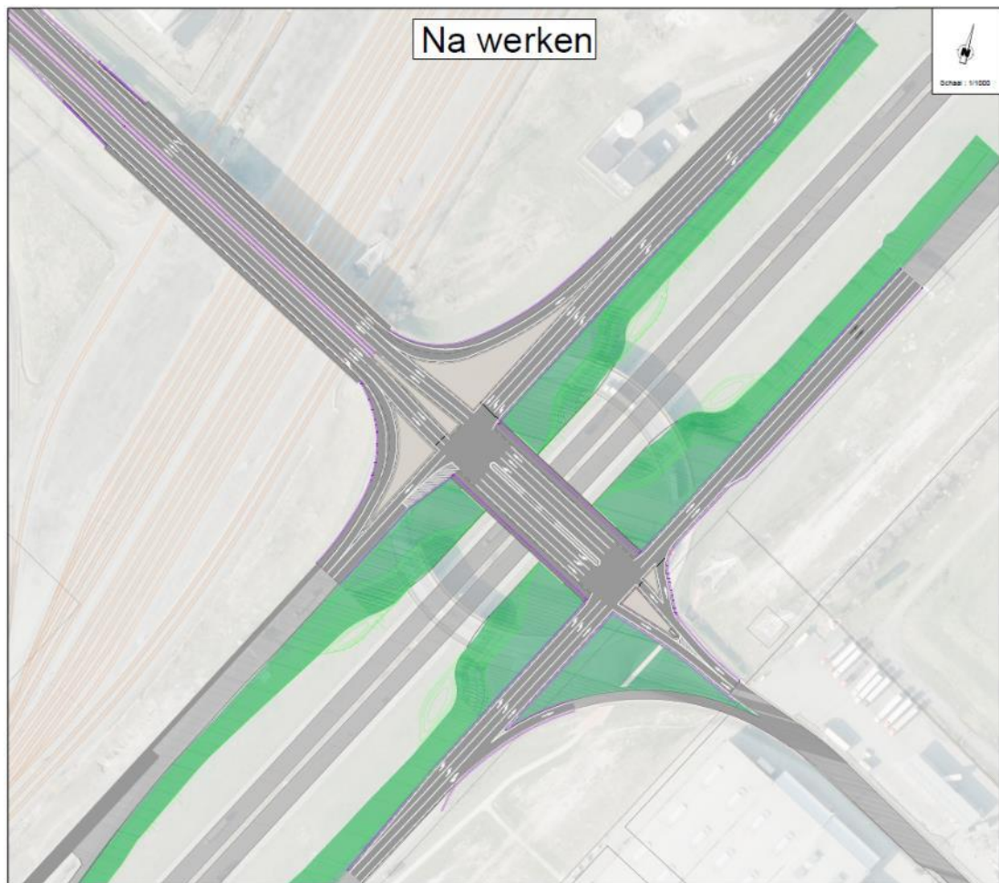
Figuur 112 Ontwerp Waaslandhaven-Noord, plan 16EF/3758 van AMT
