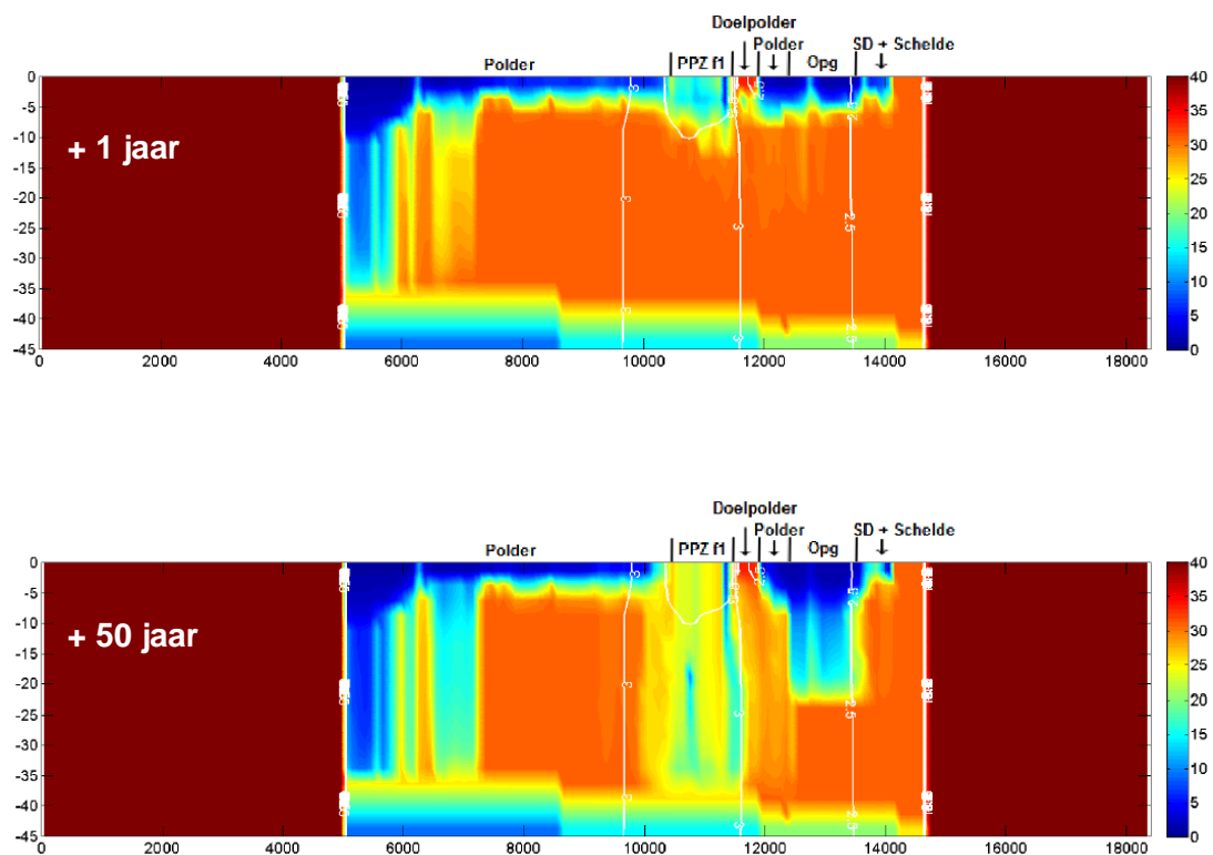
Figuur 100 Evolutie van de zoet-zout waterverdeling op basis van verticale west-oost doorsnede ter hoogte van het Saeftinghedok
