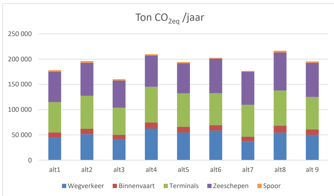
Figuur 337 Totale broeikasgasemissies en bijdrage van de verschillende bronnen voor de negen bestudeerde alternatieven
