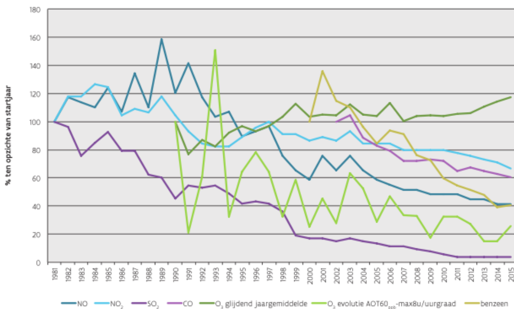
Figuur 153 Trend qua concentraties gasvormige pollutanten (bron VMM).
