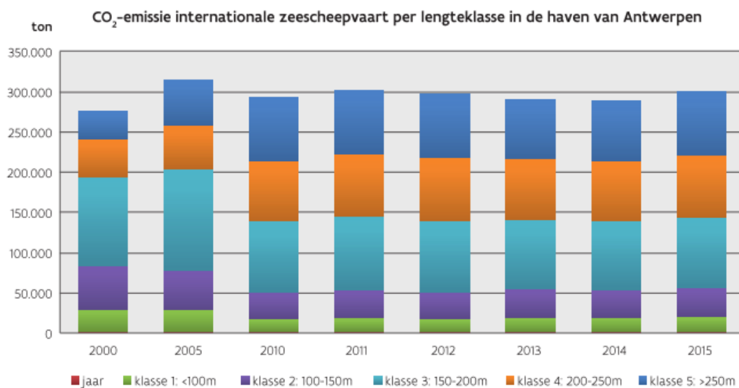
Figuur 151 Evolutie CO 2 emissies zeescheepvaart per scheepstype en per lengteklasse in de HvA (bron VMM)
