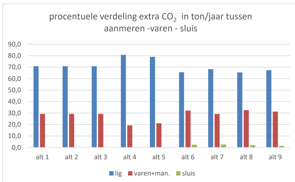
Figuur 162 Relatieve CO 2 emissies zeevaart per alternatief bij aangemeerd liggen, varen+manoeuvres en t.h.v. de sluis.
