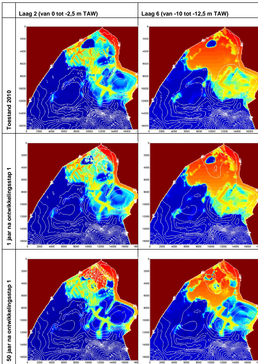
Figuur 87 Evolutie van de zoet-zout waterverdeling in laag 2 (van 0 tot -2,5 m TAW) en laag 6 (van -10 tot -12,5 m TAW) voor de toestand 2010, 1 jaar na ontwikkelingsstap 1 en 50 jaar na ontwikkelingsstap 1 Kleurenschaal is het zoutwaterpercentage, x- en y-coördinaten in m. De witte lijnen stellen de zoetwaterstijghoogtes van deze laag voor.
