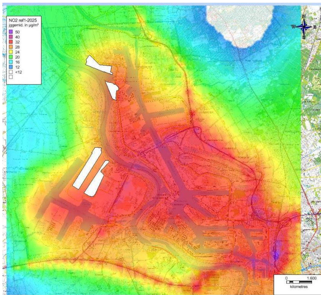
Figuur 339 Jaargemiddelde \text{NO}_2 concentratie in \mu\text{g}/\text{m}^3 voor referentie situatie 1 in 2025 met ligging van de bestaande terminals
