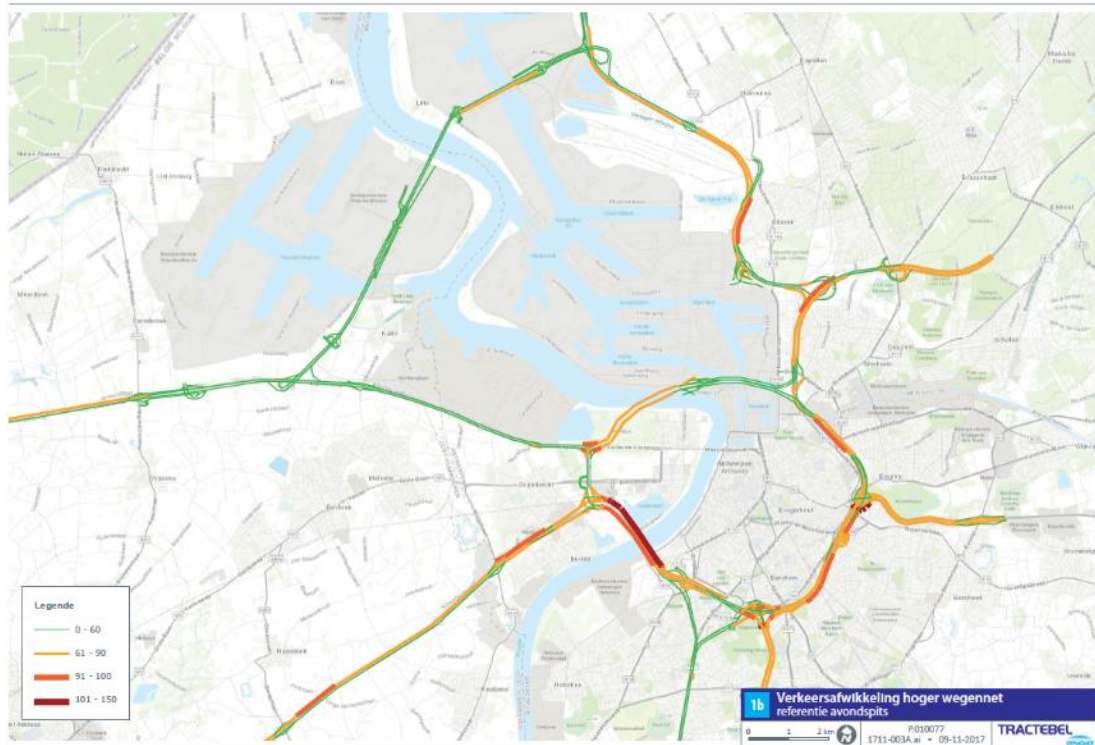
Figuur 130 Kwaliteit wegennet (snelwegen): Wegvakverzadiging referentiesituatie, avondspits (17u-18u)
