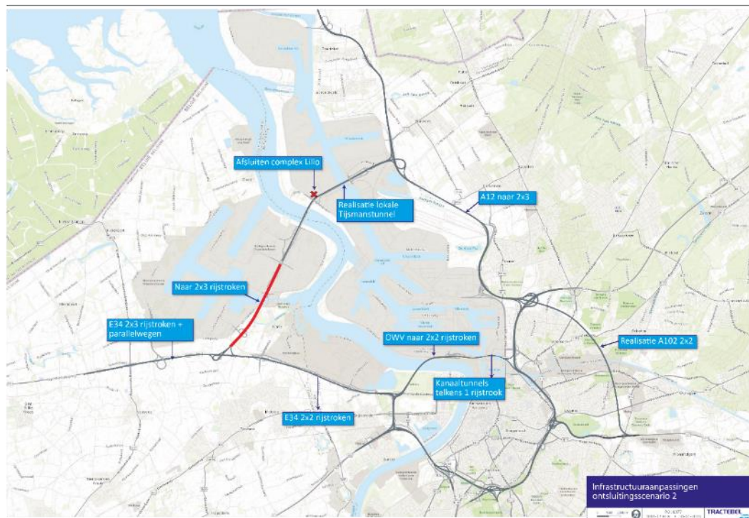
Figuur 116 Aanpassingen infrastructuur ontsluitingsscenario 1 tov huidige situatie
