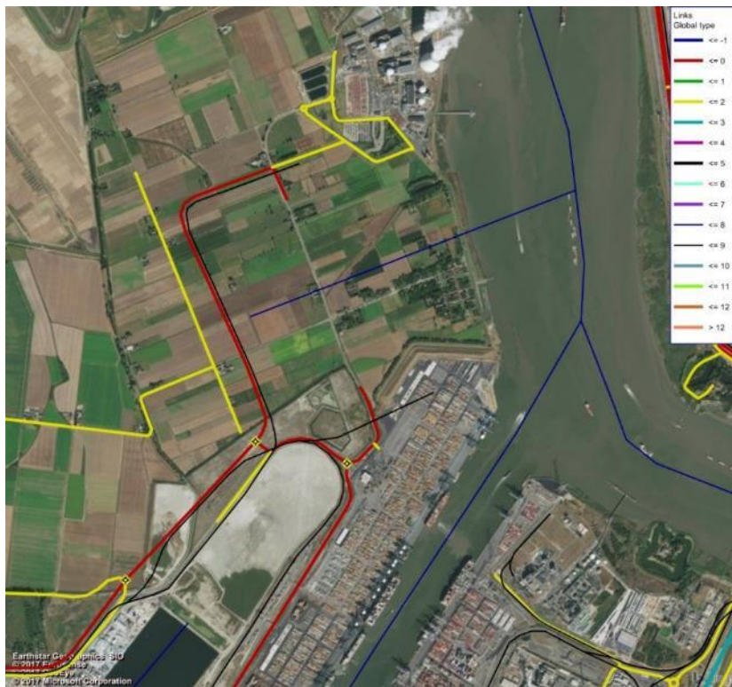
Figuur 118 Havenmodel noordzijde Waaslandhaven - Doel (rood = verbindingsweg, geel = lokale weg, blauw = water, zwart = spoor)
