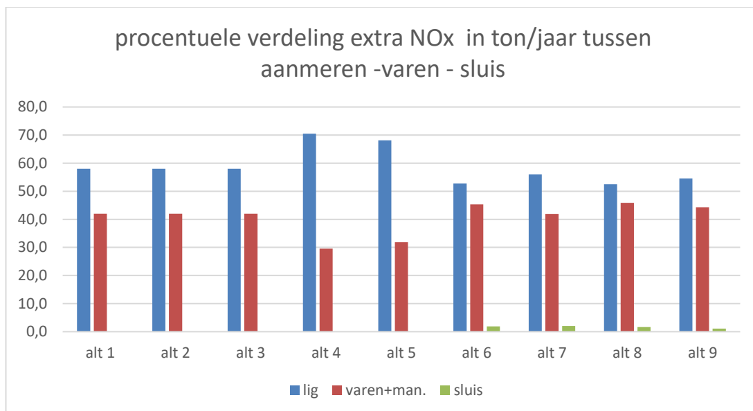
Figuur 160 Relatieve NOx emissies zeevaart per alternatief bij aangemeerd liggen, varen+manoeuvres en t.h.v. de sluis.
