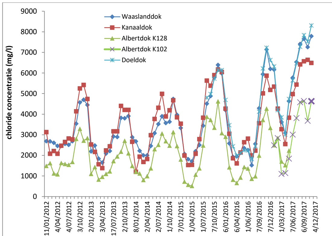
Figuur 74 Evolutie van het chloridegehalte in de dokken op Linker- en Rechteroever, van 2012 tot 2017
