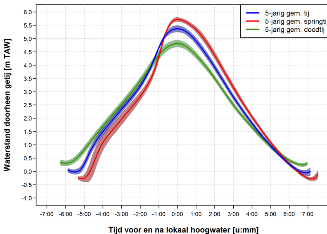
Figuur 63 Gemiddelde tijkrommen gemeten in het meetpunt ‘Antwerpen-Loodsgebouw’
