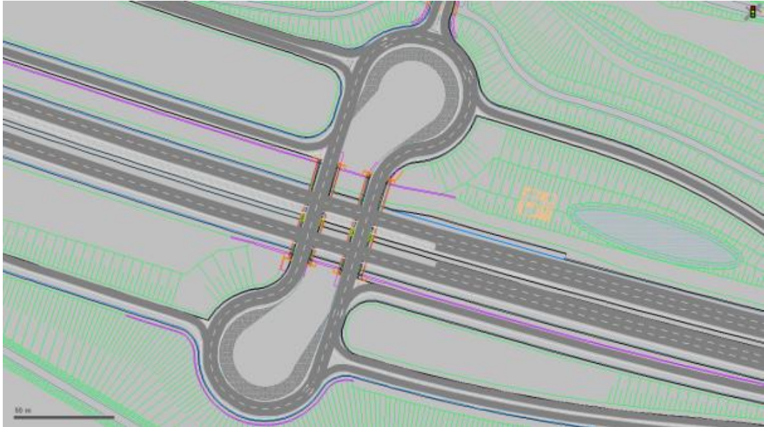
Figuur 113 Ontwerp complex Waaslandhaven-Oost
