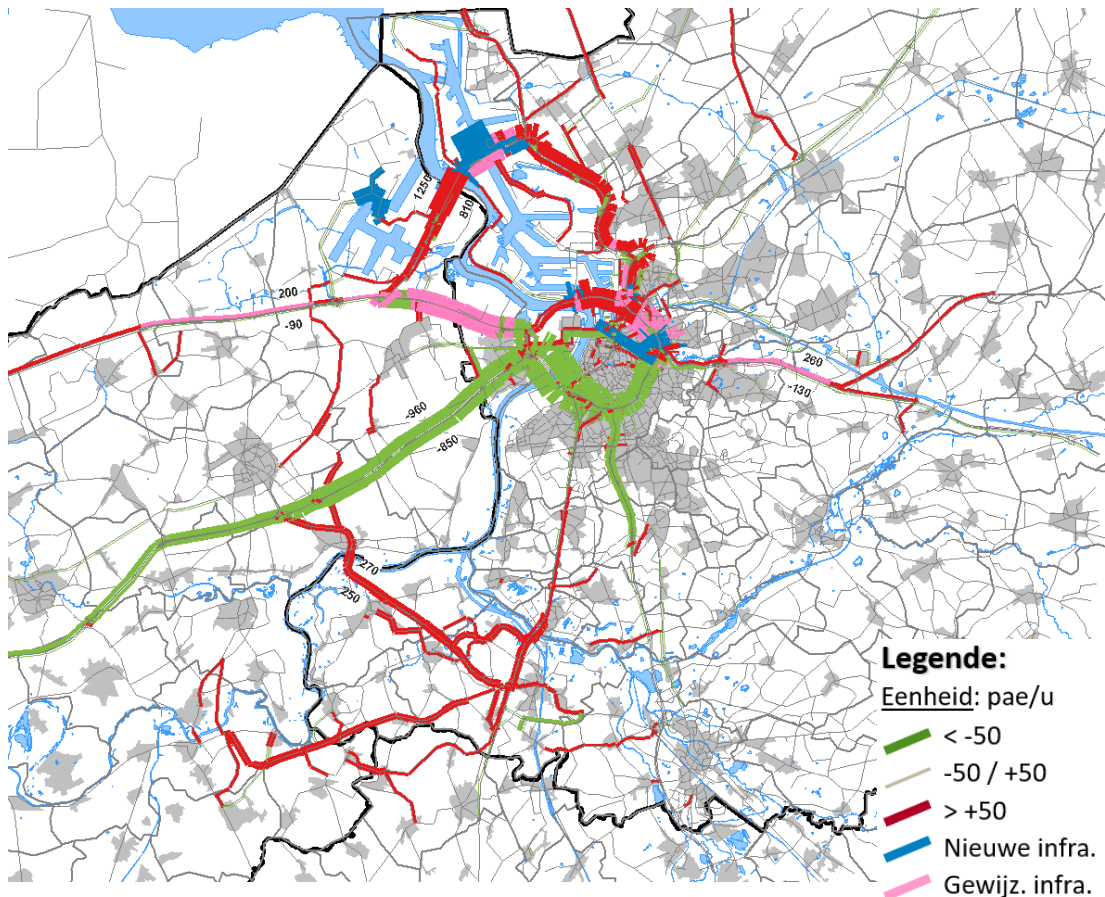
Figuur 141 Verschillenplot Ontsluitingsscenario 1 versus “voorkeursscenario” (zonder AMS), ochtendspitsuur (8u-9u)
