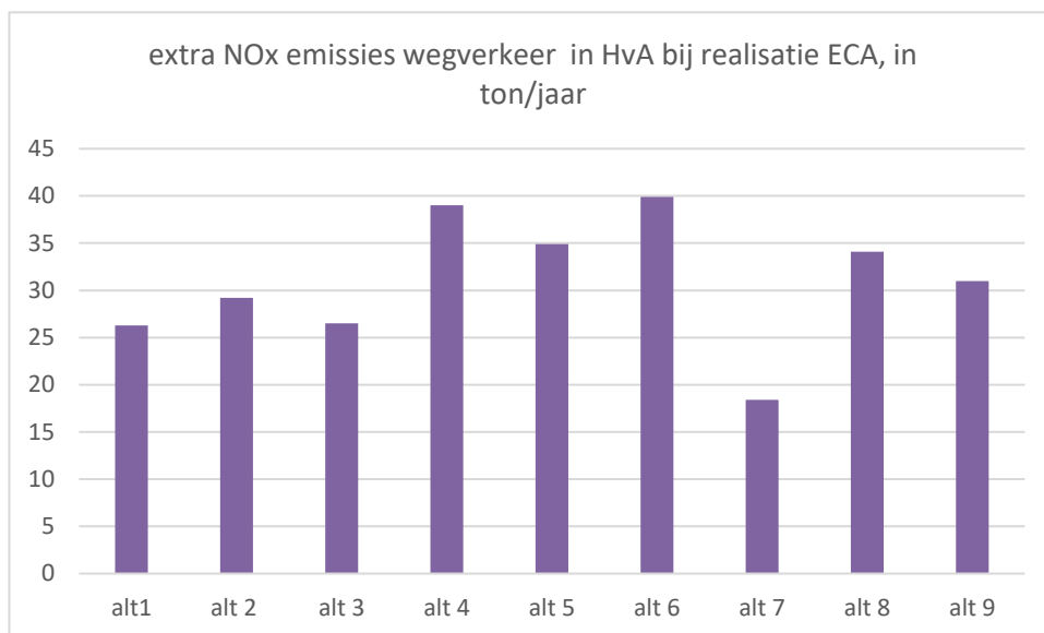
Figuur 165 Extra NOx emissies wegverkeer per alternatief, in ton/jaar
