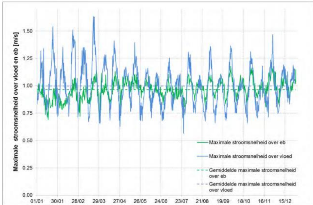
Figuur 67 Maximale stroomsnelheid over vloed en over eb te Oosterweel (Beneden-Zeeschelde), bovenste meettoestel (2015)
