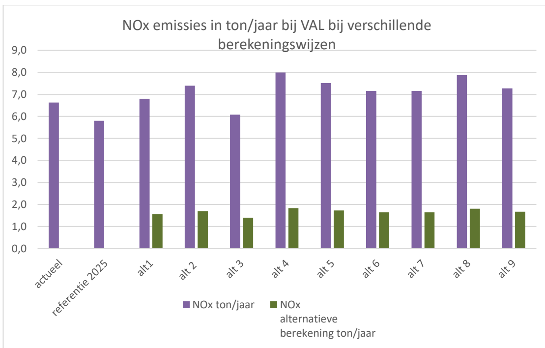
Figuur 171 NOx emissie bij VAL bij verschillende alternatieven berekend op twee onderscheiden manieren (worst case of met inzet louter nieuwe machines die aan strengste EU-grenswaarden voldoen)
