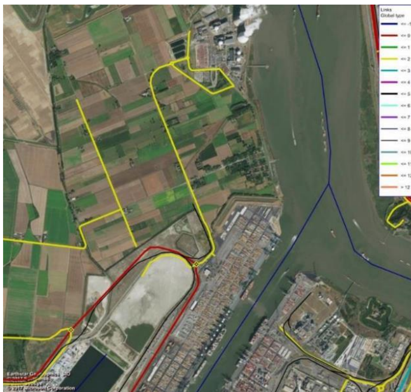
Figuur 122 Havenmodel noordzijde Waaslandhaven - Doel (rood = verbindingsweg, geel = lokale weg, blauw = water, zwart = spoor)
