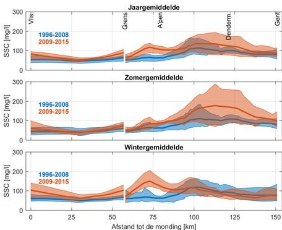
Figuur 73 Langsverdeling van sedimentconcentraties in het gehele Schelde-estuarium (naar Cox et al., 2015). Brede lijn geeft het gemiddelde weer; gekleurde gebieden geven de 10e en 90ste percentiel van de jaargemiddelden weer over de beschouwde periode. (IMDC, 2017, Voortgangrapportage 2014-2015: Synthese Rapport, Monitoringsprogramma Flexibelstorten, I/RA/11353/16117/THL)
