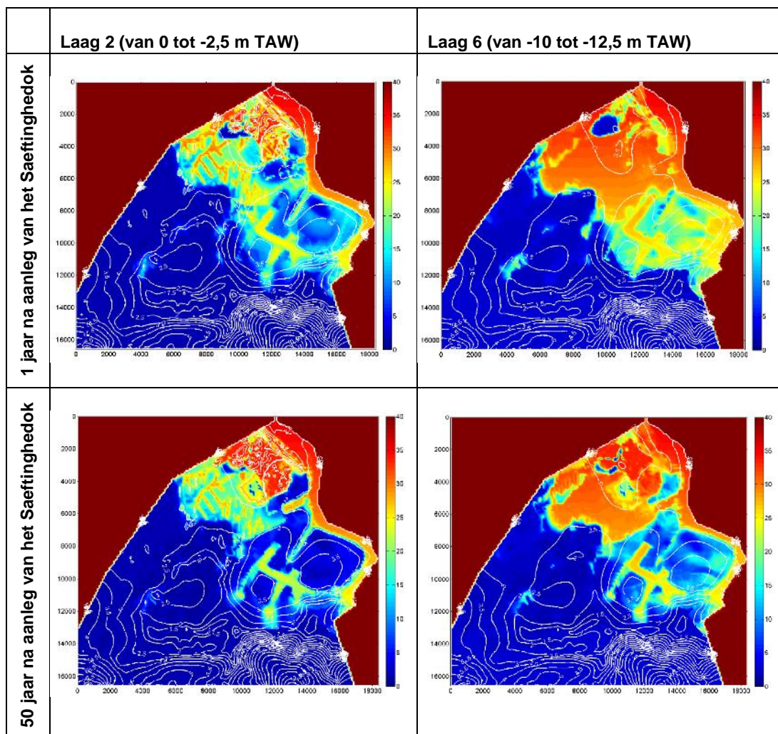
Figuur 98 Evolutie van de zoet-zout waterverdeling in laag 2 (van 0 tot -2,5 m TAW) en laag 6 (van -10 tot -12,5 m TAW) voor de toestand 2010, 1 jaar na ontwikkelingsstap 1 en 50 jaar na ontwikkelingsstap 1 Kleurenschaal is het zoutwaterpercentage, x- en y-coördinaten in m. De witte lijnen stellen de zoetwaterstijghoogtes van deze laag voor.
