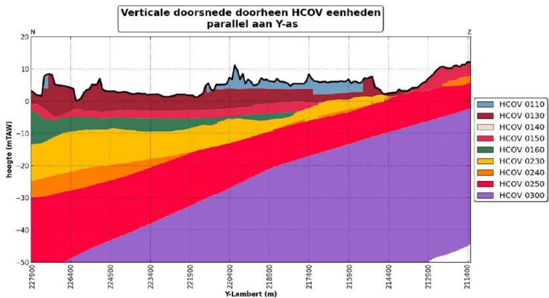
Figuur 79 Verticale (hydro)geologische doorsnede door de Waaslandhaven
