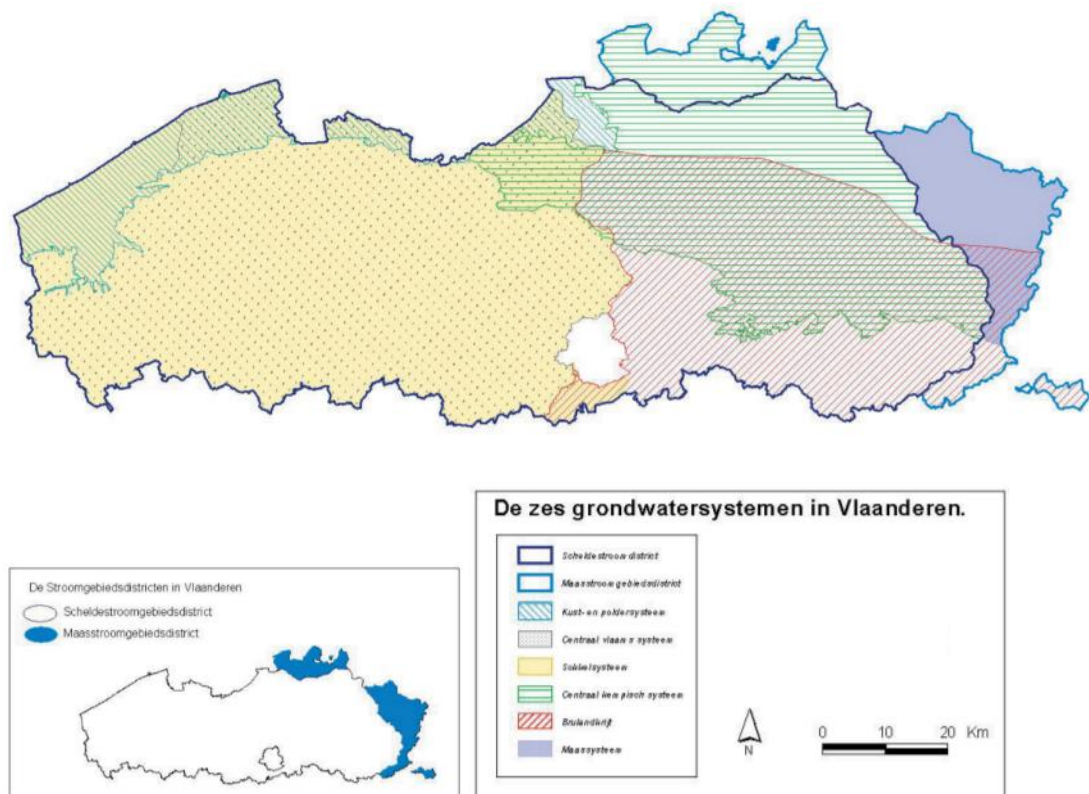
Figuur 76 Grondwatersystemen in Vlaanderen
