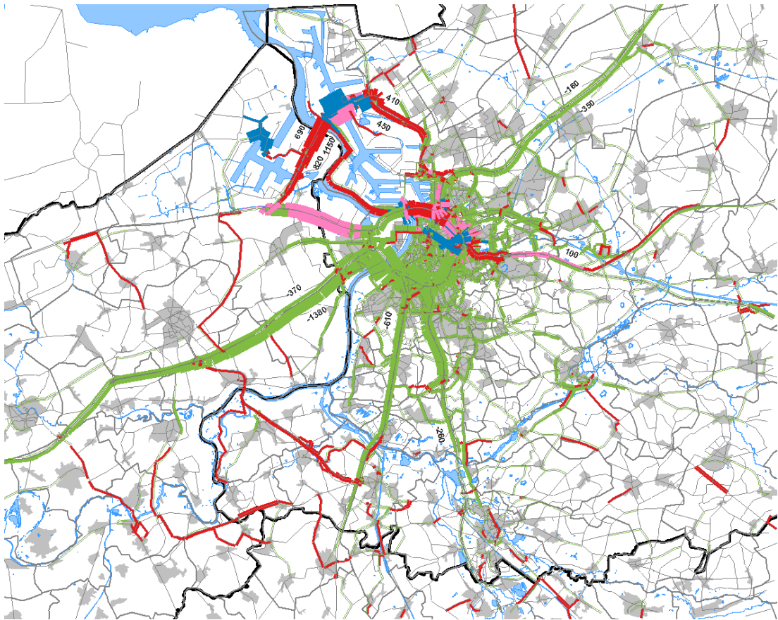
Figuur 146 Versillenplot Ontsluitingsscenario 1 versus “voorkeursscenario”, avondspitsuur (17u-18u)
