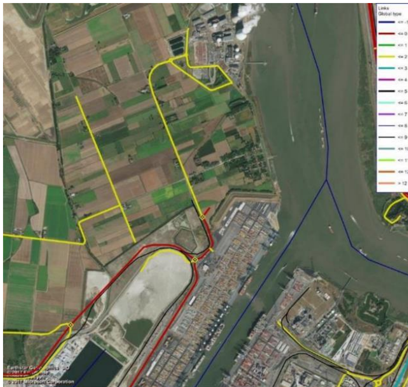
Figuur 121 Havenmodel noordzijde Waaslandhaven - Doel (rood = verbindingsweg, geel = lokale weg, blauw = water, zwart = spoor)
