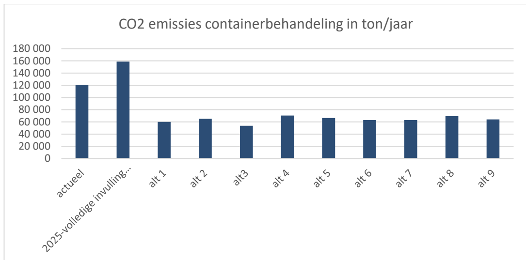
Figuur 170 CO 2 emissies containerbehandeling naargelang het alternatief
