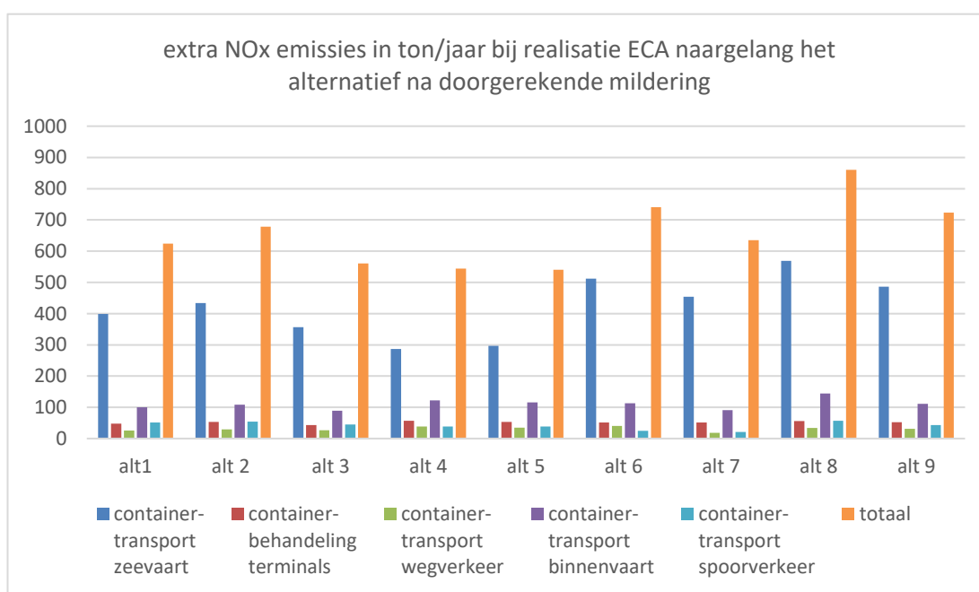
Figuur 157 Extra NOx emissies bij realiseren ECA per alternatief en per bron (excl. VAL en gebouwverwarming) bij toepassen van mildering
