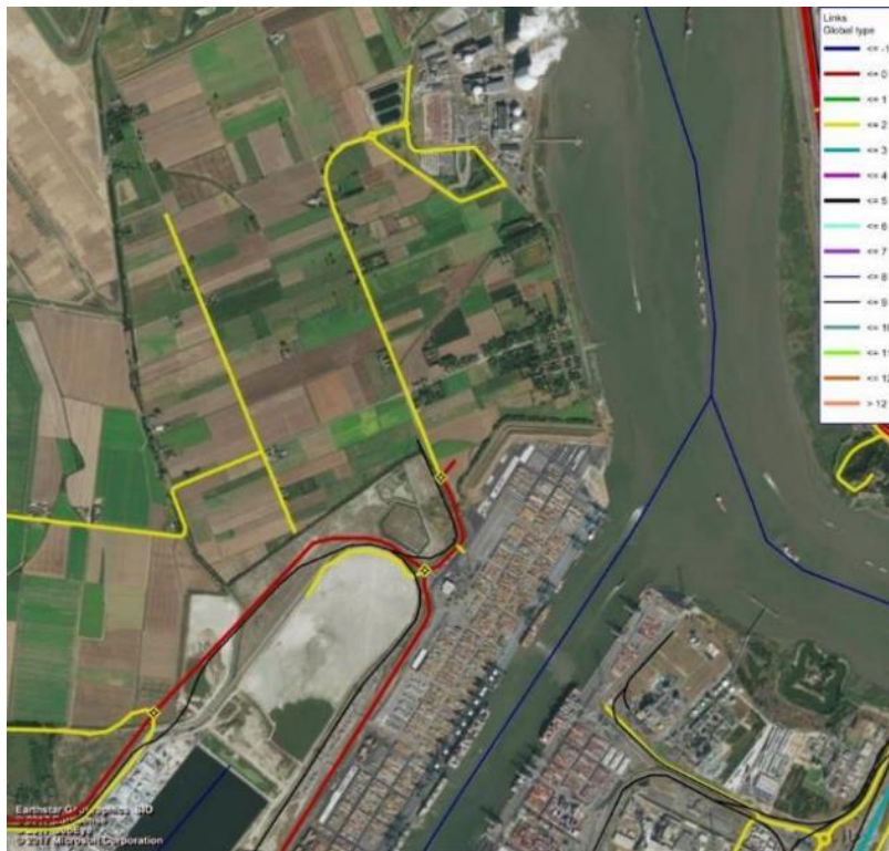
Figuur 123 Havenmodel noordzijde Waaslandhaven - Doel (rood = verbindingsweg, geel = lokale weg, blauw = water, zwart = spoor)
