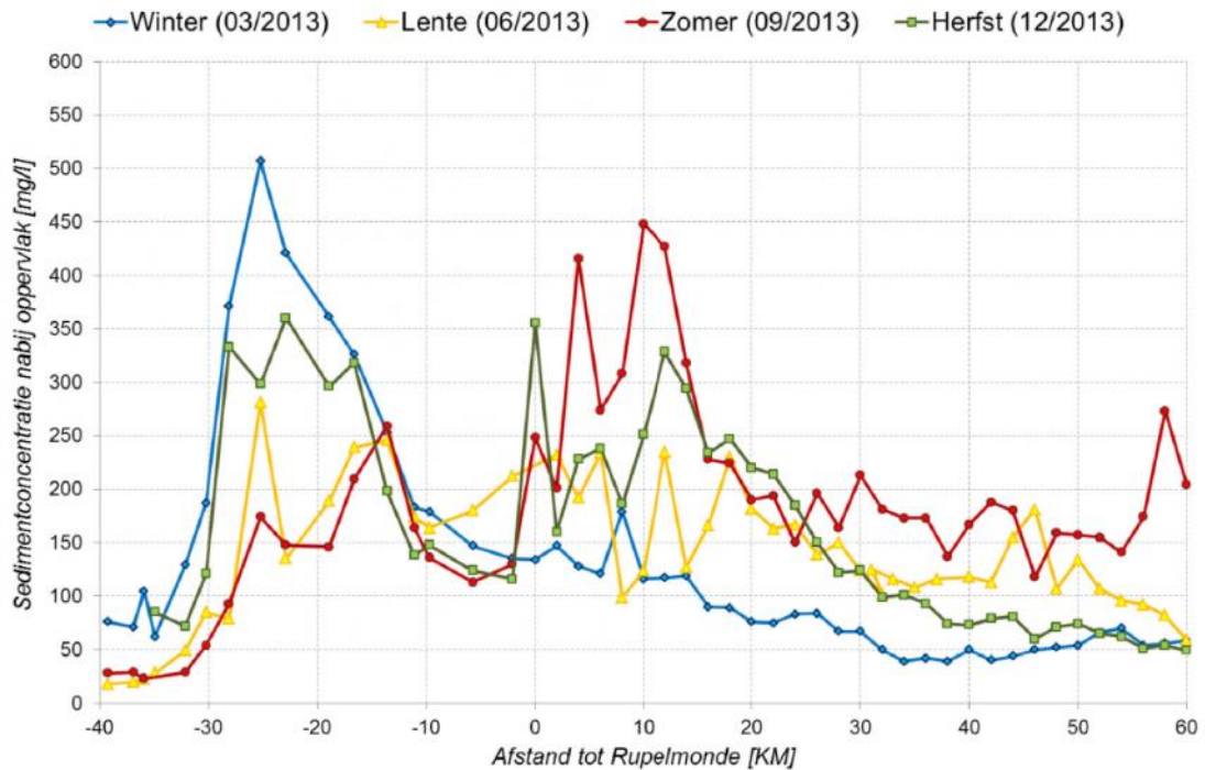
Figuur 68 Overzicht sedimentconcentratie Beneden-Zeeschelde halftij-eb 2013 (Plancke, Vereecken, Vanlede, Verwaest, & Mostaert, 2014)
