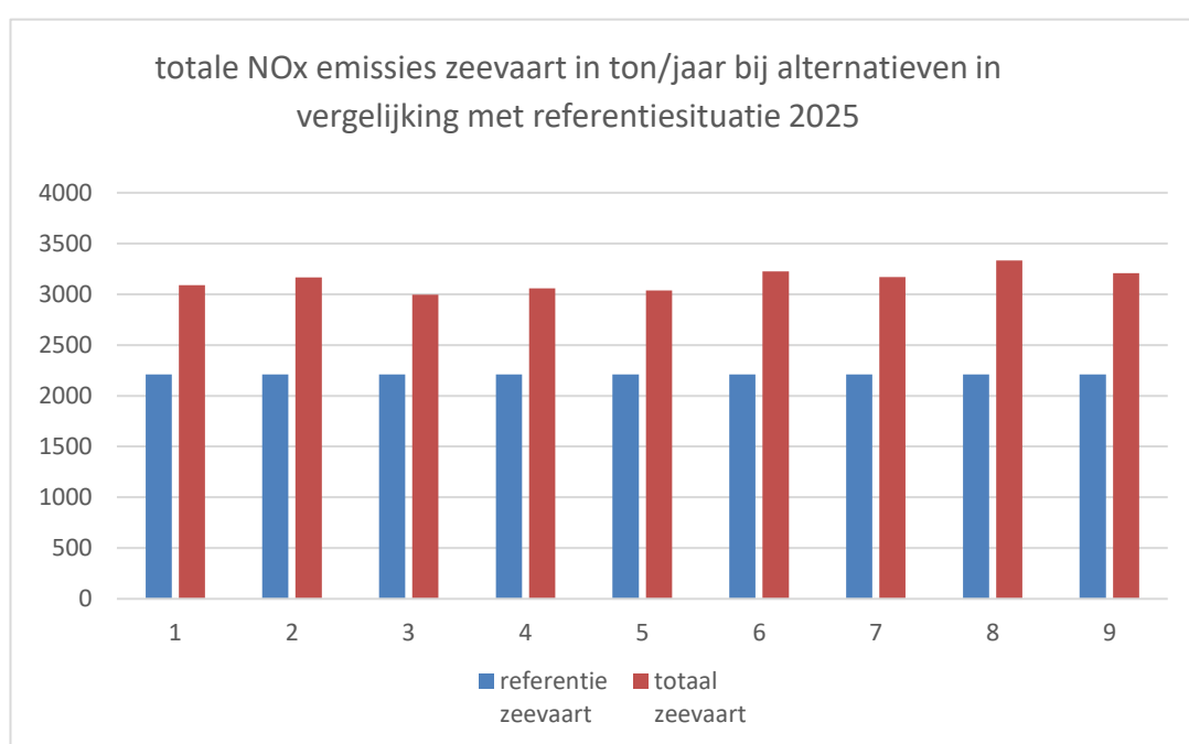
Figuur 159 NOx-emissies zeevaart in ton/jaar veroorzaakt bij de verschillende alternatieven
