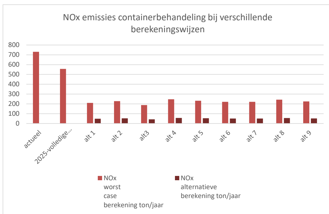
Figuur 169 NOx emissies containerbehandeling naargelang het alternatief berekend op twee onderscheiden manieren (worst case of met inzet louter nieuwe machines die aan strengste EU-grenswaarden voldoen)
