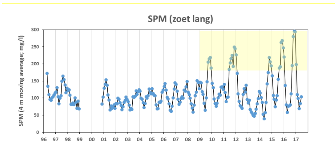
Figuur 70 Zwezende stof concentratie in de zoete zone met lange verblijftijd.
