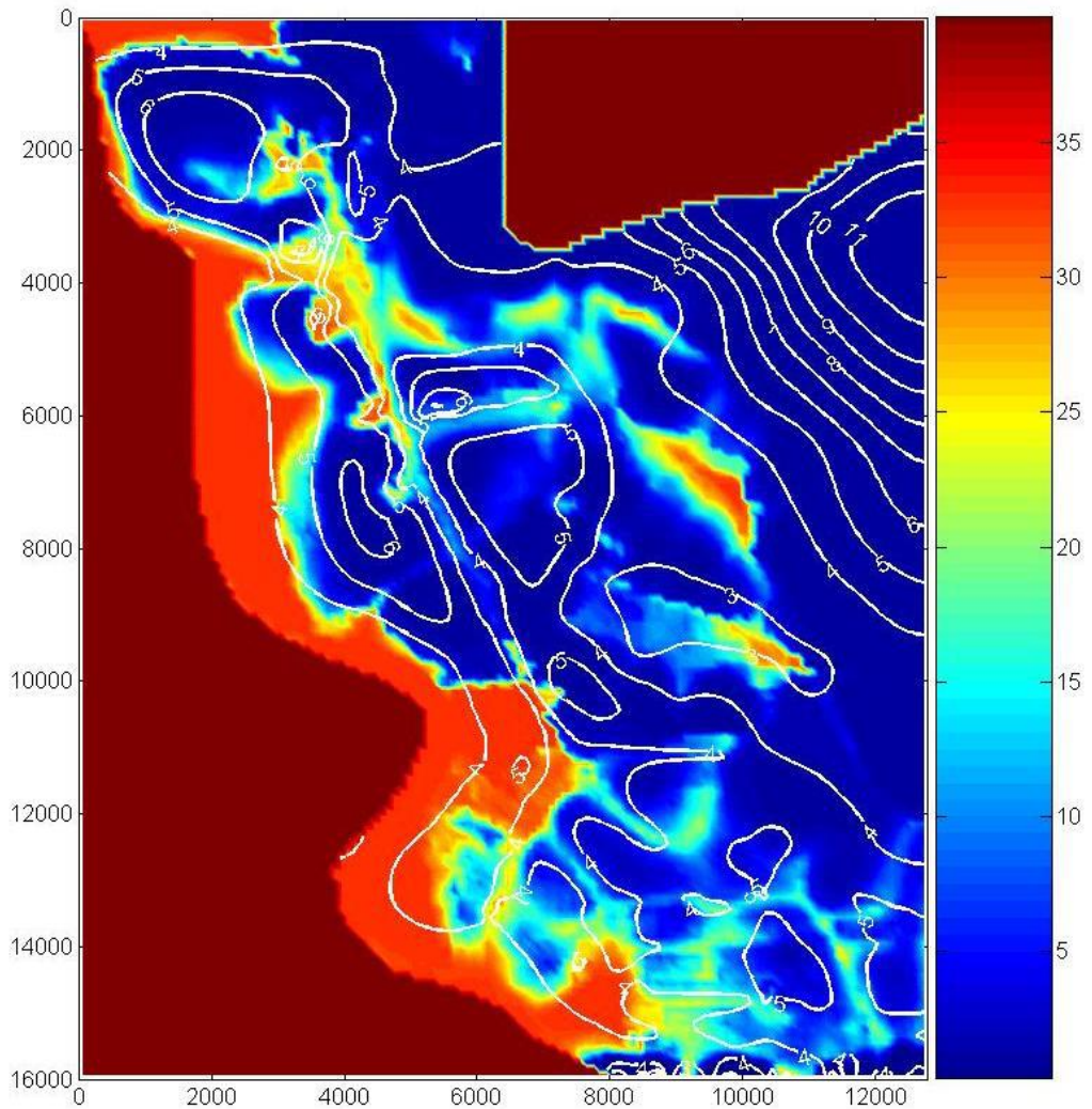
Figuur 91 Gemiddelde zoetwaterstijghoogte (witte contourlijnen in m TAW) en zoutwaterpercentage van laag 5 (-15 tot -20 m TAW) (kleurenschaal van 0 tot 40 percent) in ca. 2011 op Rechterscheldeoever (X- en Y coördinaten in m) (IMDC, 2012)
