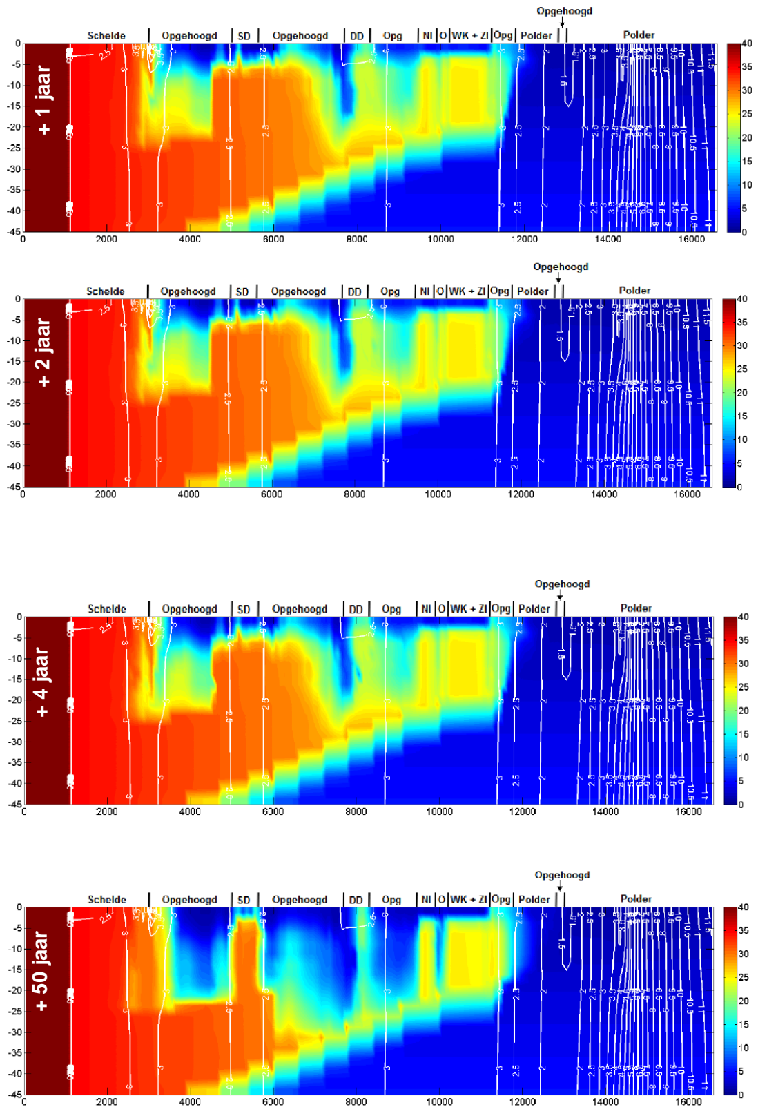
Figuur 99 Evolutie van de zoet-zout waterverdeling op basis van verticale noord-zuid doorsnede doorheen het Saeftinghedok en het centrum van de Waaslandhaven
