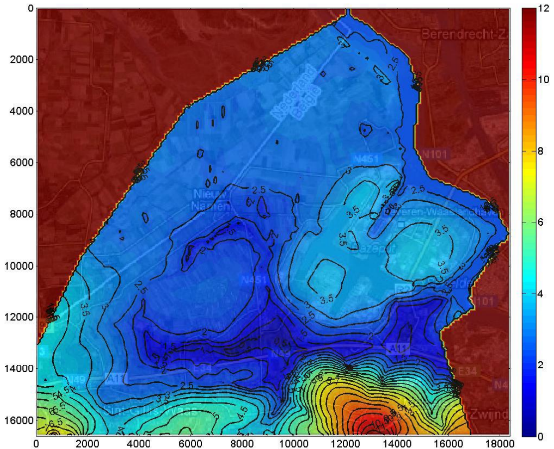
Figuur 82 Zoetwaterstijghoogte van laag 2 (van 0 tot -2,5 m TAW) in 2010
