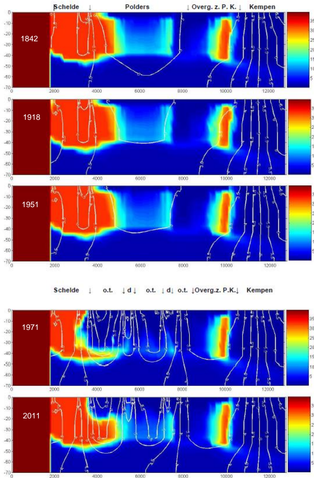
Figuur 94 Gemiddelde zoetwaterstijghoogte (witte contourlijnen in m TAW) en zoutwaterpercentage in verticale doorsnede volgens rij 75 (kleurschaal van 0 tot 40 percent). Van boven naar onder wordt de toestand weergegeven van de jaren ca. 1842, ca. 1918, ca. 1951, ca. 1971 en ca. 2011. (X- en Y - coördinaten in m) (Overg.z. P.K. = Overgangszone Polders – Kempen, o.t. = opgespoten terrein, d = dok)
