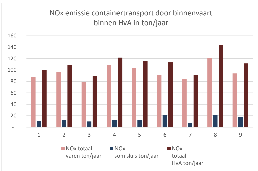
Figuur 163 NOx emissie containertransport door binnenvaart binnen HvA
