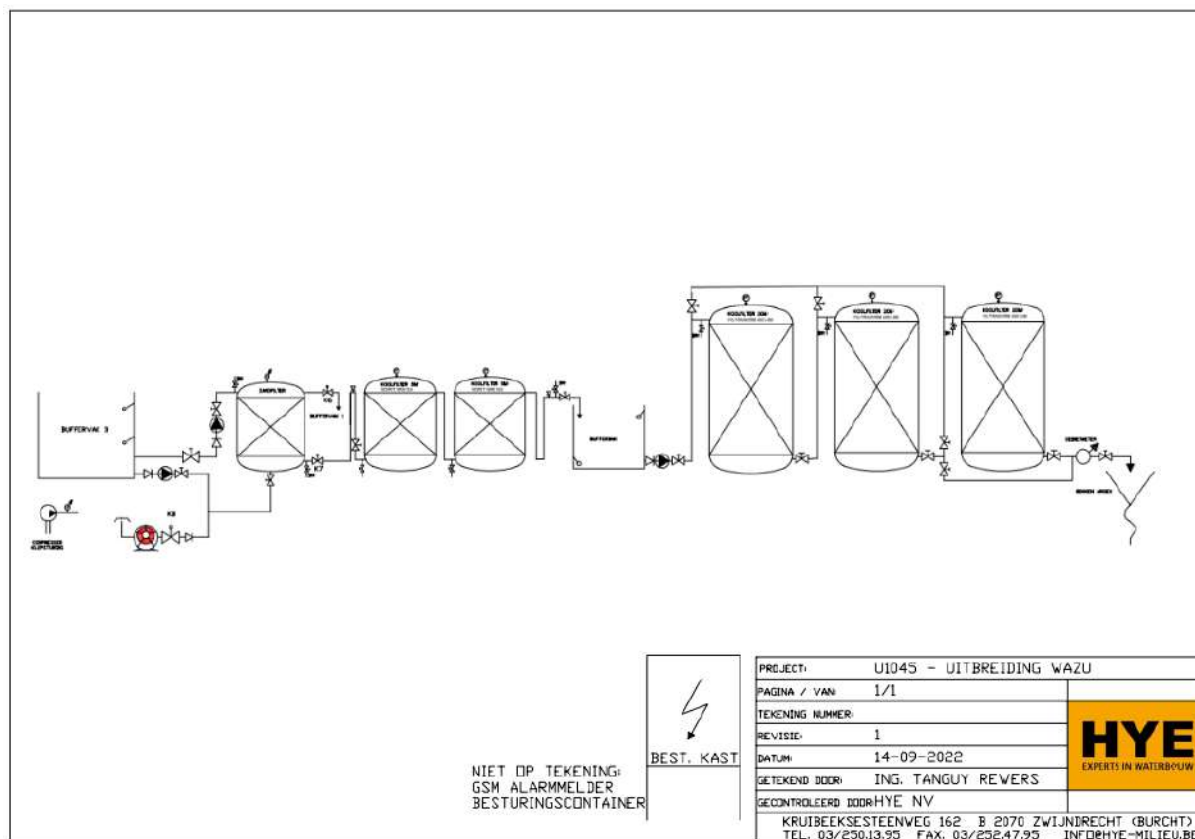
Figuur 21: Flowschema waterzuiveringsinstallatie na uitbreiding met actief koolfilters tbv PFAS-verwijdering.
