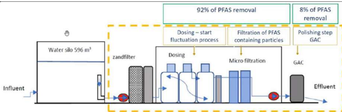
Figuur 1: Waterbehandelingstrein toegepast door HMVT voor de verwijdering van PFAS in grondwater via coagulatie gevolgd door een actief kool nabehandeling.
