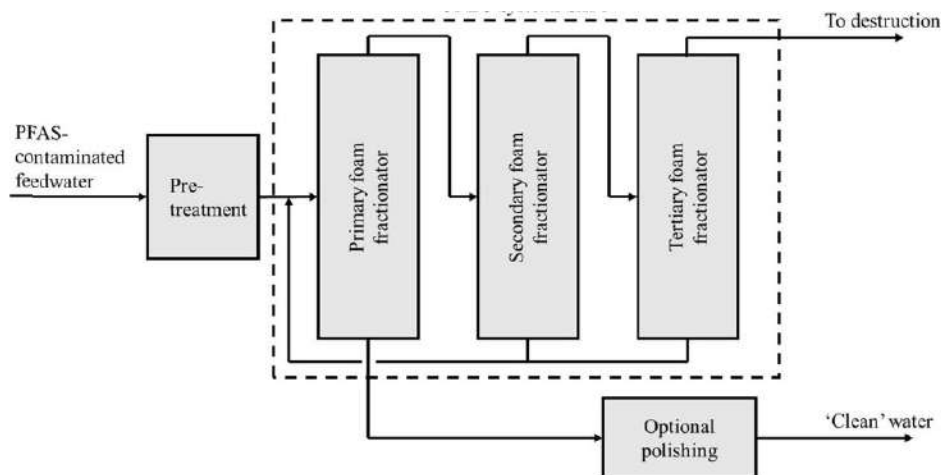
Figuur 2: Vereenvoudigde schematische weergave van meertrapsschuimfractionatie voor de verwijdering van PFAS (Burns et al., 2021).
