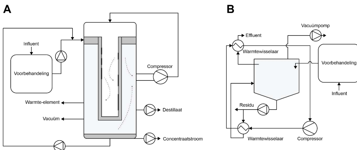
Figuur 20: Vereenvoudigde schematische weergave van (A) mechanische damp recompressie en (B) vacuÛmverdamp(er) (gebaseerd op WASS, 2010).
