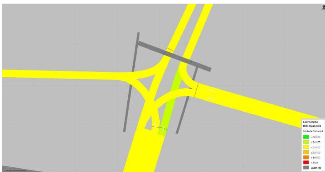
Figuur 205: Verliestijd ASP Melsele Noord
