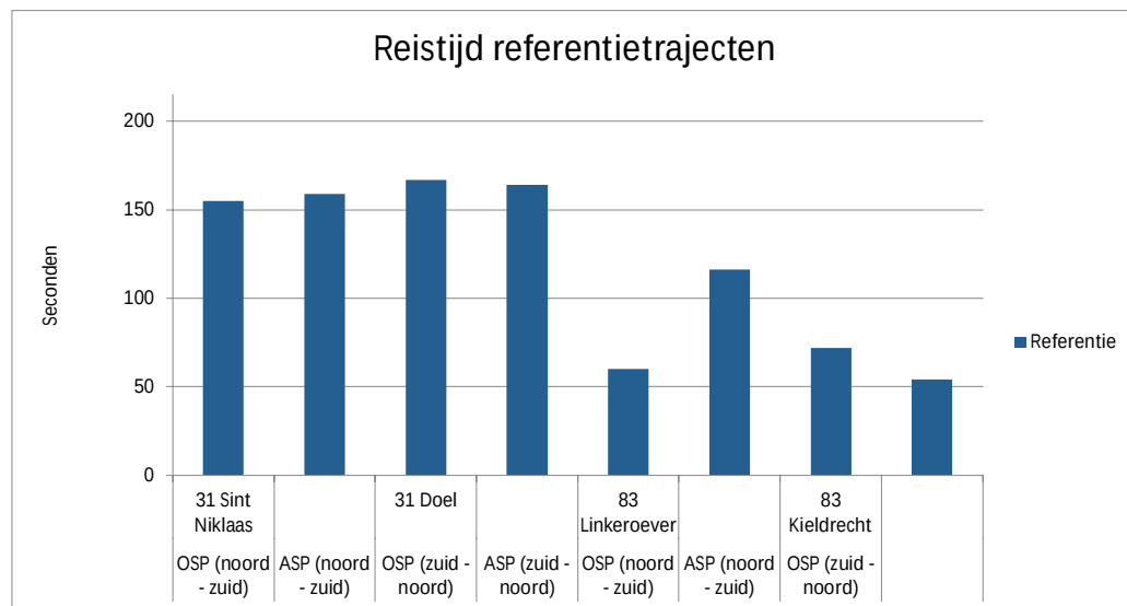
Figuur 6-14: Reistijden op de referentietrajecten – referentietoestand
