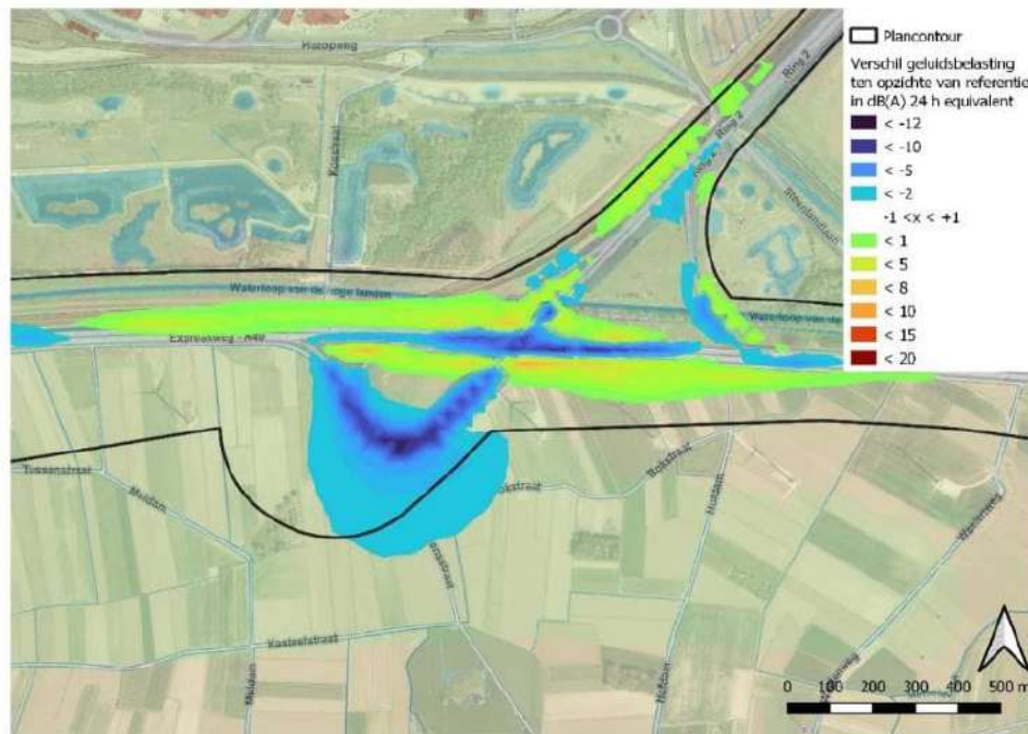
Figuur 6-126 Verschil in geluidsdruk op 1,5 m hoogte voor scenario 1HCc met de compacte aansluiting R2-E34
