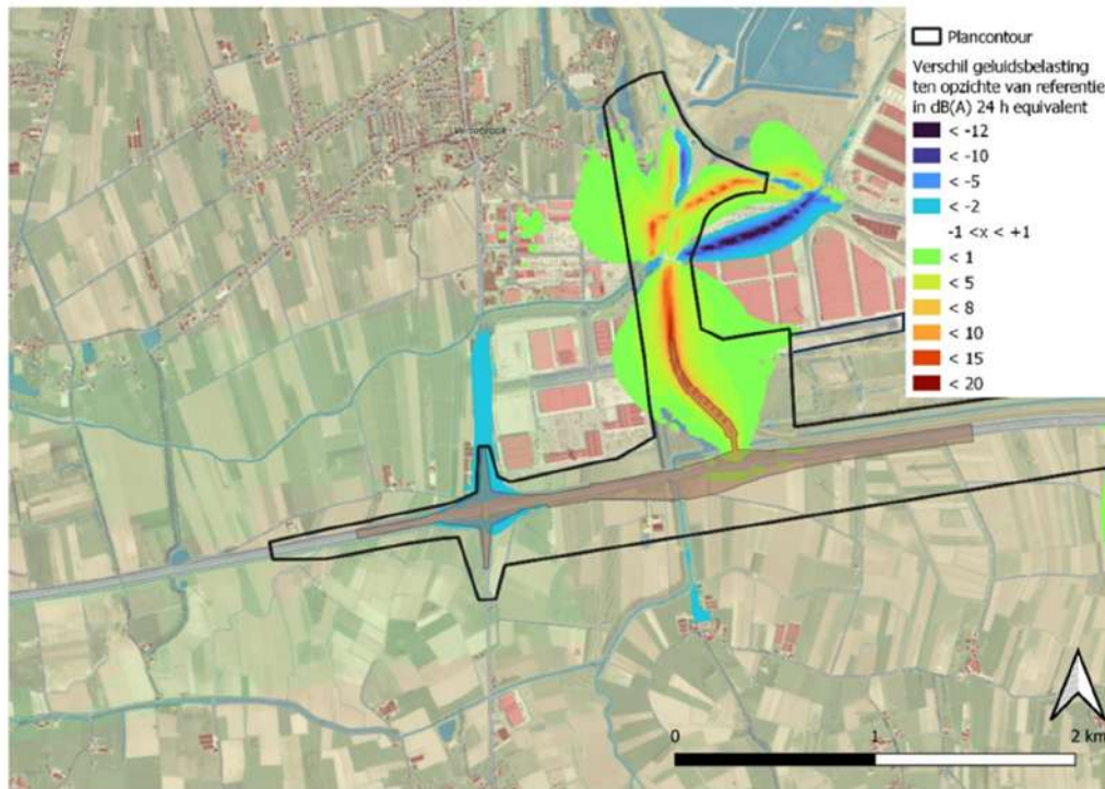
Figuur 6-123 Verskil in geluidsdruk op 1,5 m hoogte voor scenario 1HCc met een ongelijkvloers complex aan Watermolen.
