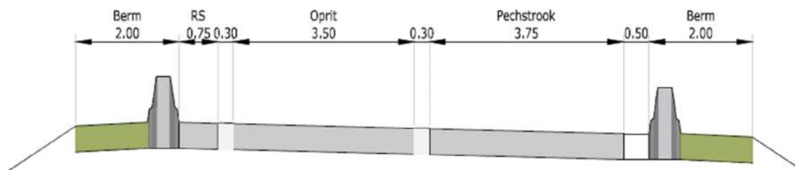
Figuur 3-25: Enkele oprit (indicatief profiel; ontwerp ter onderbouwing van de afbakening van de planologische bestemmingen)
