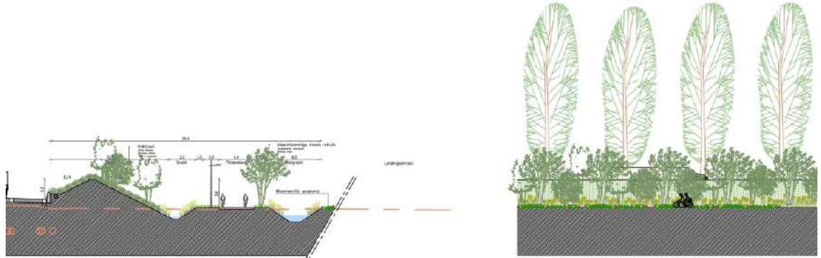
Figuur 3-36 Snede D (ontwerp voorafname ter onderbouwing van de afbakening van de planologische bestemmingen)
