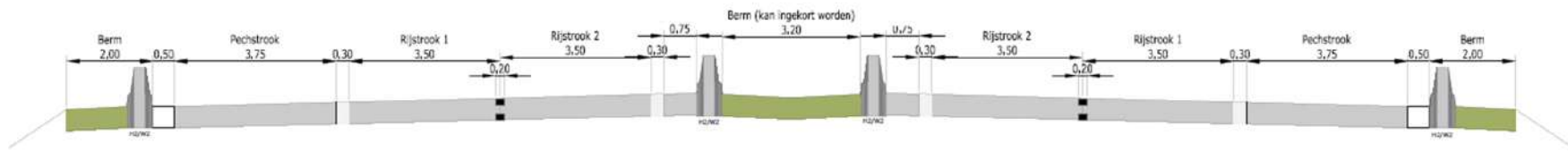
Figuur 3-23: E34 (indicatief profiel; ontwerp voorafname ter onderbouwing van de afbakening van de planologische bestemmingen)
