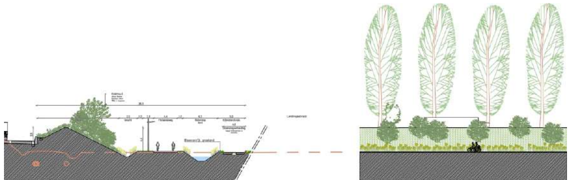
Figuur 3-35 Snede C (ontwerp voorafname ter onderbouwing van de afbakening van de planologische bestemmingen)
