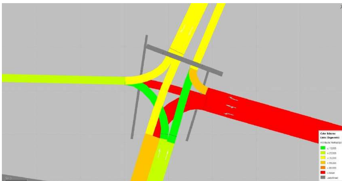
Figuur 224: Verliestijd OSP Melsele Noord
