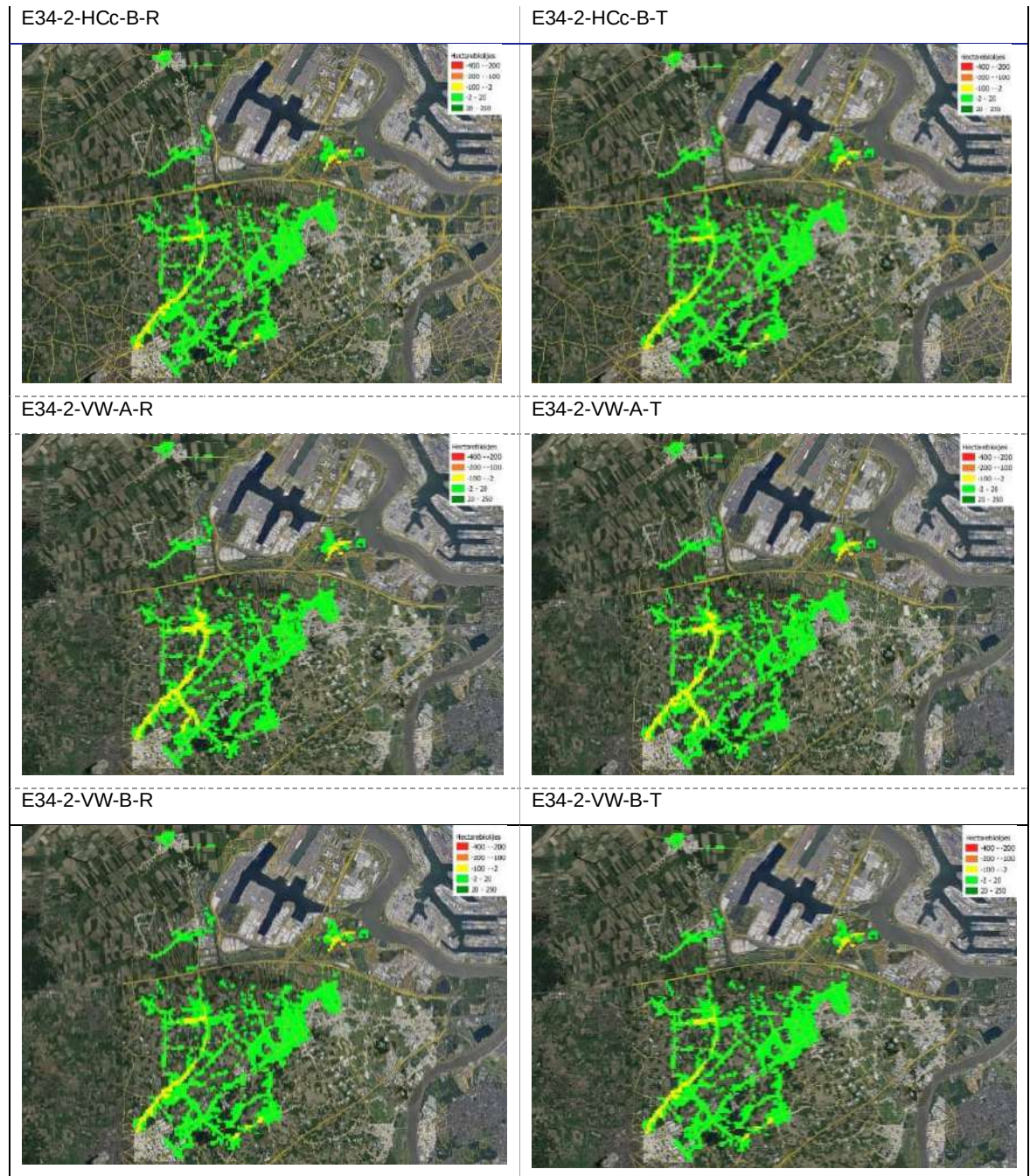
Figuur 6-82 Verskil in geluidsniveaus inrichtingsalternatieven op niveau hectarehokken
