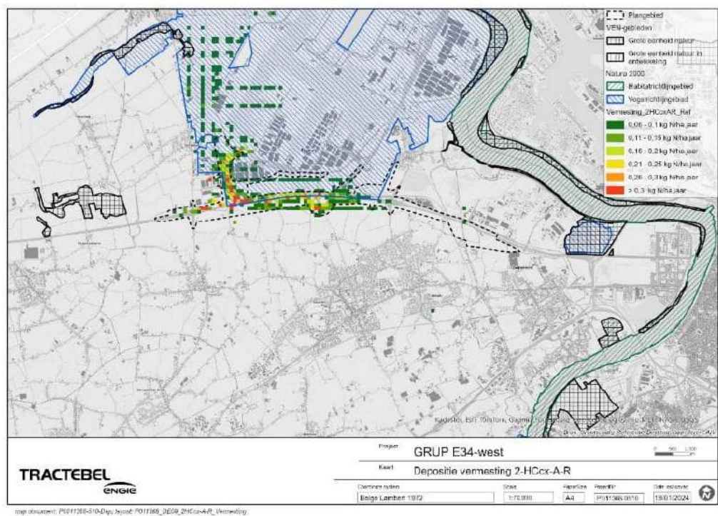
Figuur 6-130 Stikstofdepositietoenames in alternatief 2-HCc-A-R
