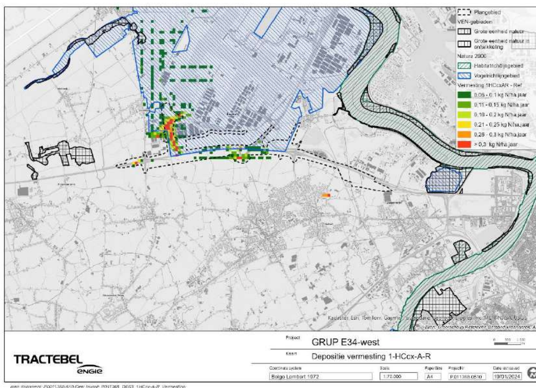
Figuur 5-4 Stikstofdepositietoenames in alternatief 1-HCcx-A-R 5 . De overige alternatieven zijn niet onderscheidend op vlak van stikstofdepositie.
