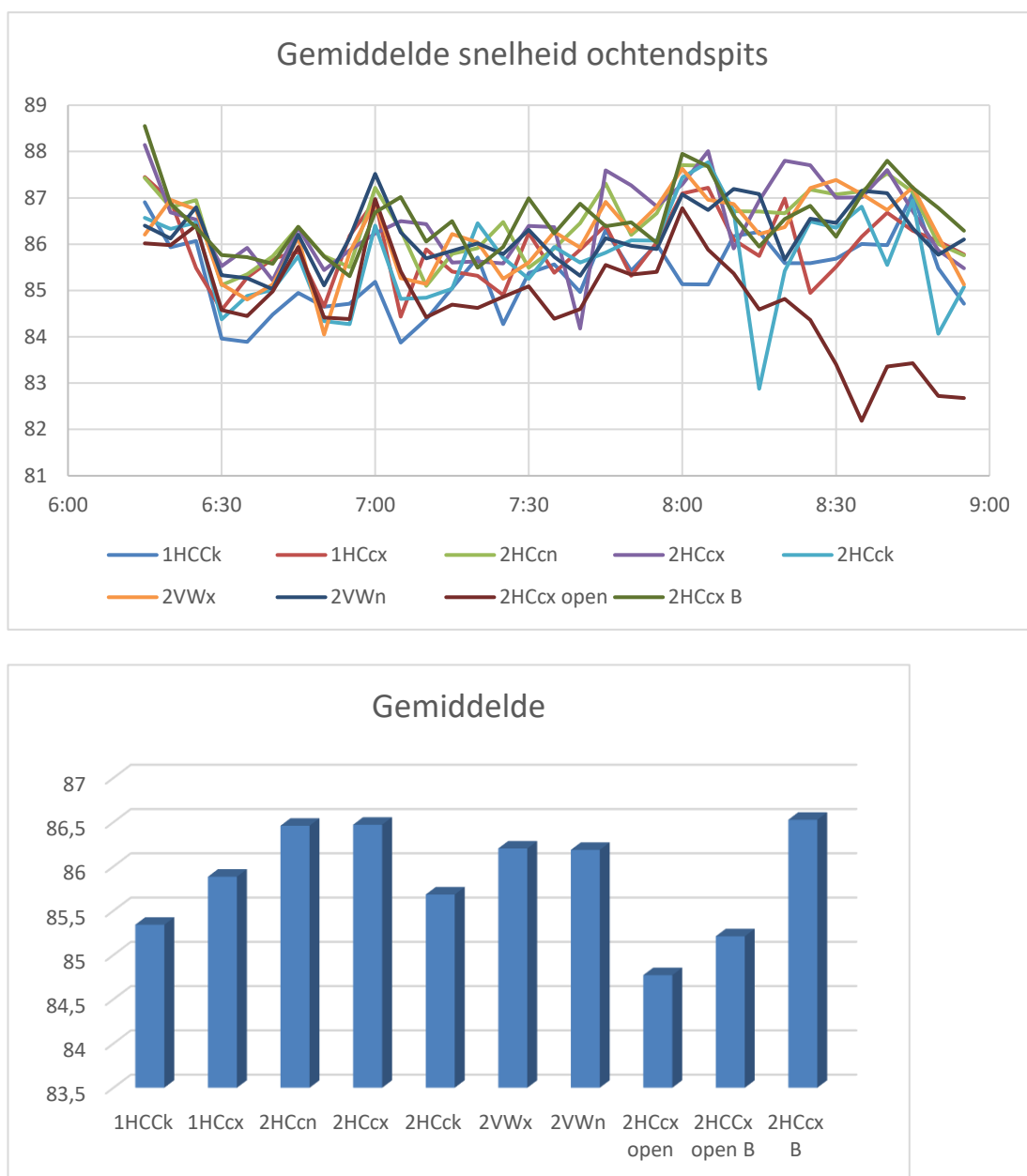
Figuur 44: Gemiddelde snelheid OSP
