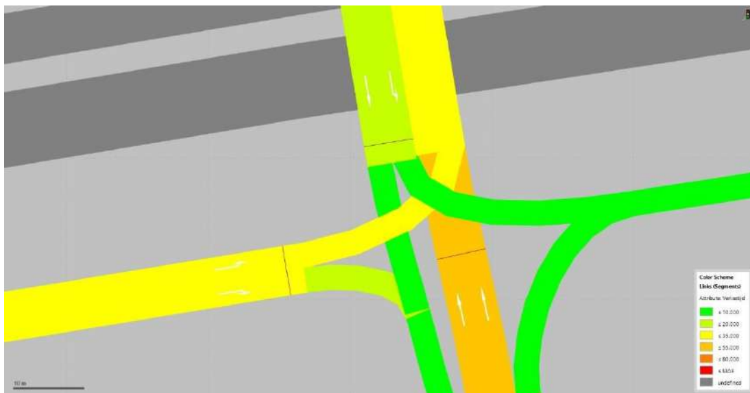
Figuur 100: Verliestijd OSP Waaslandhaven-West Zuid
