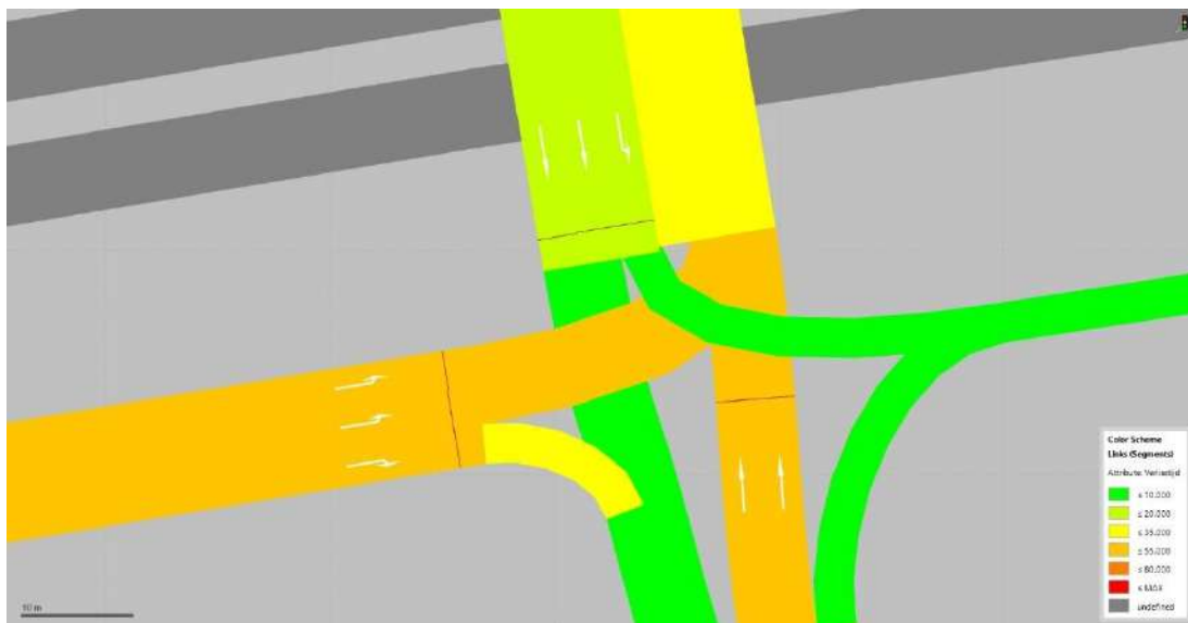
Figuur 55: Verliestijd OSP Waaslandhaven-West Zuid
