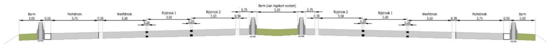
Figuur 3-24: E34 met weefstrook (indicatief profiel; ontwerp voorafname ter onderbouwing van de afbakening van de planologische bestemmingen)
