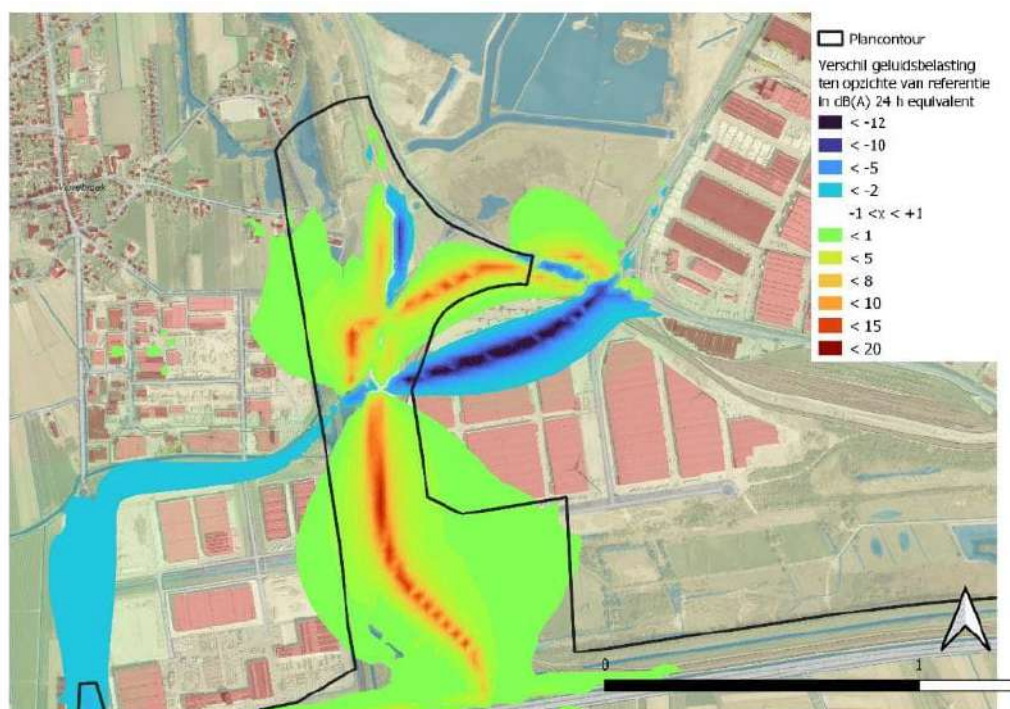
Figuur 6-128 Vershil in geluidsdruk op 1,5 m hoogte voor scenario 2HCc met een ongelijkvloers complex aan Watermolen.
