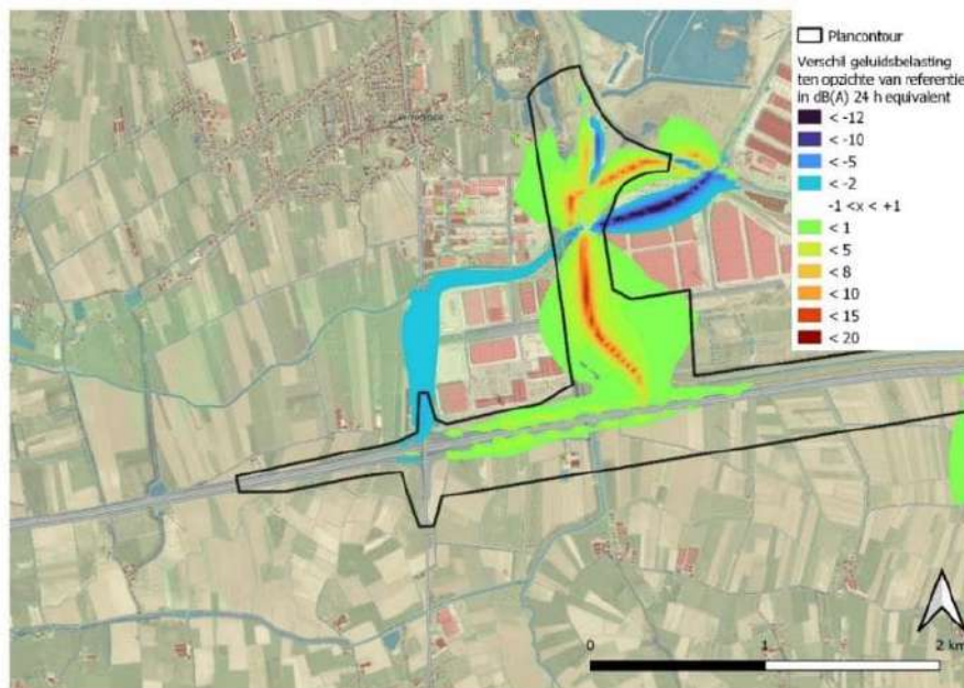
Figuur 6-124 Verskil in geluidsdruk op 1,5 m hoogte voor scenario 2HCc met een ongelijkvloers complex aan Watermolen.
