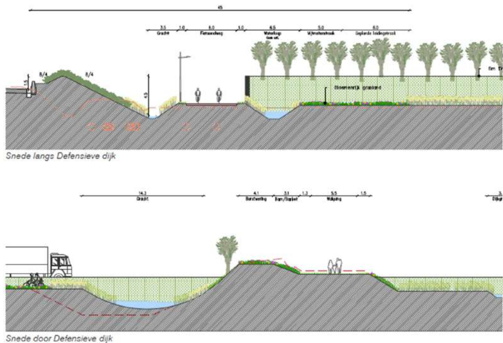
Figuur 3-40: Snedes defensieve dijk (ontwerp voorafname ter onderbouwing van de afbakening van de planologische bestemmingen)
