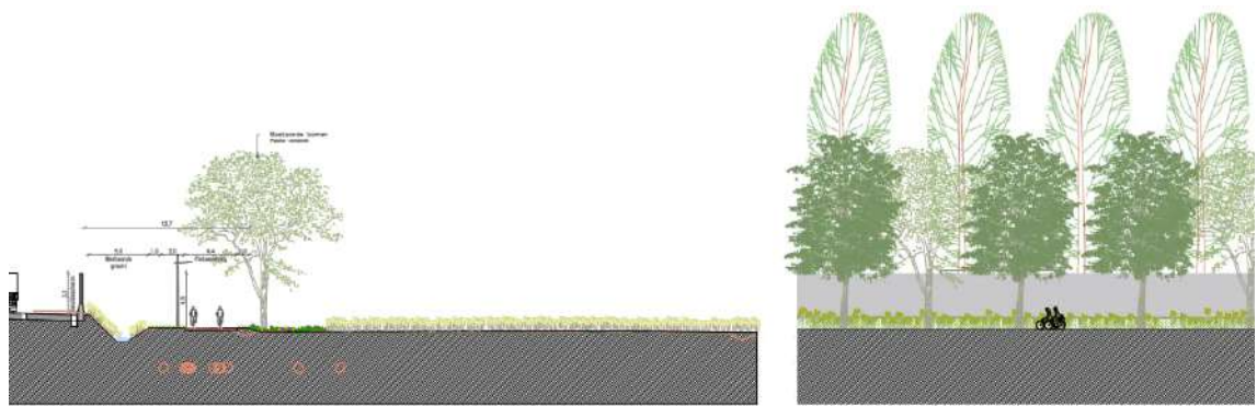
Figuur 3-38: Snede F (ontwerp voorafname ter onderbouwing van de afbakening van de planologische bestemmingen)
