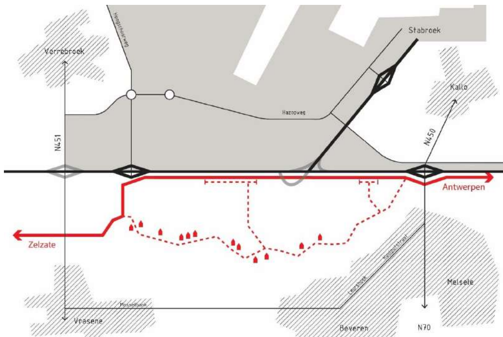
Figuur 3-16: F41 parallel aan de E34
