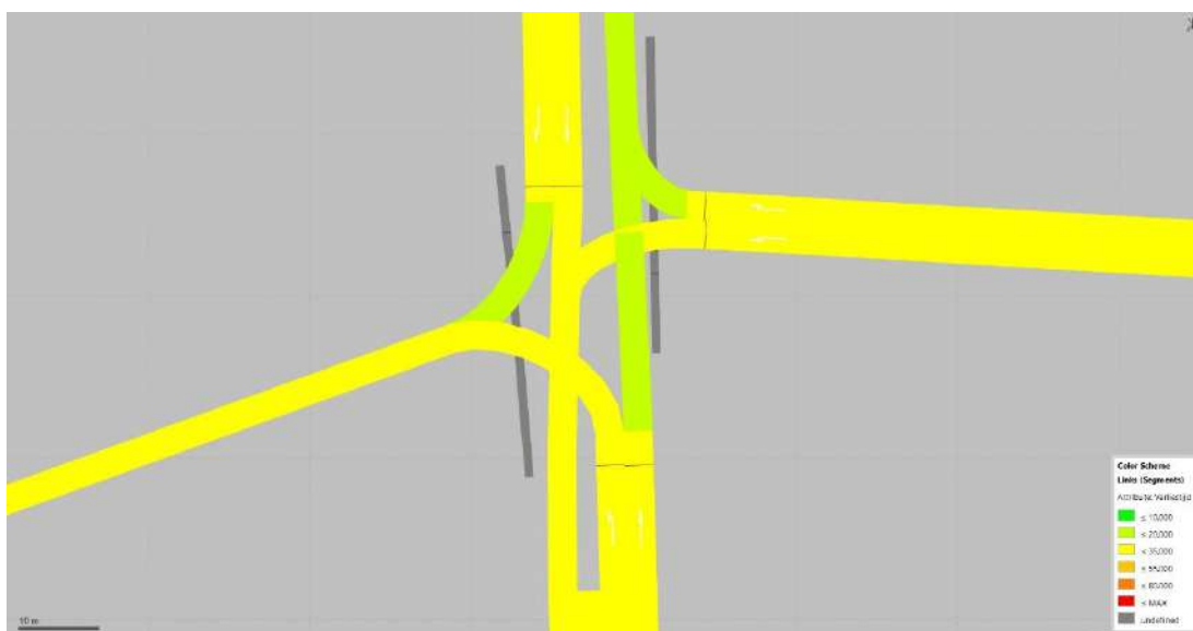
Figuur 153: Verliestijd ASP Vrasene Noord
