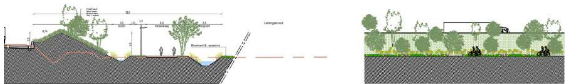
Figuur 3-41: Snede H variant landschapsberm 2,5 m (ontwerp voorafname ter onderbouwing van de afbakening van de planologische bestemmingen)
