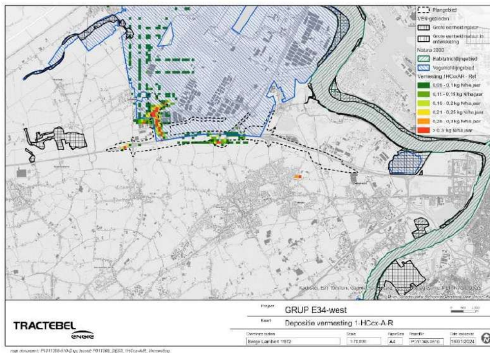
Figuur 6-129 Stikstofdepositietoenames in alternatief 1-HCc-A-R
