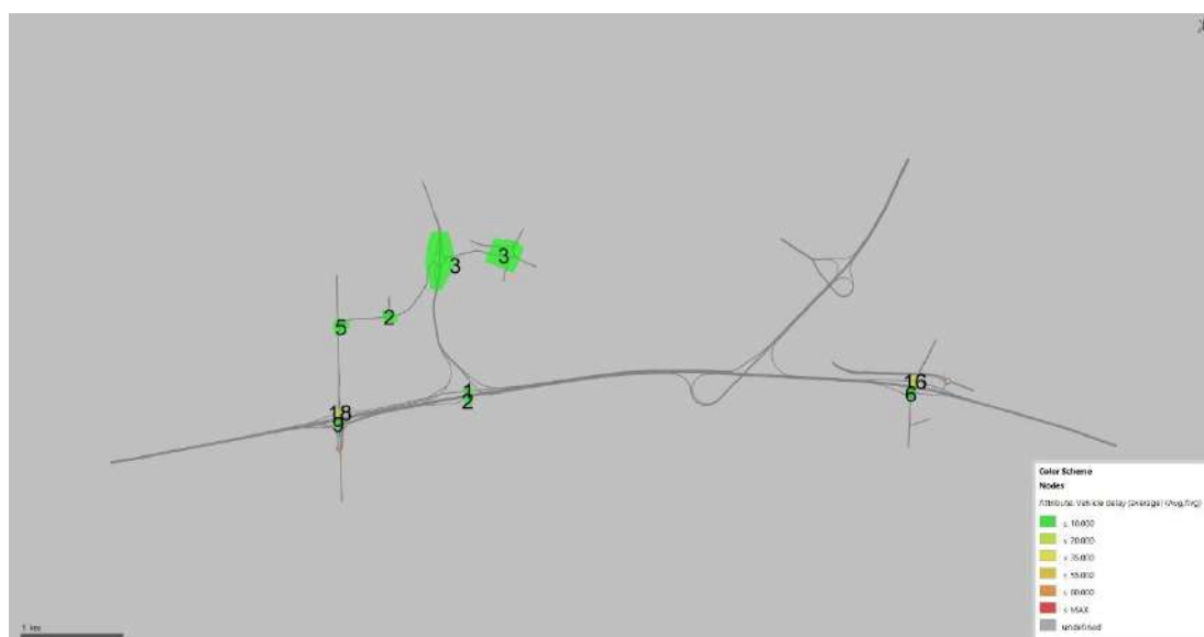
Figuur 208: Verliestijd per kruispunt OSP
