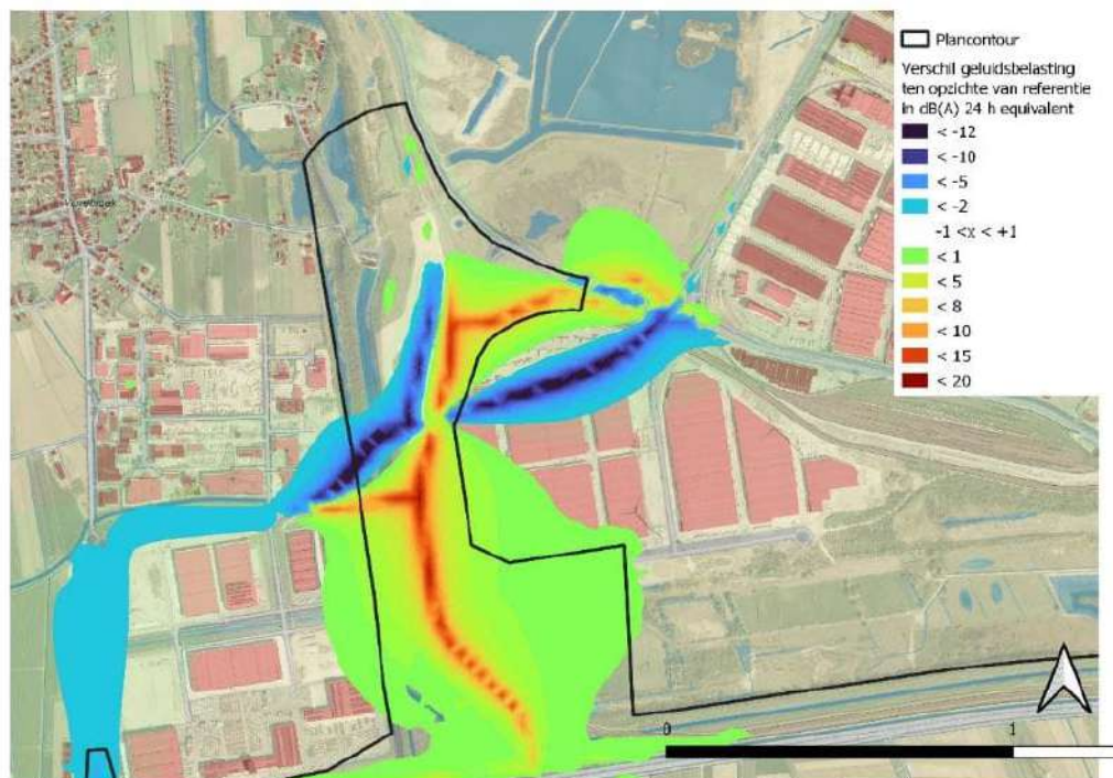
Figuur 6-127 Vershil in geluidsdruk op 1,5 m hoogte voor scenario 2HCc met twee T-kruispunten aan Watermolen.
