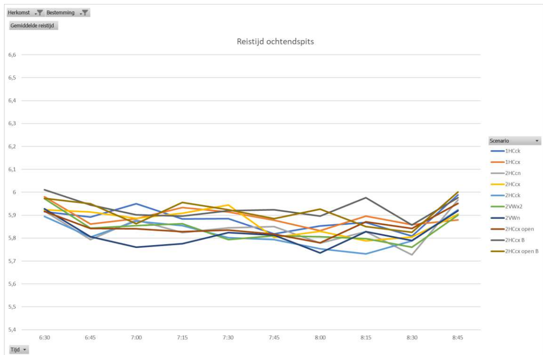
Figuur 38: Reistijden OSP - E34 Zelzate-E34 Antwerpen (X-as: seconden, Y-as: uren en minuten)
