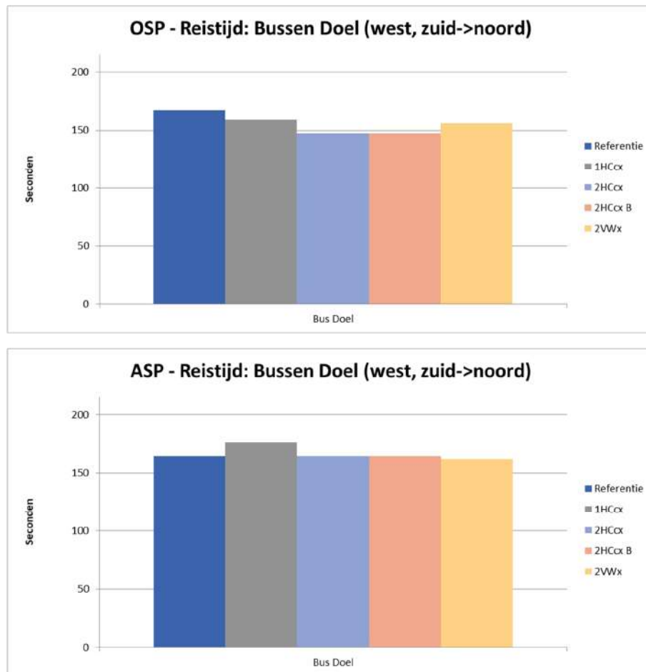
Figuur 6-44: Reistijden bussen Doel West OSP (boven) en ASP (onder)
