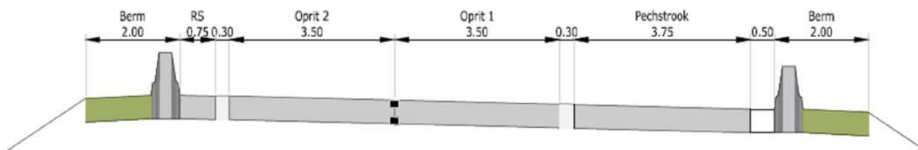
Figuur 3-26: Dubbele oprit (indicatief profiel; ontwerp ter onderbouwing van de afbakening van de planologische bestemmingen)
