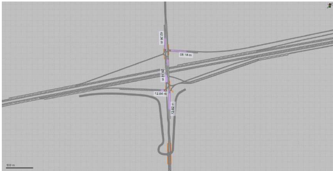
Figuur 186: Gemiddelde maximale wachtrij per 5 minuten OSP Vrasene
