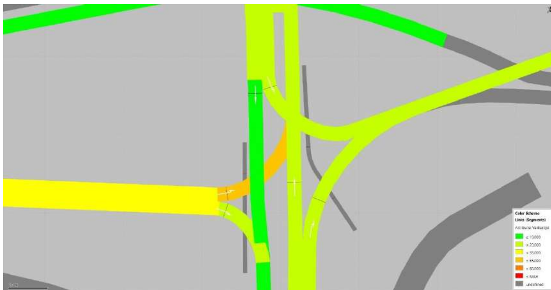
Figuur 154: Verliestijd OSP Vrasene Zuid
