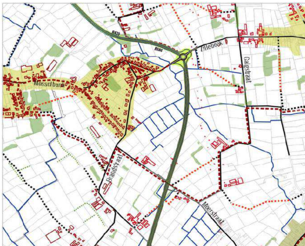
Figuur 8: Scenario 3 - variant 1 - Verhoogde rotonde Zillebeek (bron: deelnota_ontwerpend Onderzoek_tracescenarios_2010_0)
