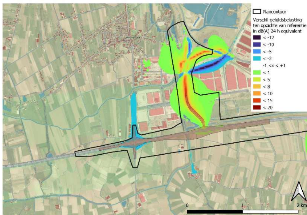
Figuur 5-3 Verschil in geluidsdruk op 1,5 m hoogte voor scenario 1HCc met een rotonde aan Watermolen.
