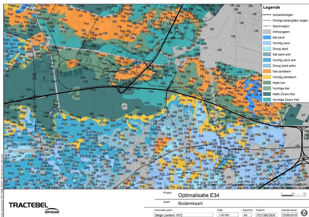
Figuur 3-8: Bodemkaart
