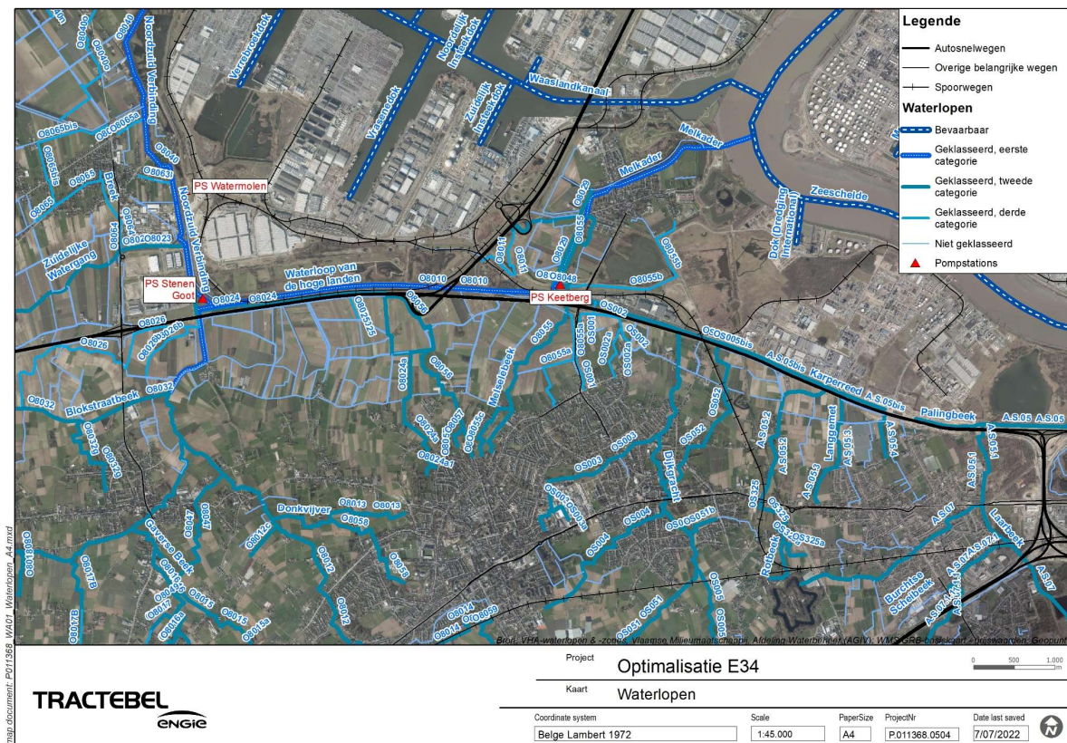
Figuur 3-12: Waterlopen
