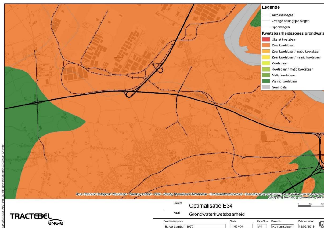
Figuur 3-14: Grondwaterkwetsbaarheidskaart
