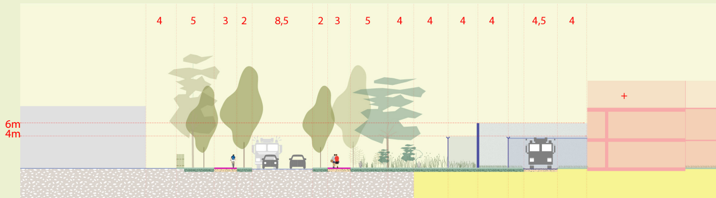
doorsnede BB
