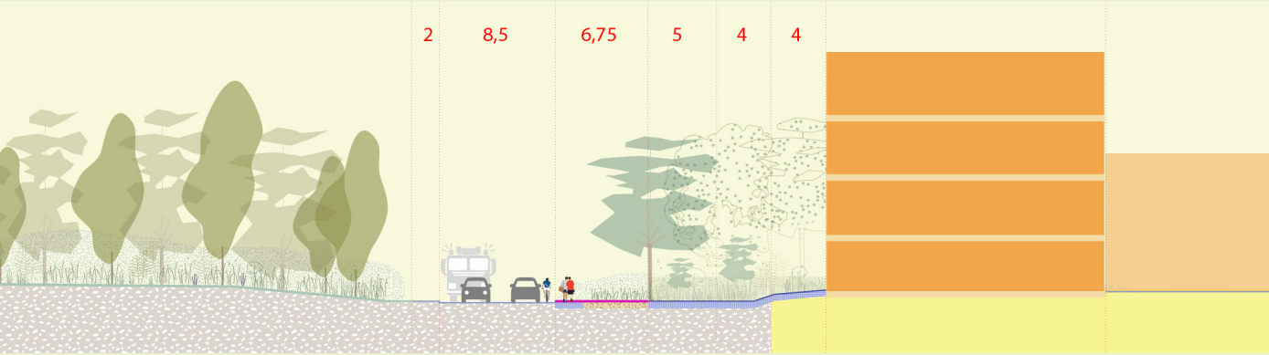
doorsnede AA_2030
