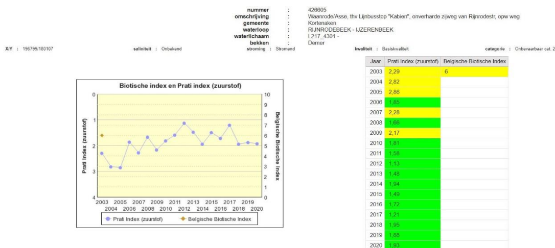
Figuur 3-8: Resultaten Biotische index en Prati index voor de relevante waterlopen in de omgeving van het centrale alternatief (geoloket waterkwaliteit, VMM).
