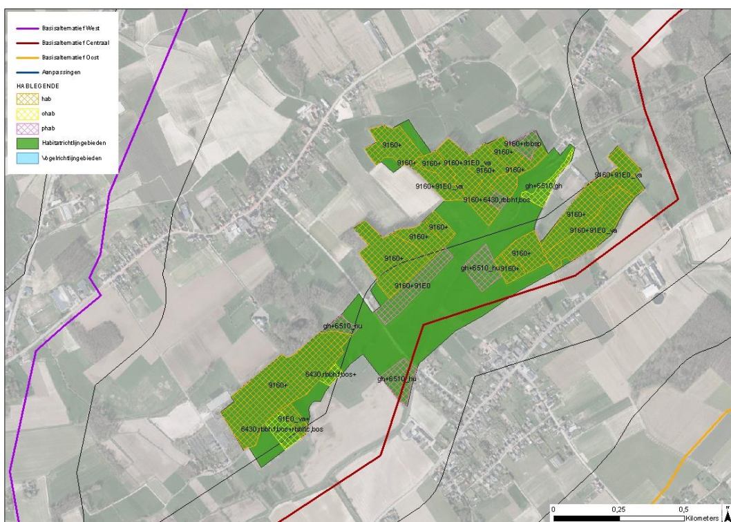
Figuur 4-17: Voorkomende habitats binnen deelgebied 26 Zuurbemde van SBZ-H 'Bos en kalkgraslanden van Haspengouw'.
