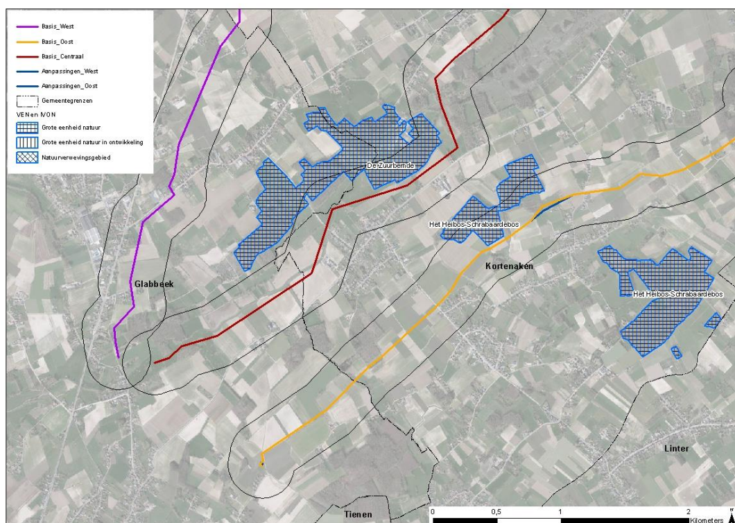
Figuur 4-25: VEN-gebied De Zuurbemde bij alternatief centraal en Het Heibos-Schrabaardebos bij alternatief oost.
