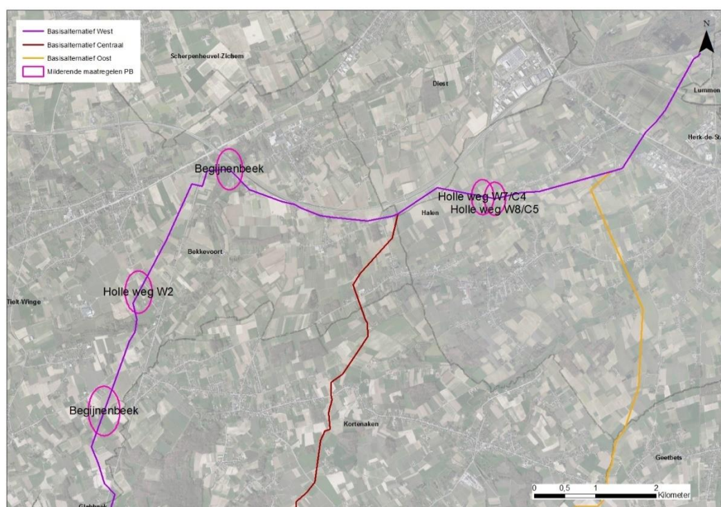
Figuur 4-24: Waardevolle kleine landschapselementen voor vleermuizen.
