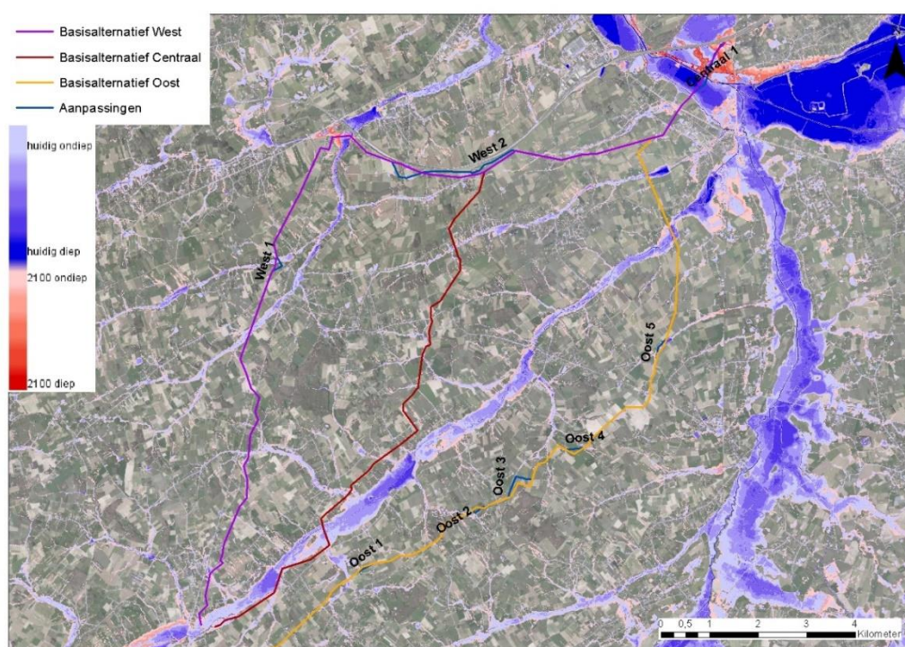
Figuur 3-5: Aangroeikaart overstroombaar gebied (scenario hoog impact 2100)
