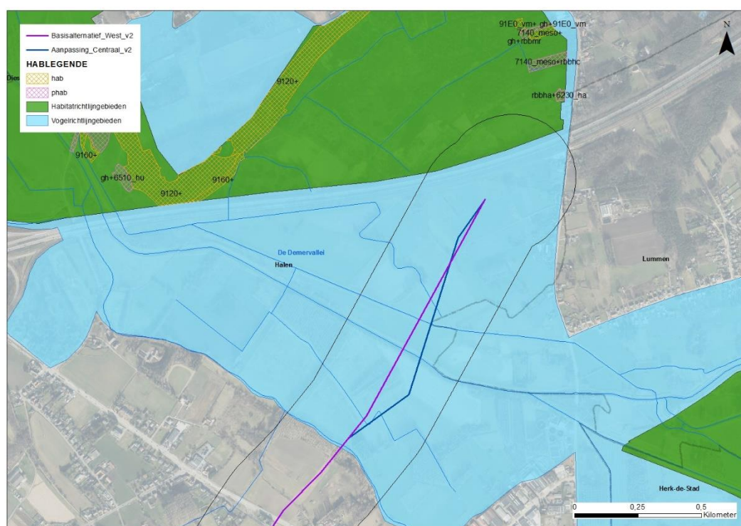
Figuur 4-21: Voorkomende habitats binnen het SBZ-H Demervallei.
