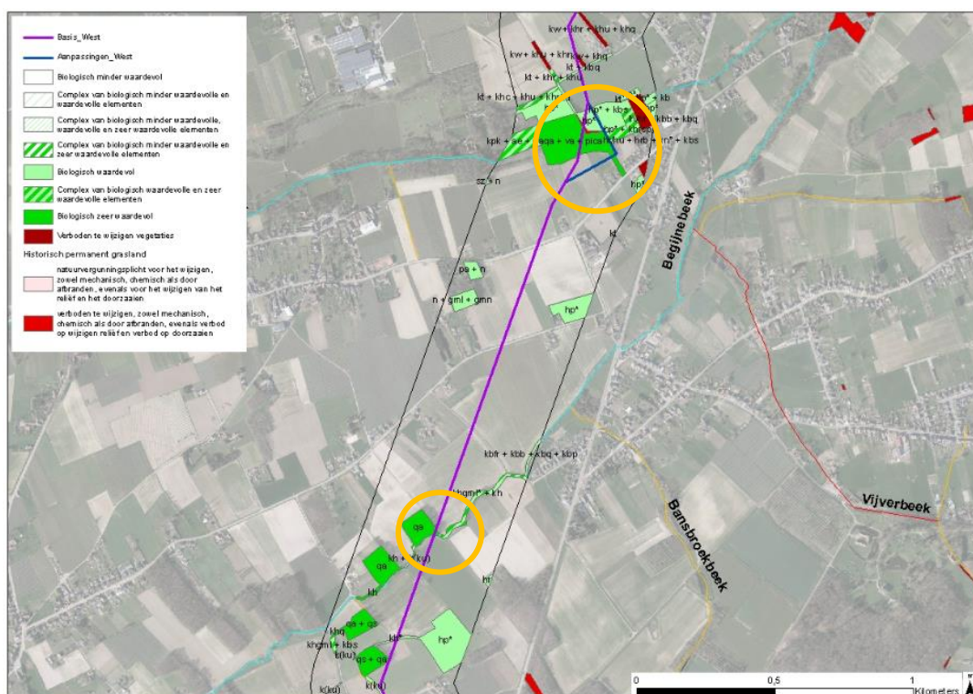
Figuur 4-5: Analyse Biotoopverlies Alternatief West (middenzone).
