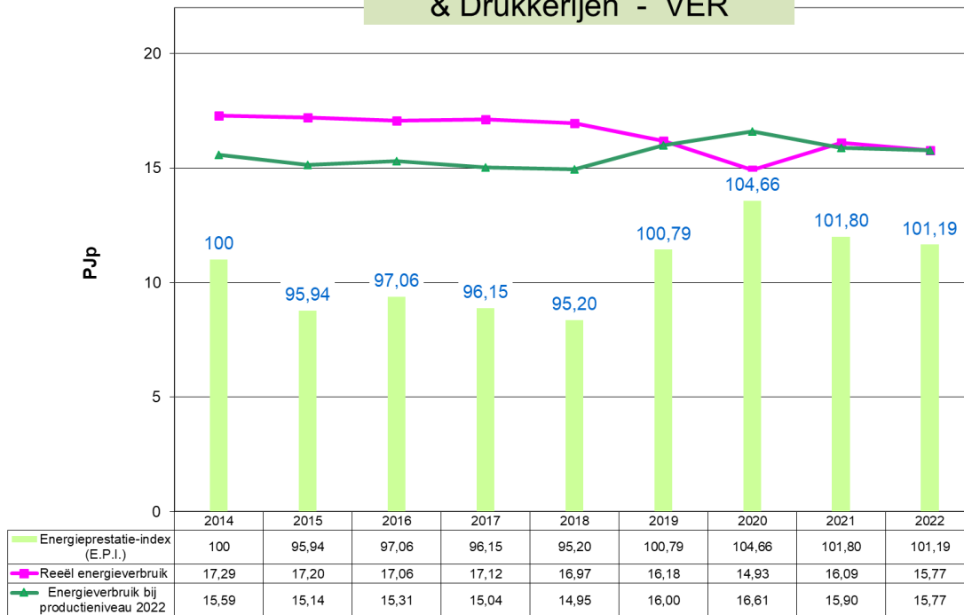
Grafiek 34: Evolutie 2014 – 2022 van het energieverbruik en de E.P.I. voor Papier, Papier- en kartonverwerking & Drukkerijen (VER-bedrijven)
