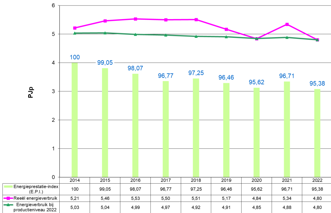
Grafiek 44: Evolutie 2014 – 2022 van het energieverbruik en de E.P.I. voor Textiel & Hout (niet VER-bedrijven)
