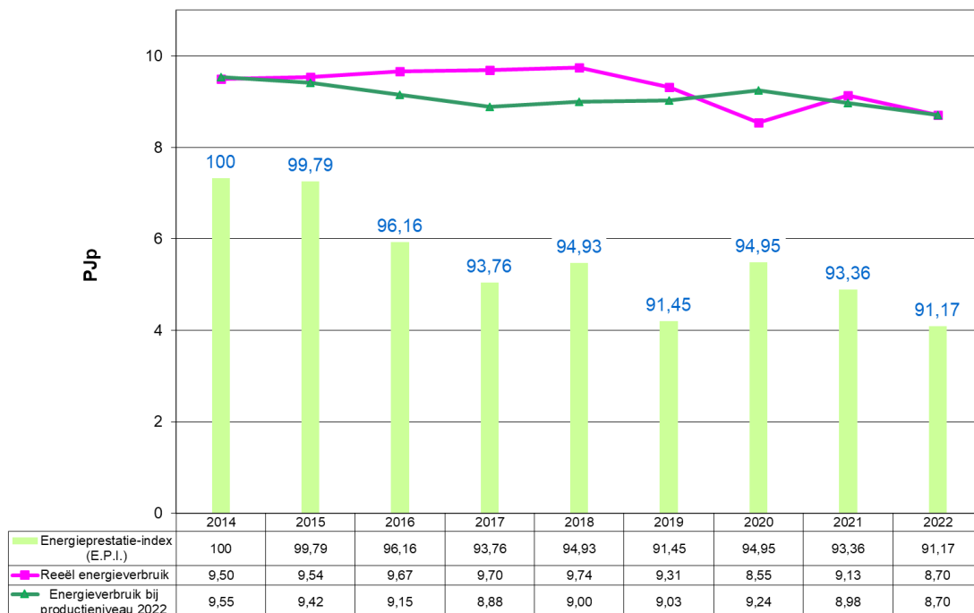
Grafiek 41: Evolutie 2014 – 2022 van het energieverbruik en de E.P.I. voor Non-ferro & Metaalverwerking (niet VER-bedrijven)
