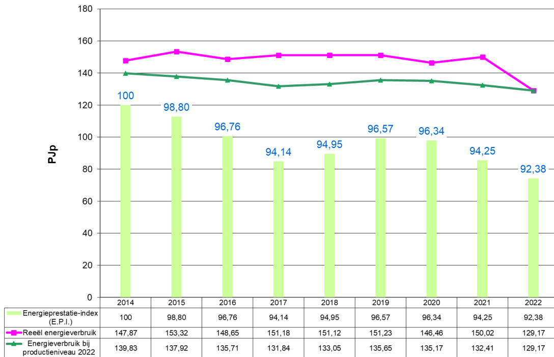
Grafiek 30: Evolutie 2014 – 2022 van het energieverbruik en de E.P.I. voor Chemie & Kunststoffen (VER-bedrijven)
