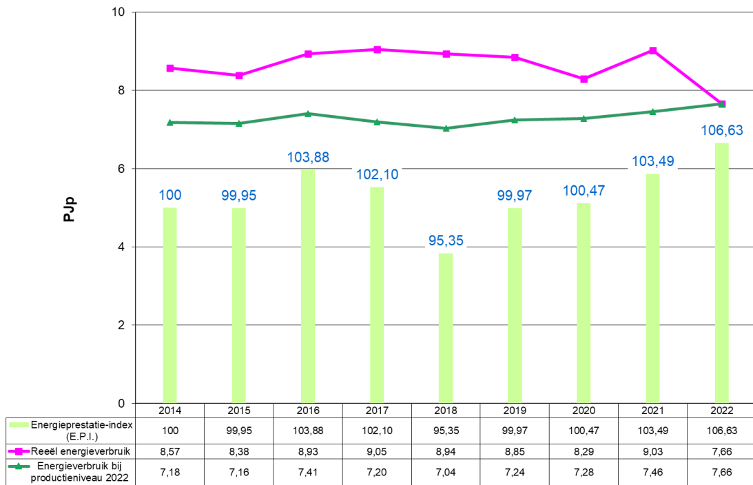
Grafiek 43: Evolutie 2014 – 2022 van het energieverbruik en de E.P.I. voor Textiel & Hout (VER-bedrijven)
