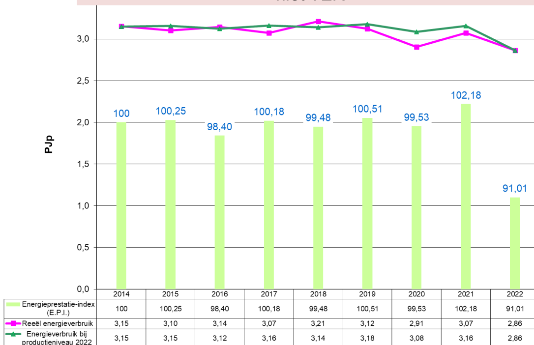
Grafiek 47: Evolutie 2014 – 2022 van het energieverbruik en de E.P.I. voor Keramische sector, Minerale niet-metaalproducten & Glas (niet VER-bedrijven)
