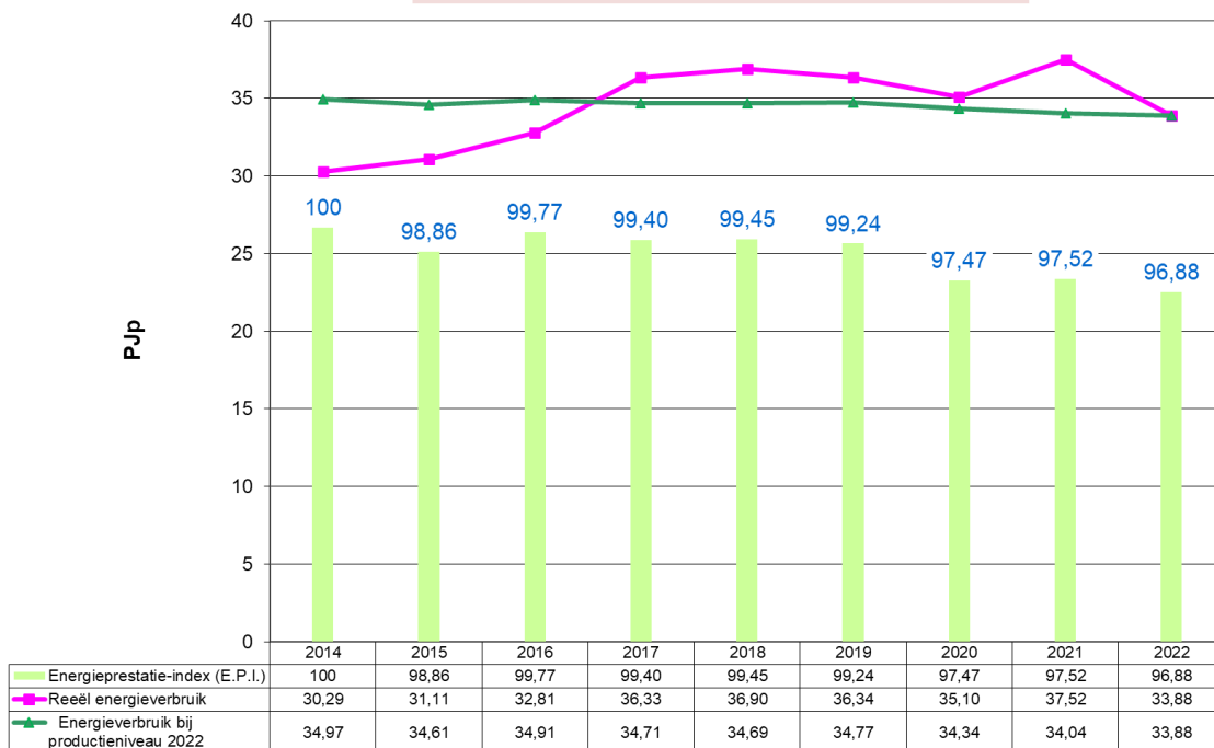
Grafiek 31: Evolutie 2014 – 2022 van het energieverbruik en de E.P.I. voor Chemie & Kunststoffen (niet VER-bedrijven)
