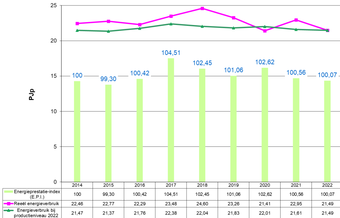
Grafiek 40: Evolutie 2014 – 2022 van het energieverbruik en de E.P.I. voor Non-ferro & Metaalverwerking (VER-bedrijven)
