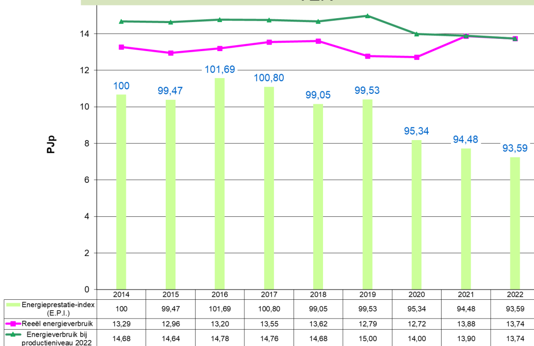
Grafiek 46: Evolutie 2014 – 2022 van het energieverbruik en de E.P.I. voor Keramische sector, Minerale niet-metaalproducten & Glas (VER-bedrijven)
