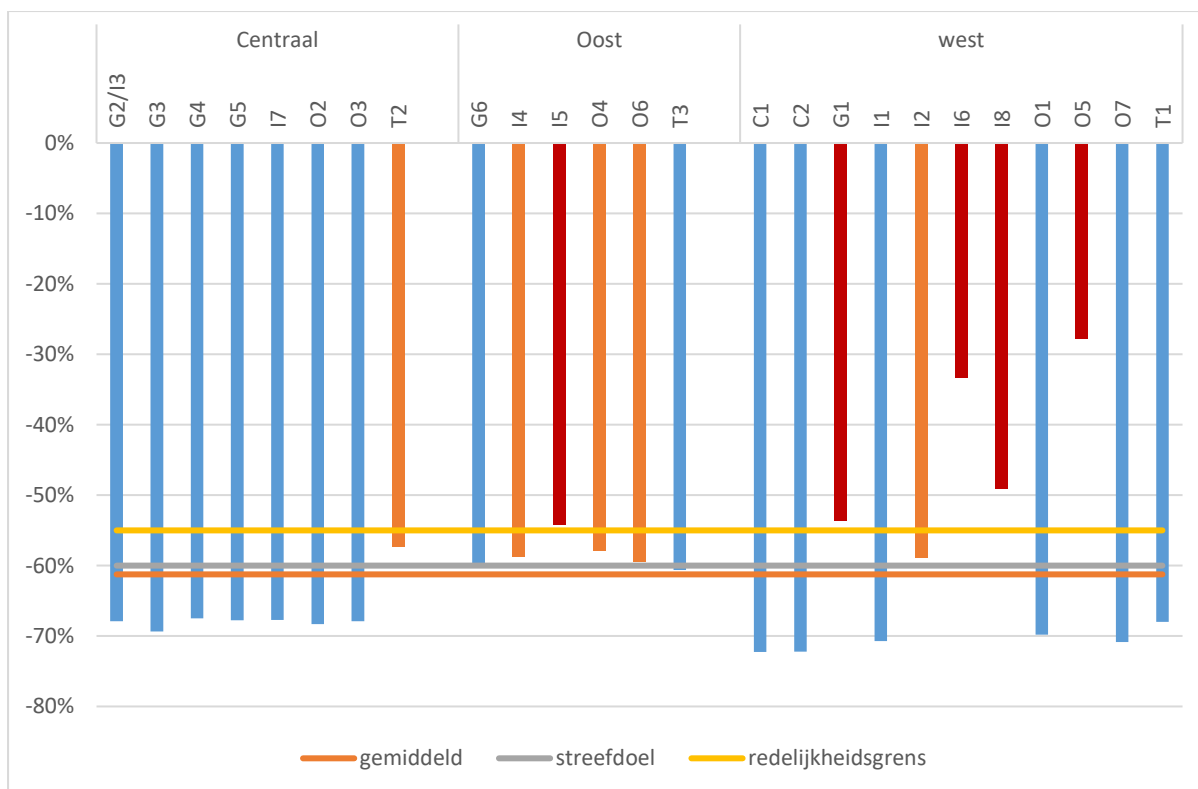
Figuur 5-4 | overzicht evolutie vrachtkilometers in woongebied per alternatief (blauw: voldoet aan het streefdoel, oranje: voldoet niet aan het streefdoel, maar valt binnen de redelijkheidsgrenzen, rood: voldoet niet aan de redelijkheidsgrenzen)
