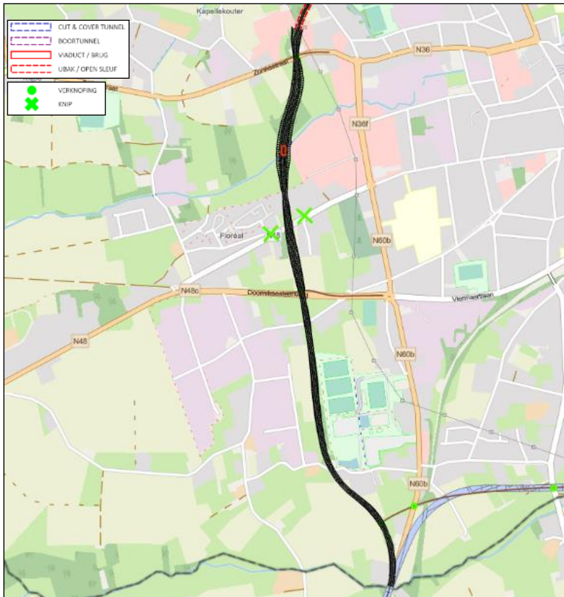
Figuur 5-16 | conceptuutwerking vak 3 van inspraakalternatief G2/I3
