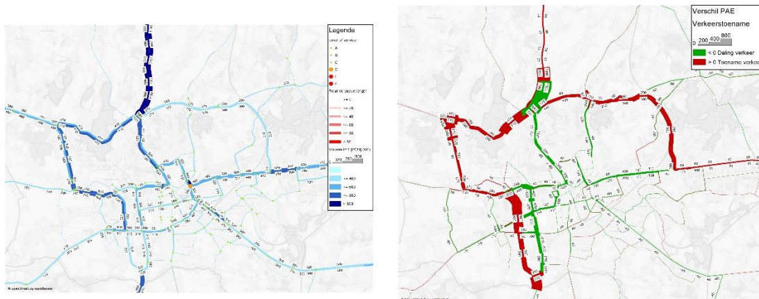
Figuur 5-71 | Verkeersintensiteiten (links) en verschillenplot (rechts) voor alternatief I8
