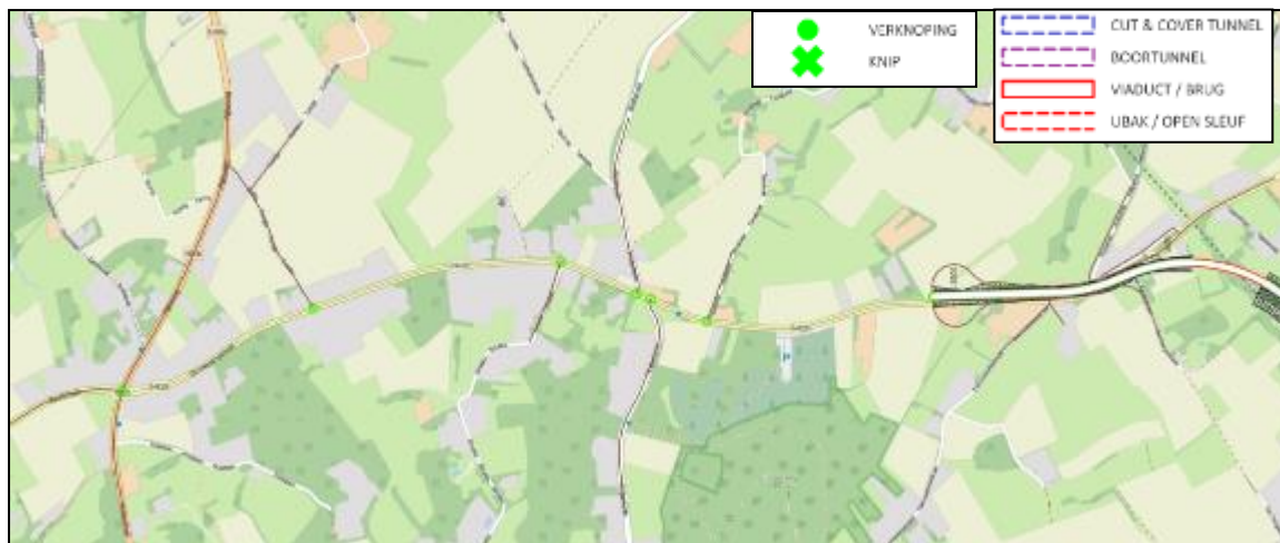
Figuur 5-143 | conceptuutwerking vak 1 van deelalternatief N2
