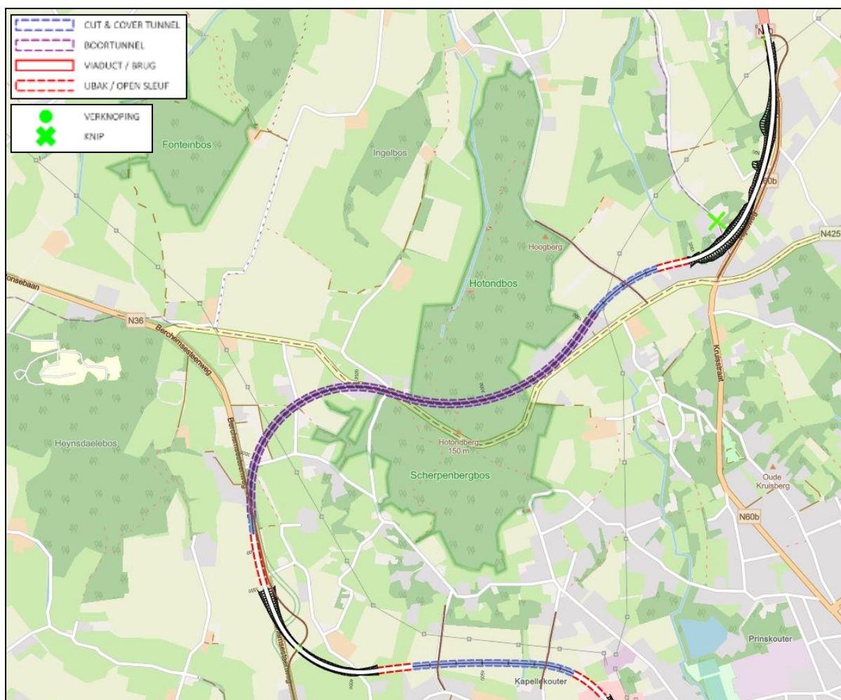
Figuur 5-125 | Conceptuutwerking vak 1 van alternatief C1
