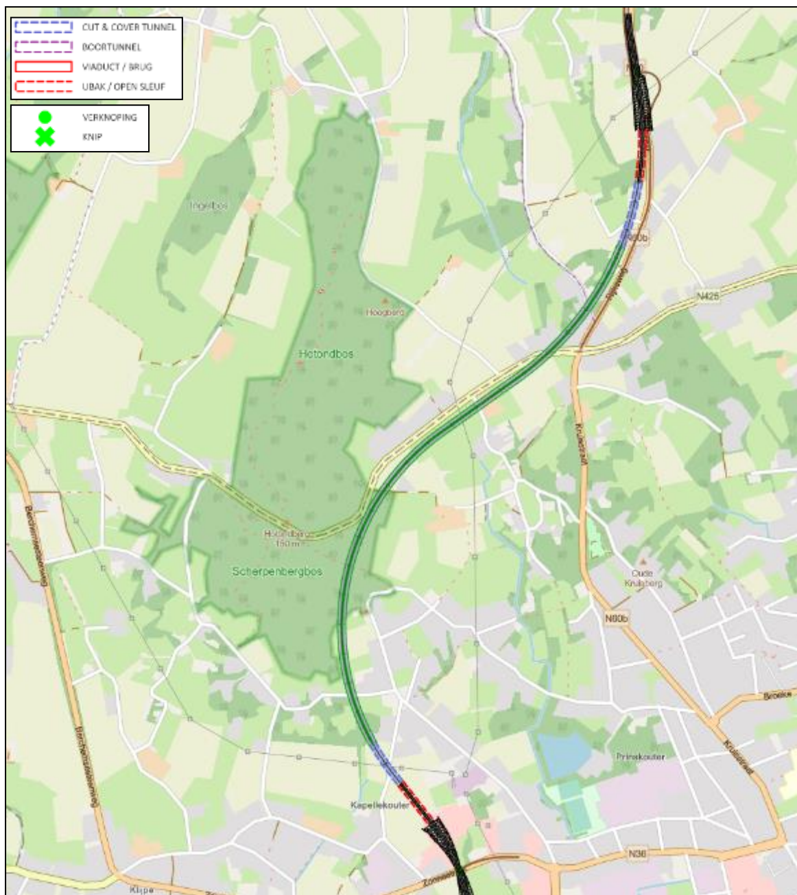
Figuur 5-84 | conceptuitwerking vak 1 van alternatief O2
