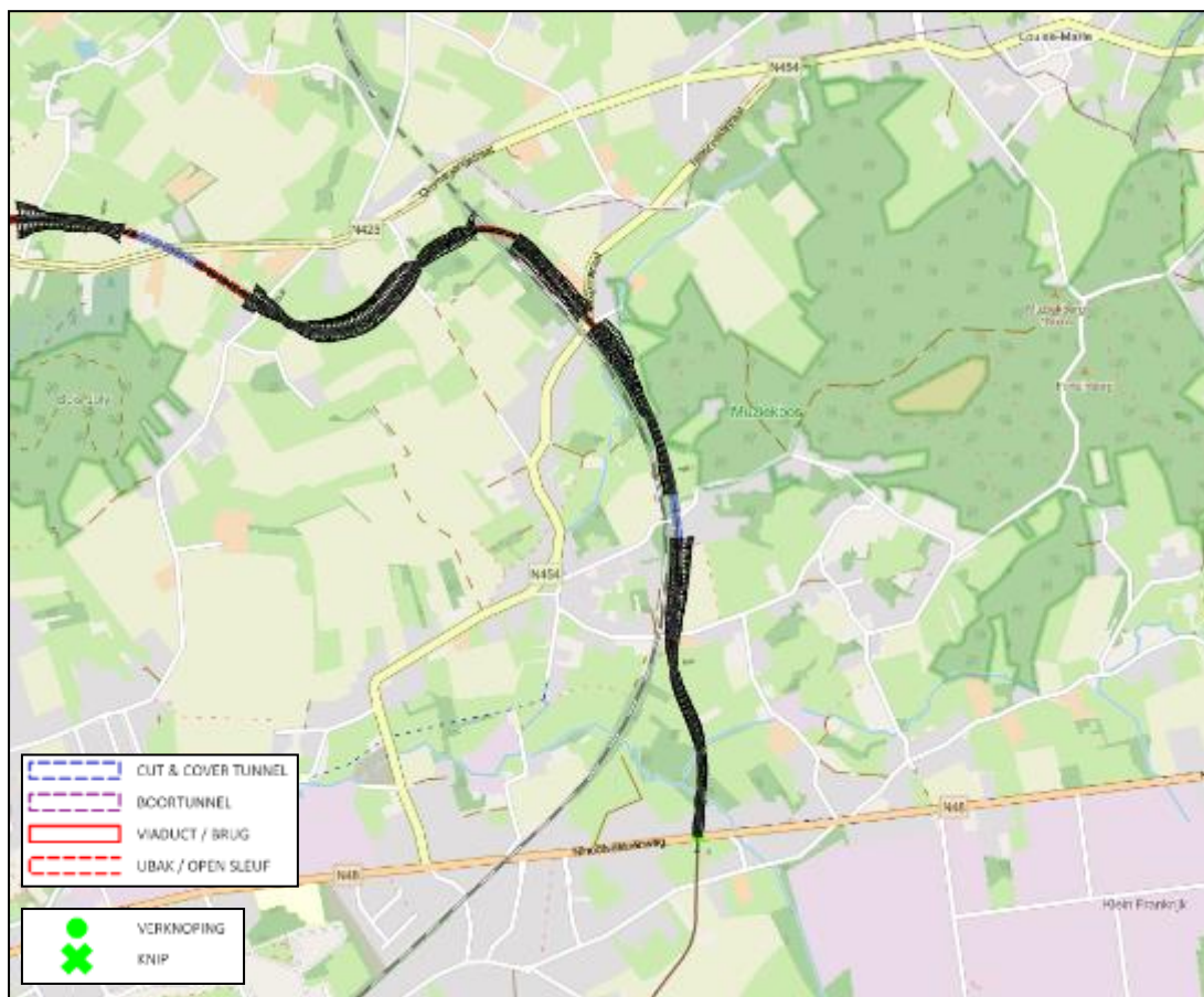
Figuur 5-96 | conceptuitwerking vak 2 van alternatief O4
