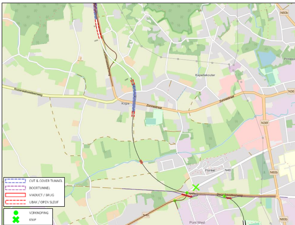
Figuur 5-131 | conceptuitwerking vak 2 van alternatief C2
