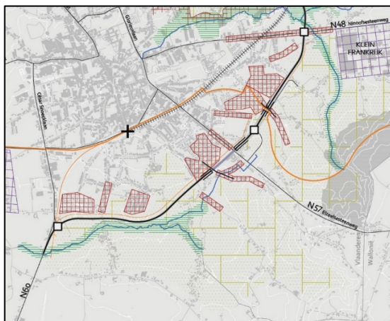
Figuur 4.39 | doorvertaling ontwerpalternatief Z1
