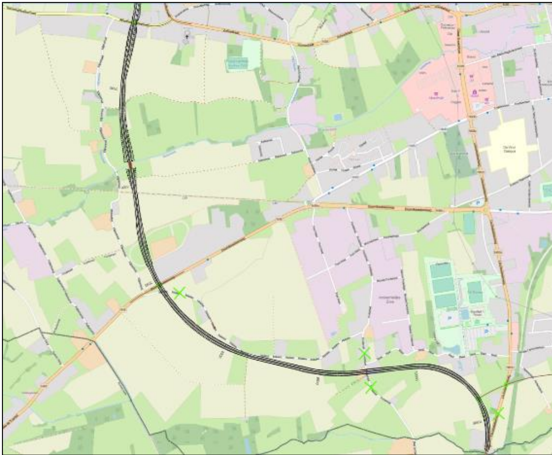
Figuur 5-43 | conceptuitwerking vak 3 van inspraakalternatief I1
