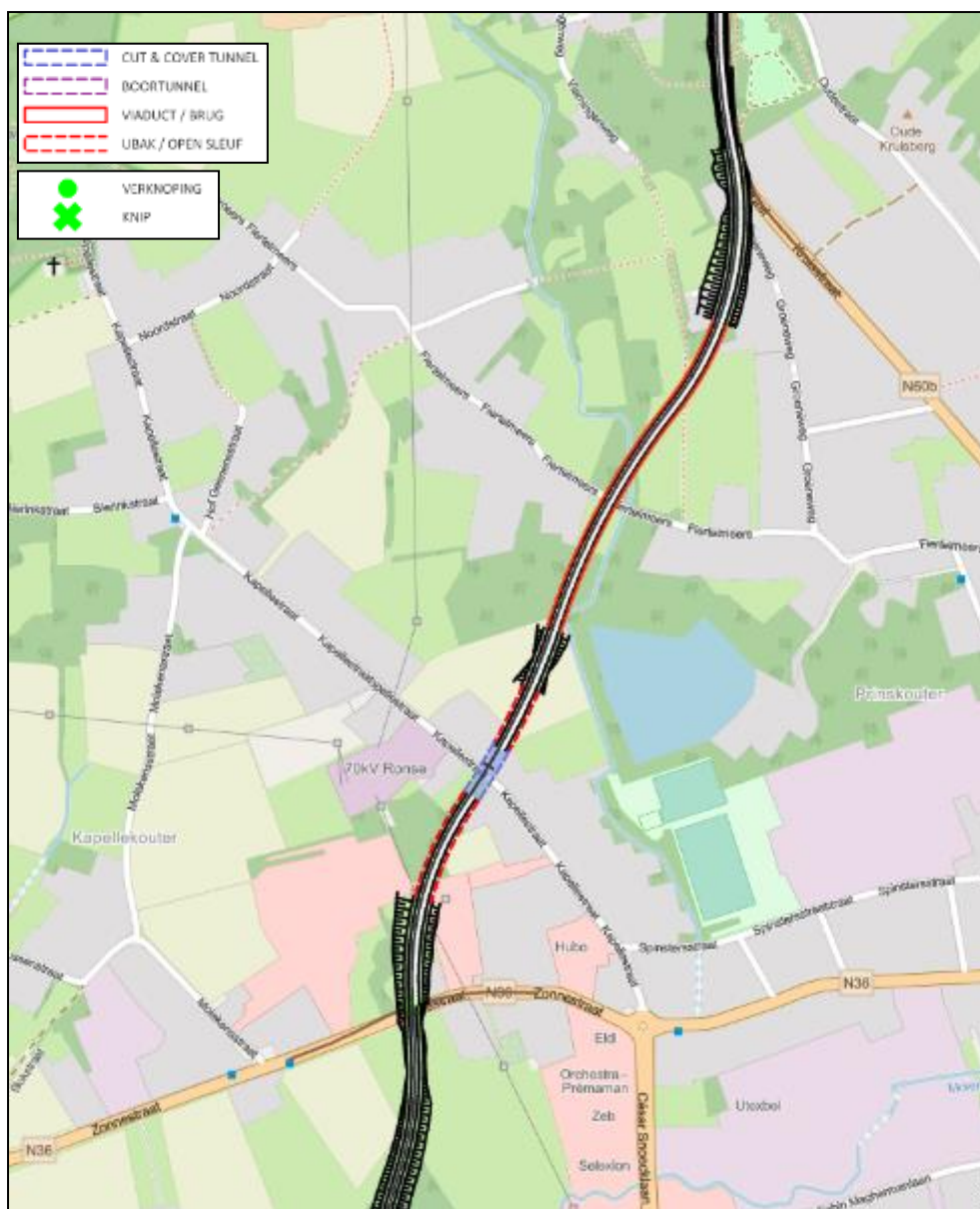
Figuur 5-21 | conceptuitwerking vak 2 van alternatief G3
