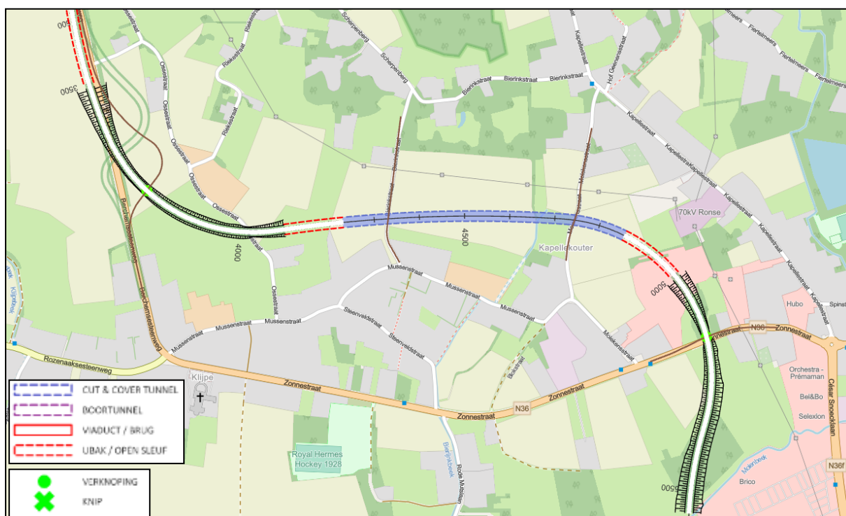
Figuur 5-126 | conceptuitwerking vak 2 van alternatief C1
