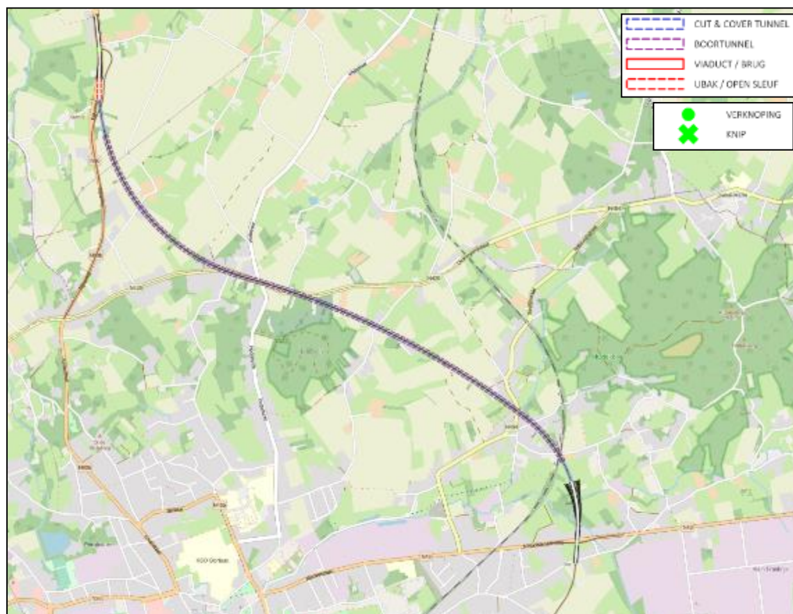
Figuur 5-122 | conceptuutwerking vak 1 van oostelijk tunnelalternatief T3
