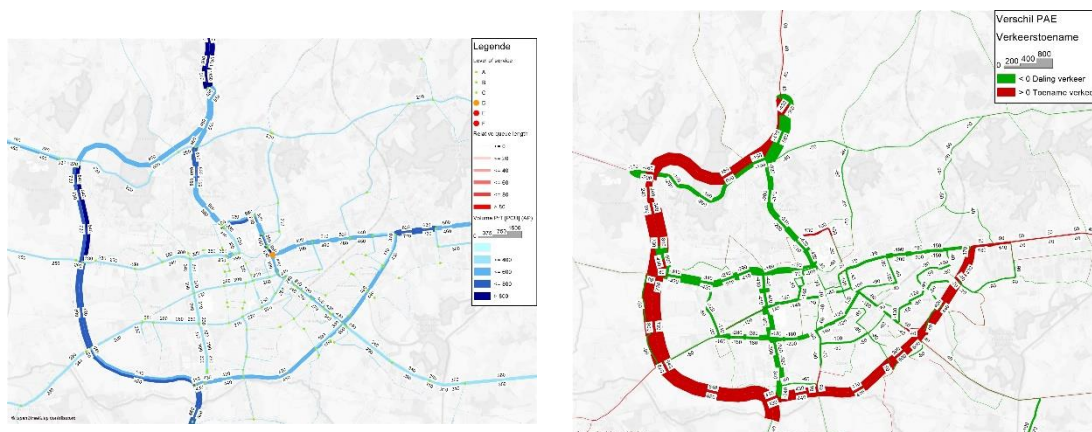
Figuur 5-78: Verkeersintensiteiten (links) en verschillenplot (rechts) voor alternatief O1
