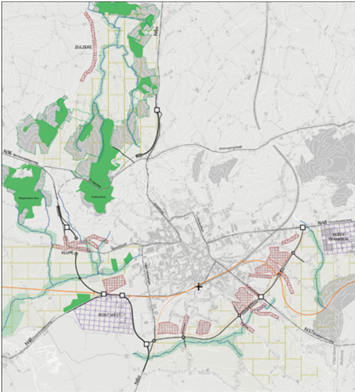
Figuur 4.37 | Voorstelling combinatiealternatief C2
