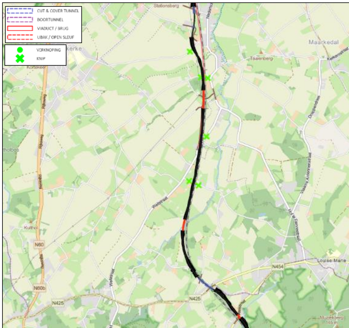
Figuur 5-52 | conceptuïtwerking vak 1 (2e deel) van inspraakalternatief I4
