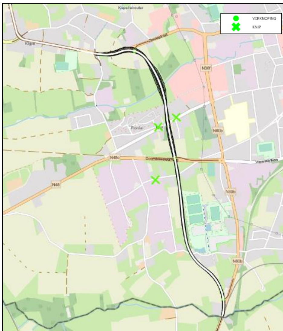
Figuur 5-74 | conceptuitwerking vak 3 van inspraakalternatief I8
