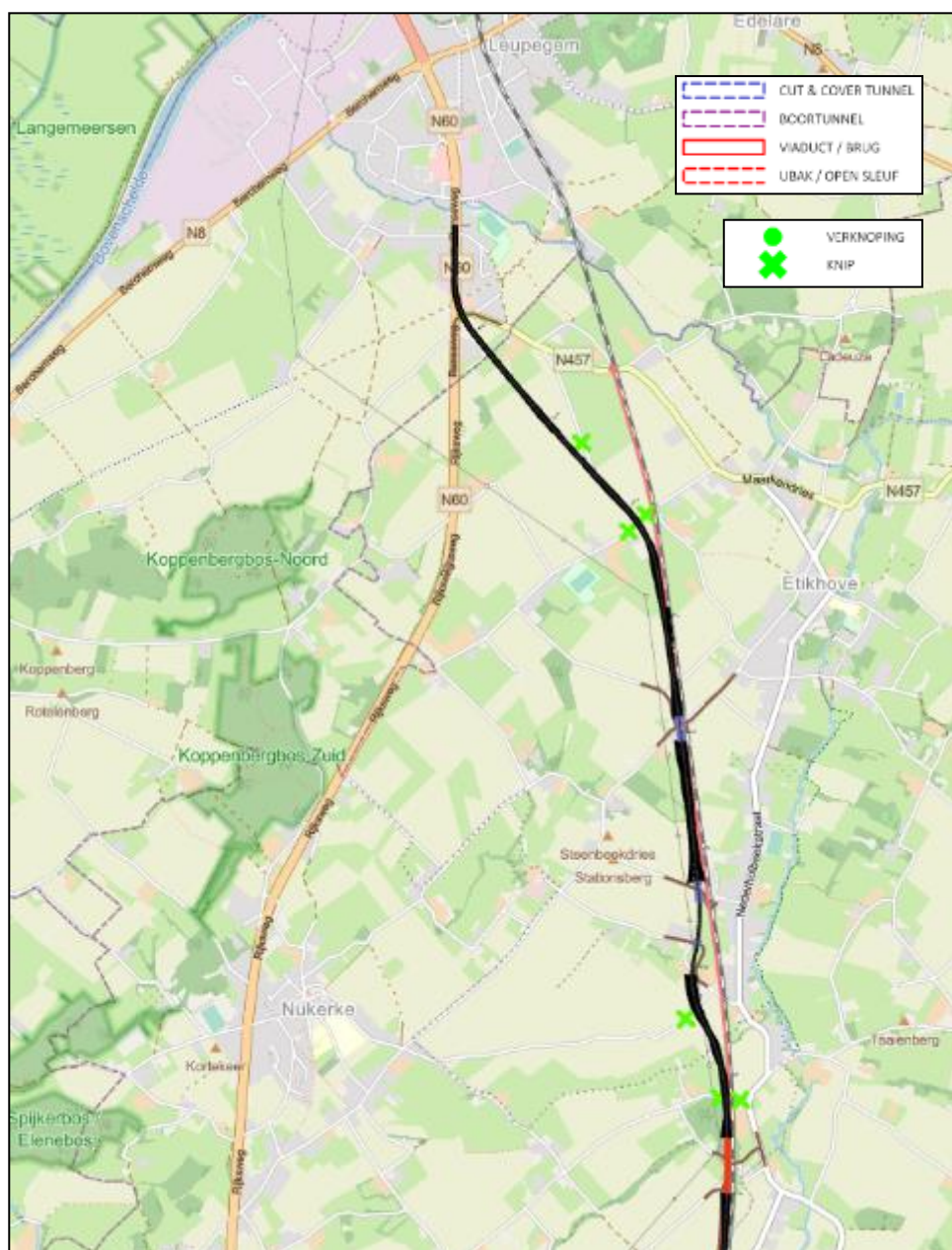
Figuur 5-51 | conceptuitwerking vak 1 (1e deel) van inspraakalternatief I4.
