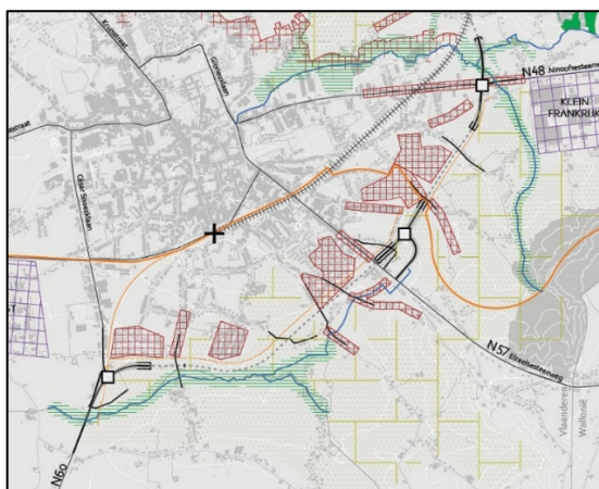
Figuur 4.41 | doorvertaling ontwerpalternatief Z3
