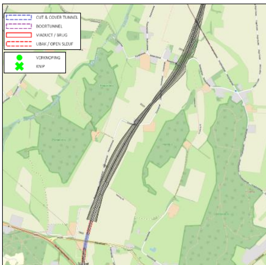
Figuur 5-41 | conceptuitwerking vak 1 (3e deel) van inspraakalternatief I1
