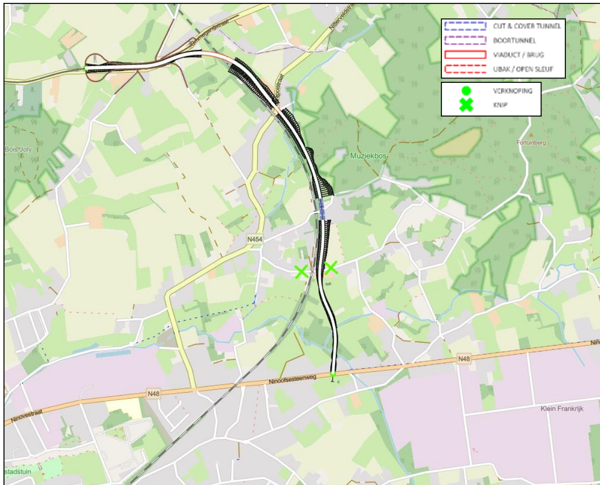
Figuur 5-76 | conceptuitwerking vak 5 van inspraakalternatief I8
