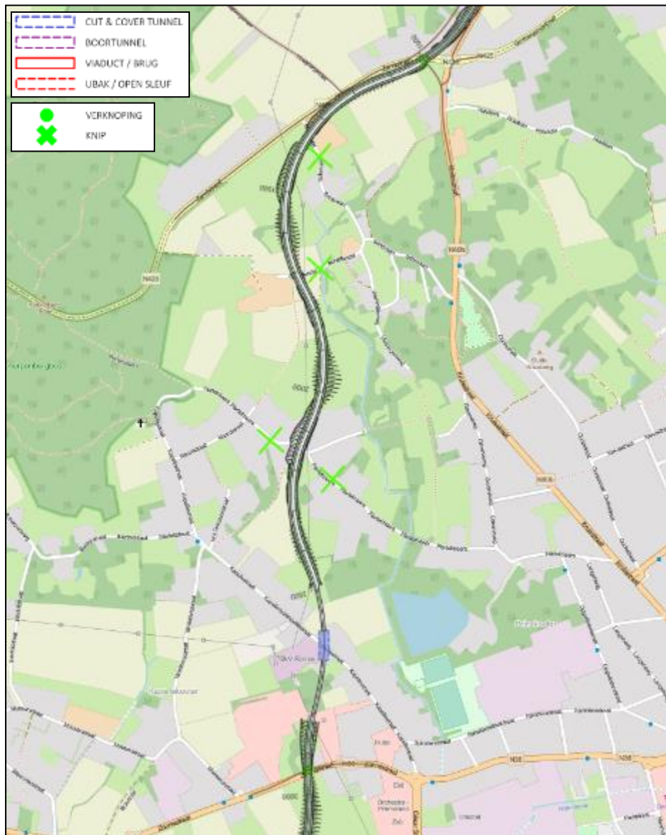
Figuur 5-67 | conceptuitwerking vak 2 van inspraakalternatief I7
