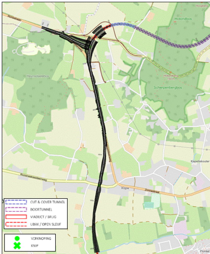
Figuur 5-80 | conceptuutwerking vak 2 van alternatief O1
