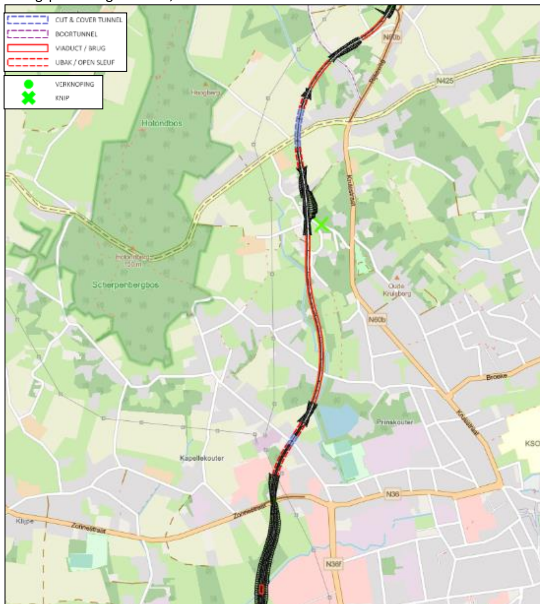
Figuur 5-15 | conceptuitwerking vak 2 van inspraakalternatief G2/I3
