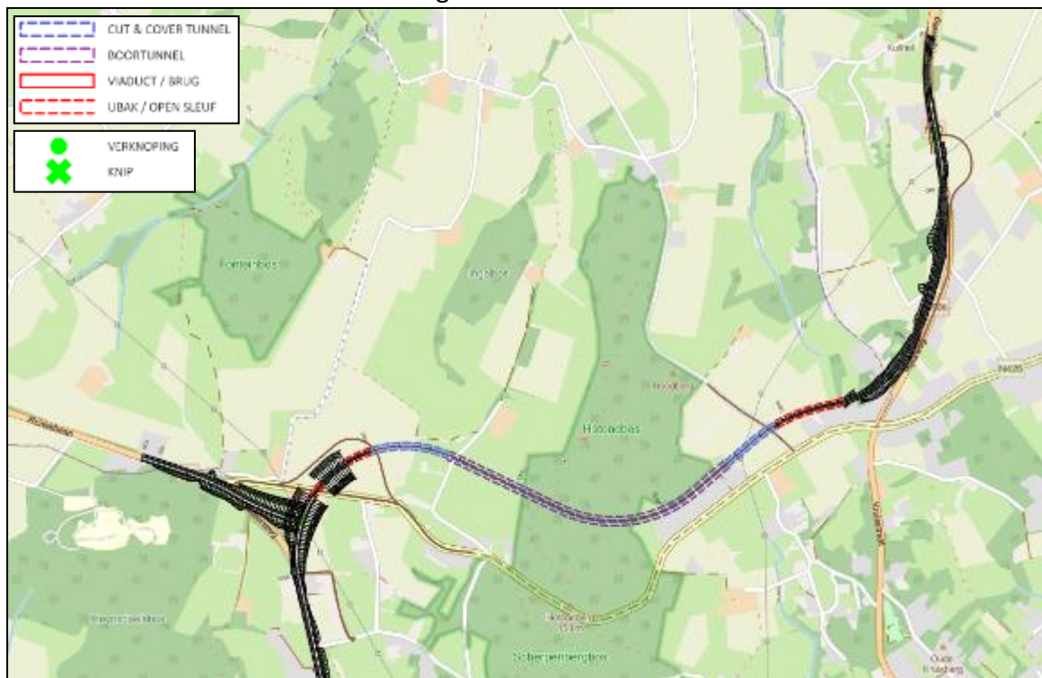
Figuur 5-79 | conceptuutwerking vak 1 van alternatief O1
