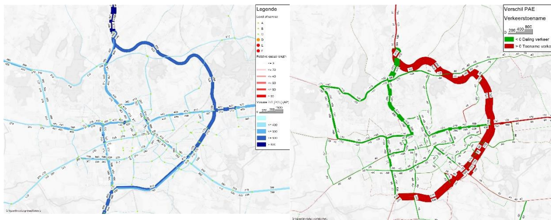
Figuur 5-103 | Verkeersintensiteiten (links) en verschillenplot (rechts) voor alternatief O6
