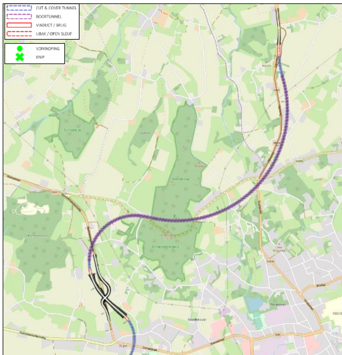
Figuur 5-113 | conceptuitwerking vak 1 van tunnelalternatief T1
