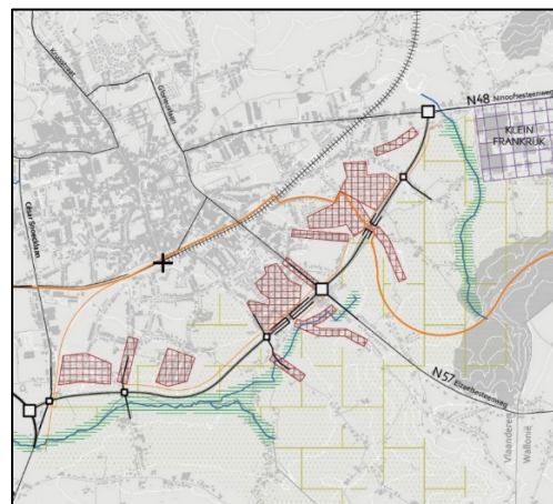
Figuur 4.40 | doorvertaling ontwerpalternatief Z2
