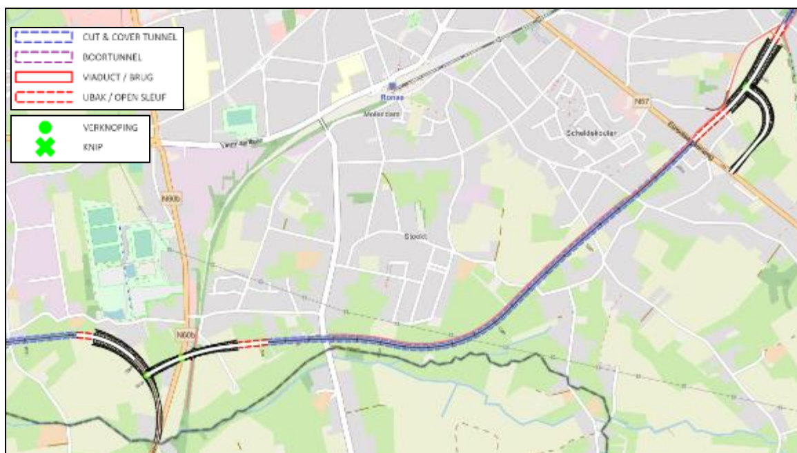
Figuur 5-140 | conceptuutwerking vak 1 van alternatief Z4
