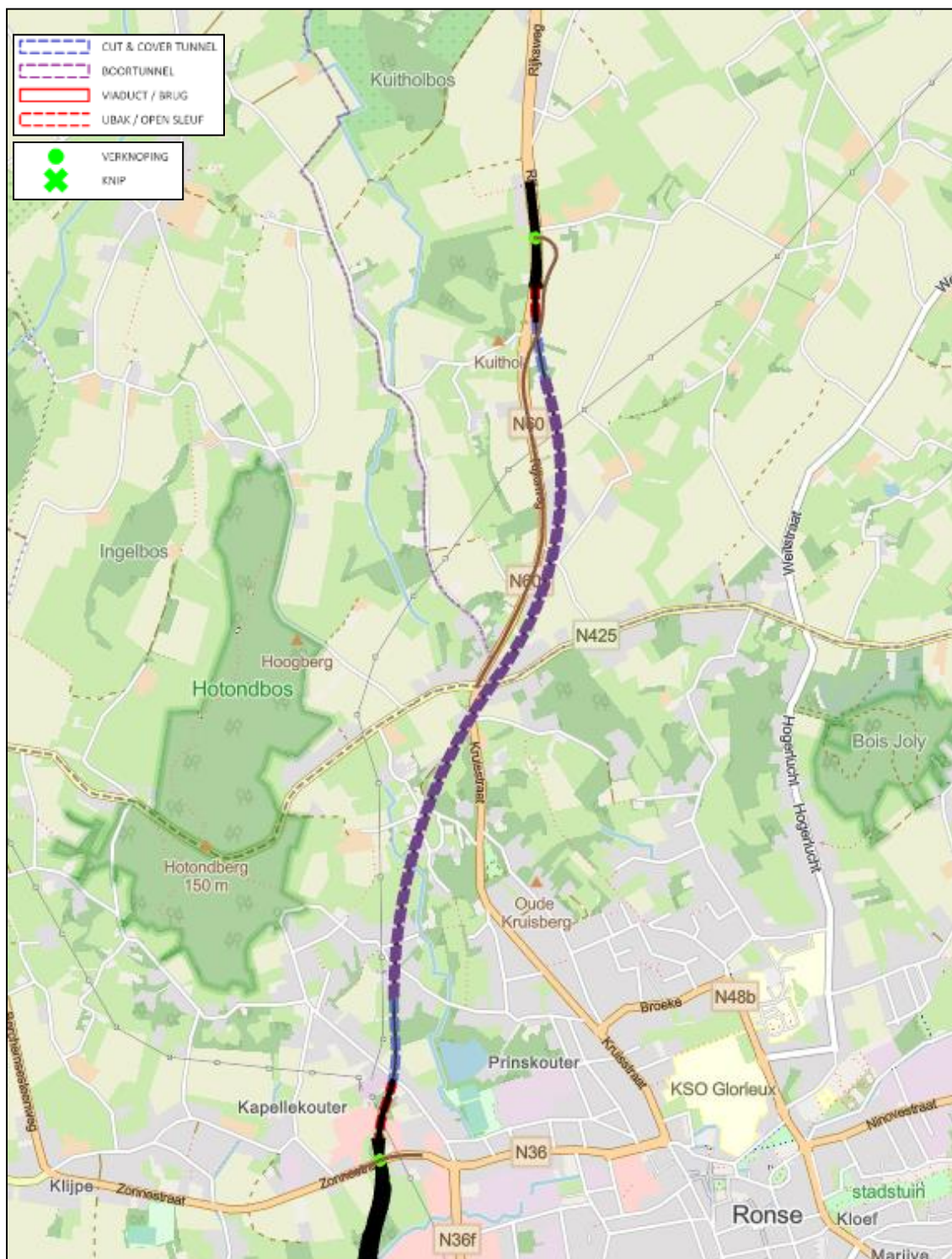
Figuur 5-25 | conceptuitwerking vak 1 van alternatief G4
