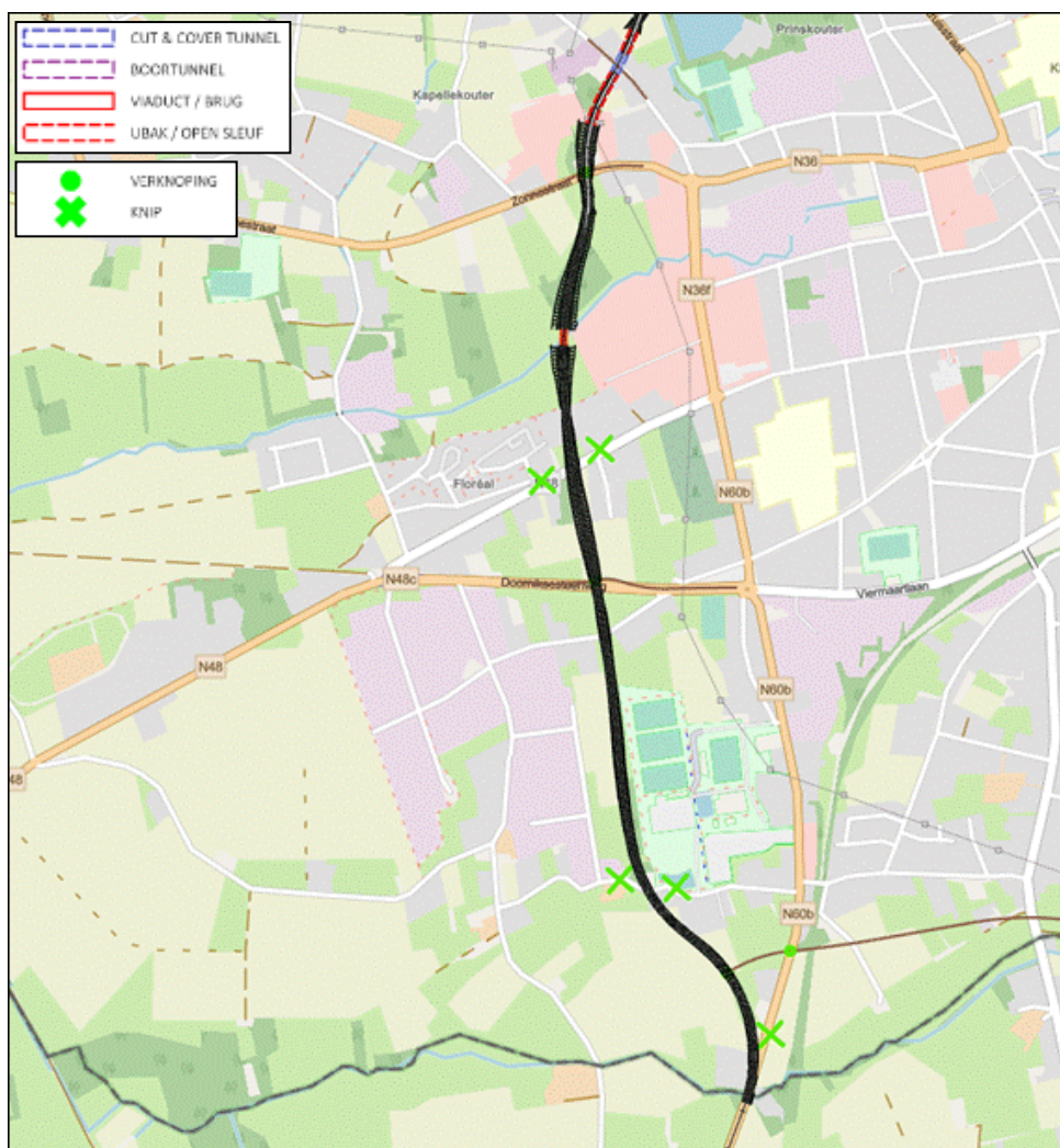
Figuur 5-92 | conceptuitwerking vak 3 van alternatief O3
