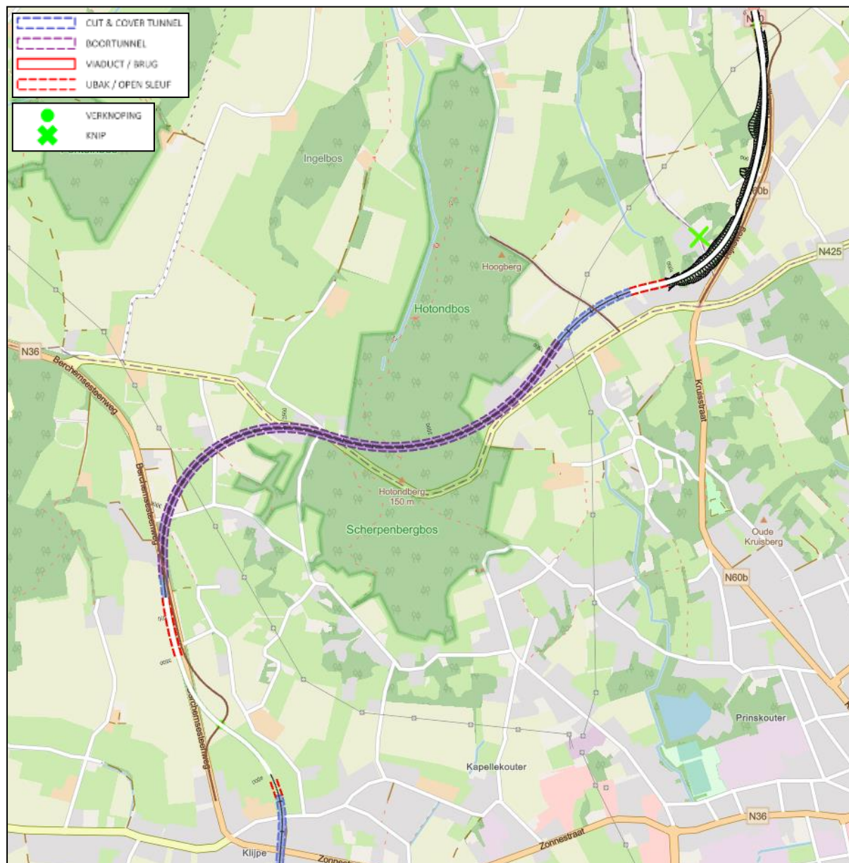
Figuur 5-130 | conceptuitwerking vak 1 van alternatief C2
