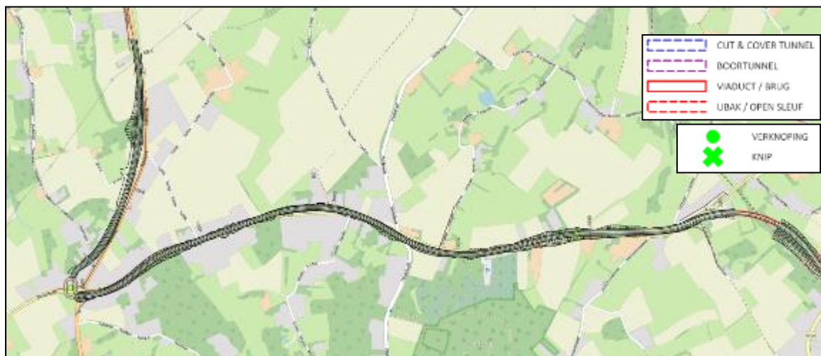
Figuur 5-56 | conceptuutwerking vak 1 van inspraakalternatief I5
