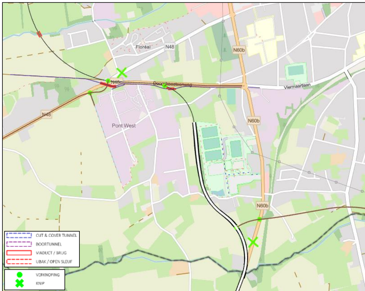
Figuur 5-132 | conceptuitwerking vak 3 van alternatief C2
