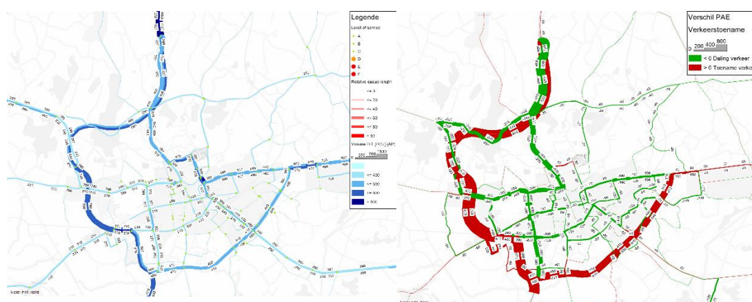
Figuur 5-129 | Verkeersintensiteiten (links) en verschillenplot (rechts) voor alternatief I7
