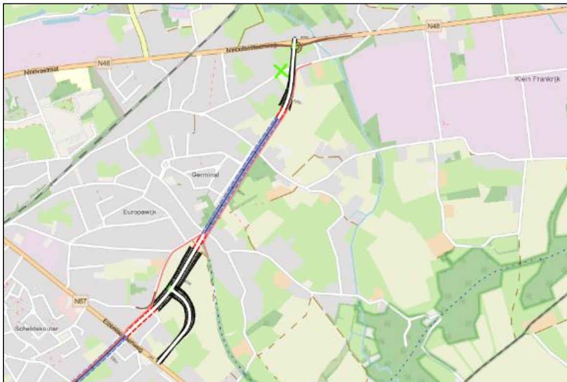
Figuur 5-141 | conceptuitwerking vak 1 van alternatief Z4
