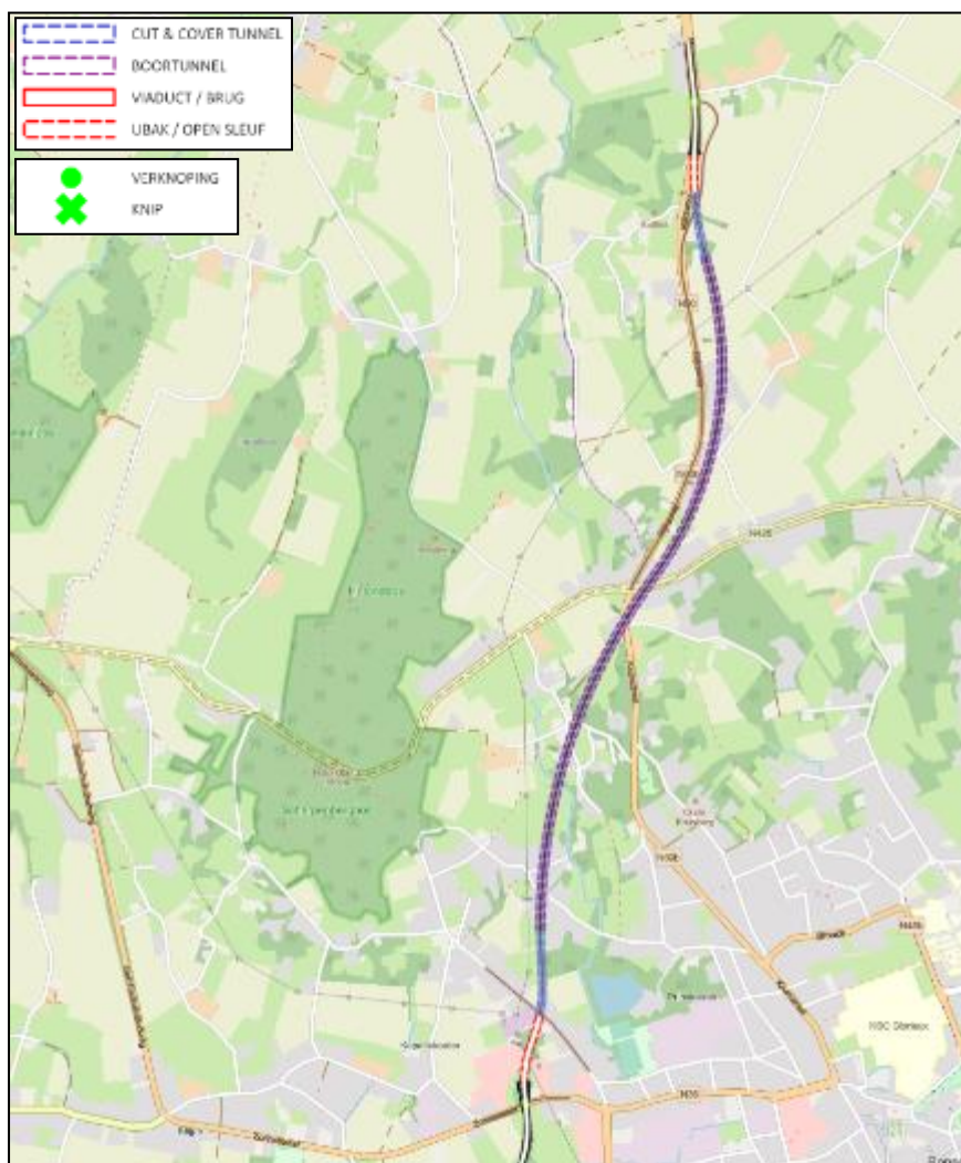
Figuur 5-118 | conceptuitwerking vak 1 van centraal tunnelalternatief T2
