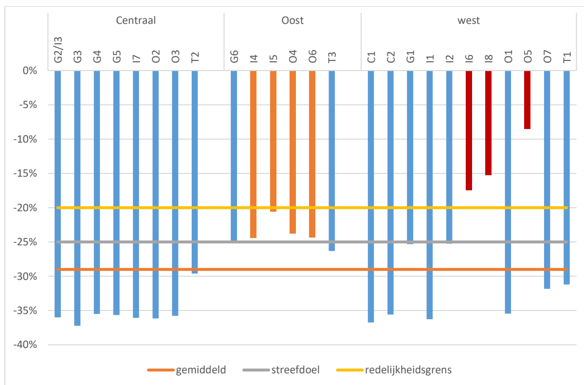
Figuur 5-3 | overzicht evolutie PAE-kilometers in woongebied per alternatief (blauw: voldoet aan het streefdoel, oranje: voldoet niet aan het streefdoel, maar valt binnen de redelijkheidsgrenzen, rood: voldoet niet aan de redelijkheidsgrenzen)
