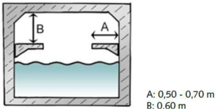
Figuur 40 Voorbeeld mogelijk ontwerp ecoduiker (bron: Prorail)
