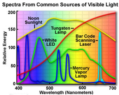
Figuur 92 Spectrum van diverse lichtbronnen, waaronder witte LED als voorbeeld van breedspectrum
