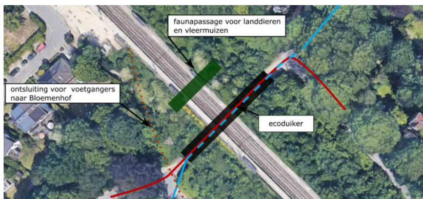
Figuur 20: Faunapassage Linkebeek – variant 2
