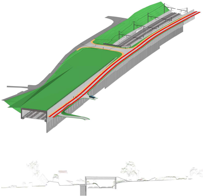
Figuur 5: Overkapping Kleiveld. Bron: TUC RAIL
