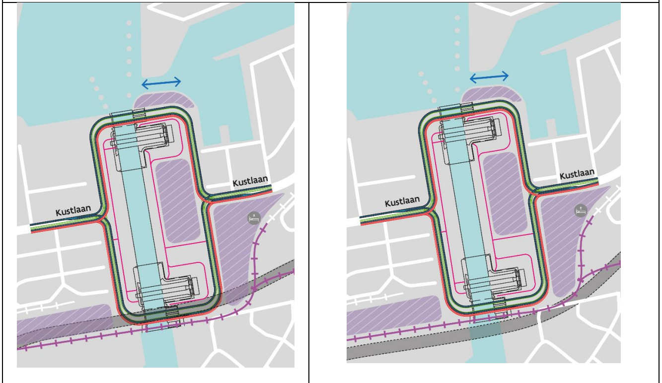
Figuur 16: Visualisatie ligging van de tunnel van de Nx onder de brugkelders en ten zuiden van de brugkelders voor de noordelijke inplanting van de sluis (figuur boven) en de zuidelijke inplanting van de sluis (figuren onder) voor het alternatief met de deurkamers ten oosten.
