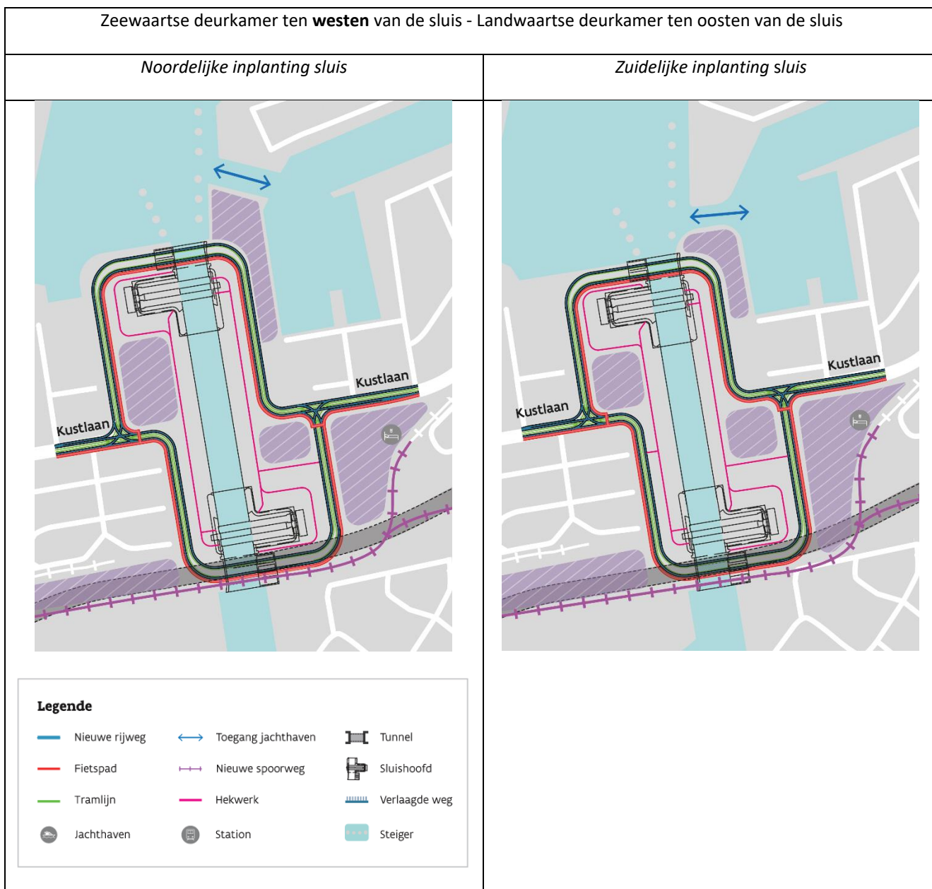
Figuur 15: Visualisatie ligging van de zee- en landwaartse deurkamers ten oosten van de sluis (figuur boven) en zeewaartse deurkamer ten westen en landwaartse deurkamer ten oosten (figuren onder) bij de noordelijke inplanting van de sluis en bij de zuidelijke inplanting van de sluis en de tunnel van de Nx onder de brugkelders.
