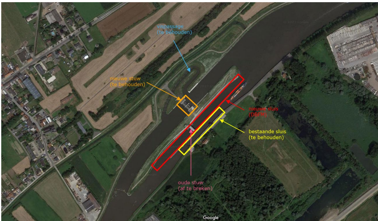
Figuur 3: Situering stuwcomplex te Kerkhove
