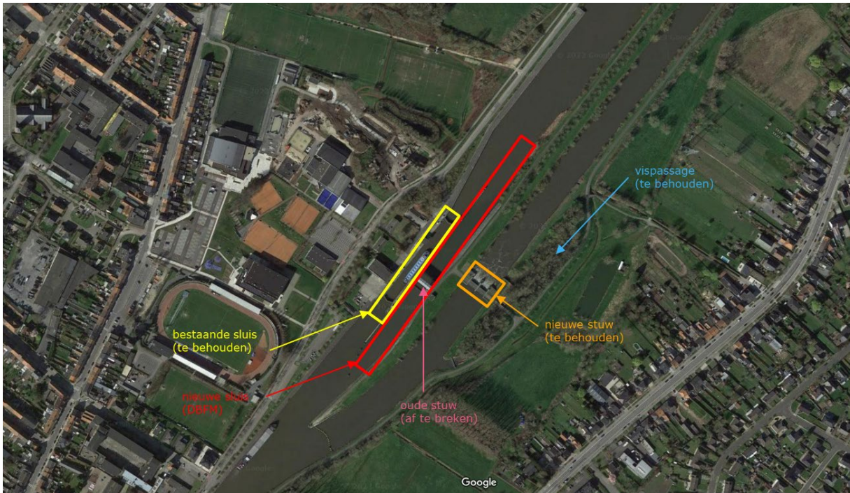
Figuur 2: Situering sluiscomplex te Oudenaarde
