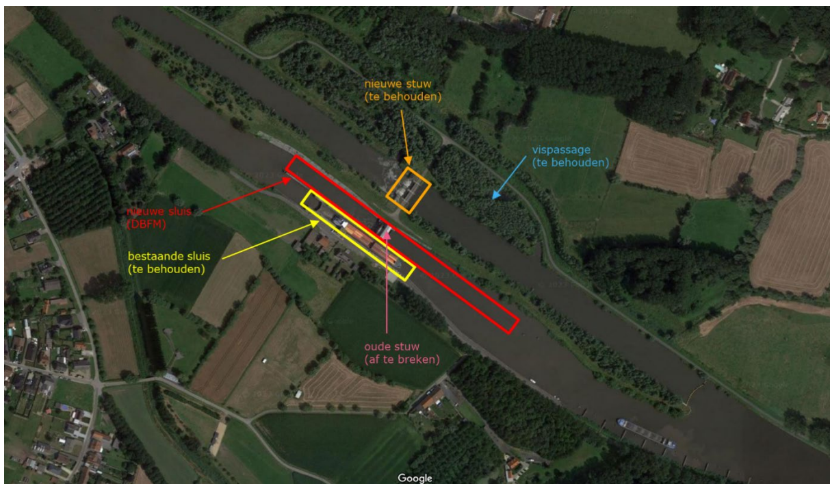
Figuur 1: Situering sluiscomplex te Asper
