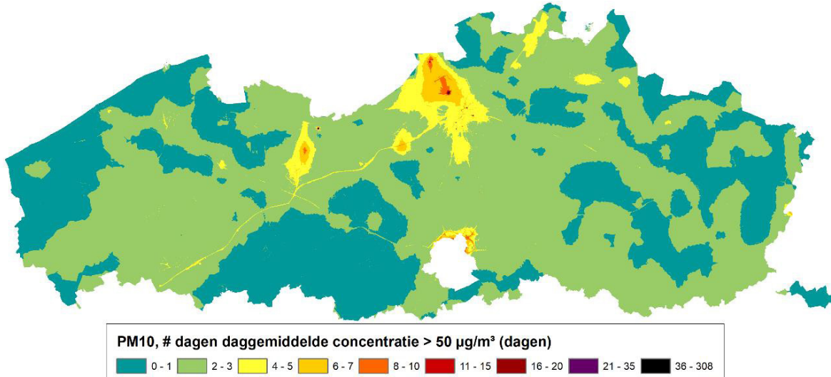
Gemiddeld aantal dagen met een daggemiddelde concentratie > 50 µg/m 3 PM 10 in 2030 volgens het beleidsscenario zoals berekend met het AURORA-RIO-IFDM-OSPM-model
