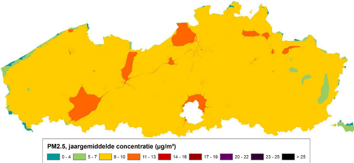
Gemiddelde jaargemiddelde PM 2.5 -concentratie in 2030 volgens het beleidsscenario zoals berekend met het AURORA-RIO-IFDM-OSPM-model
