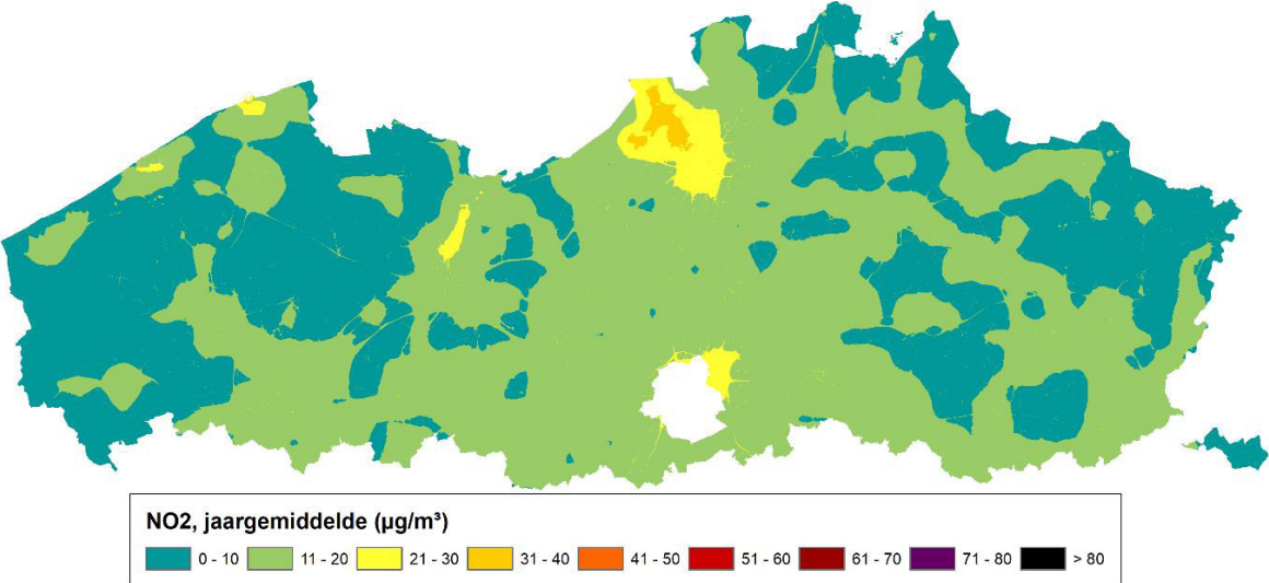
Gemiddelde jaargemiddelde NO 2 -concentratie in 2025 volgens het beleidsscenario zoals berekend met het AURORA-RIO-IFDM-OSPM-model
