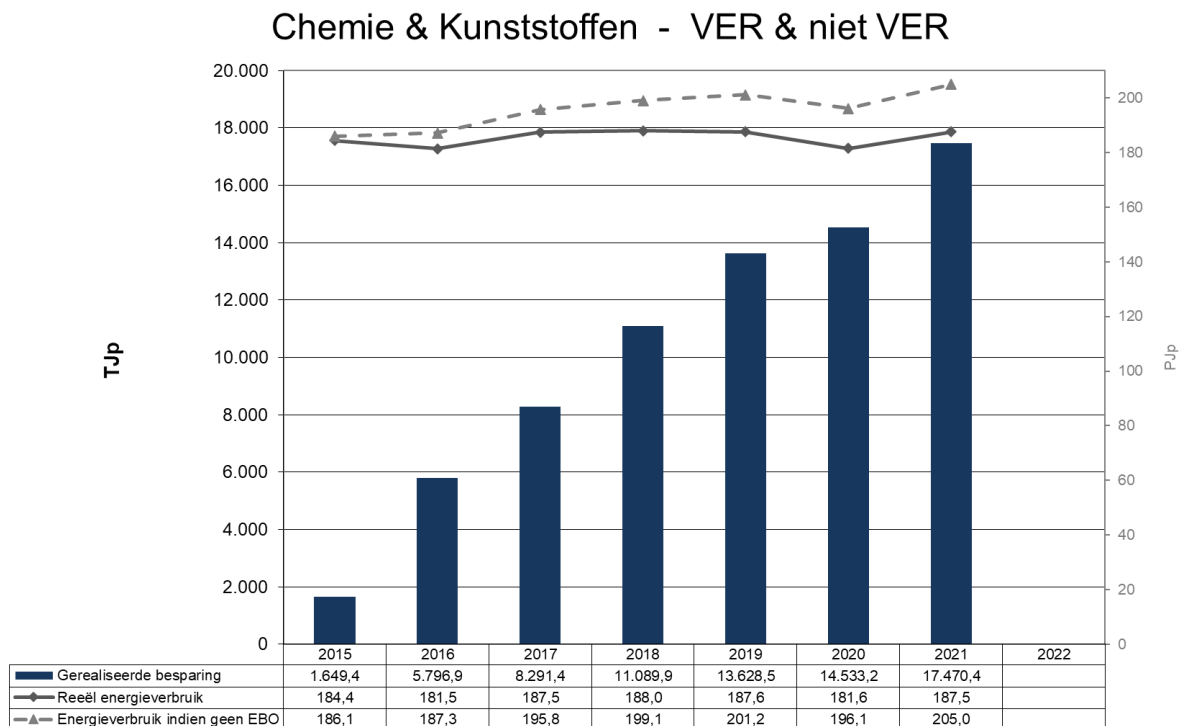
Grafiek 4: Gerealiseerde besparingen Chemie & Kunststoffen (VER en niet VER-bedrijven)
