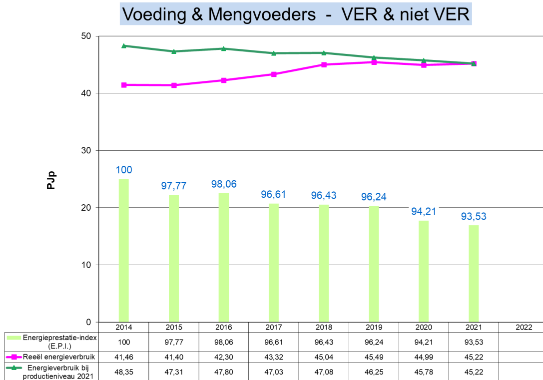
Grafiek 36: Evolutie 2014 – 2021 van het energieverbruik en de E.P.I. voor Voeding & Mengvoeders (VER en niet VER-bedrijven)
