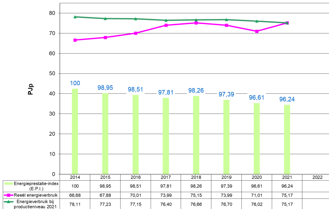
Grafiek 28: Evolutie 2014 – 2021 van het energieverbruik en de E.P.I. voor de niet VER-bedrijven
