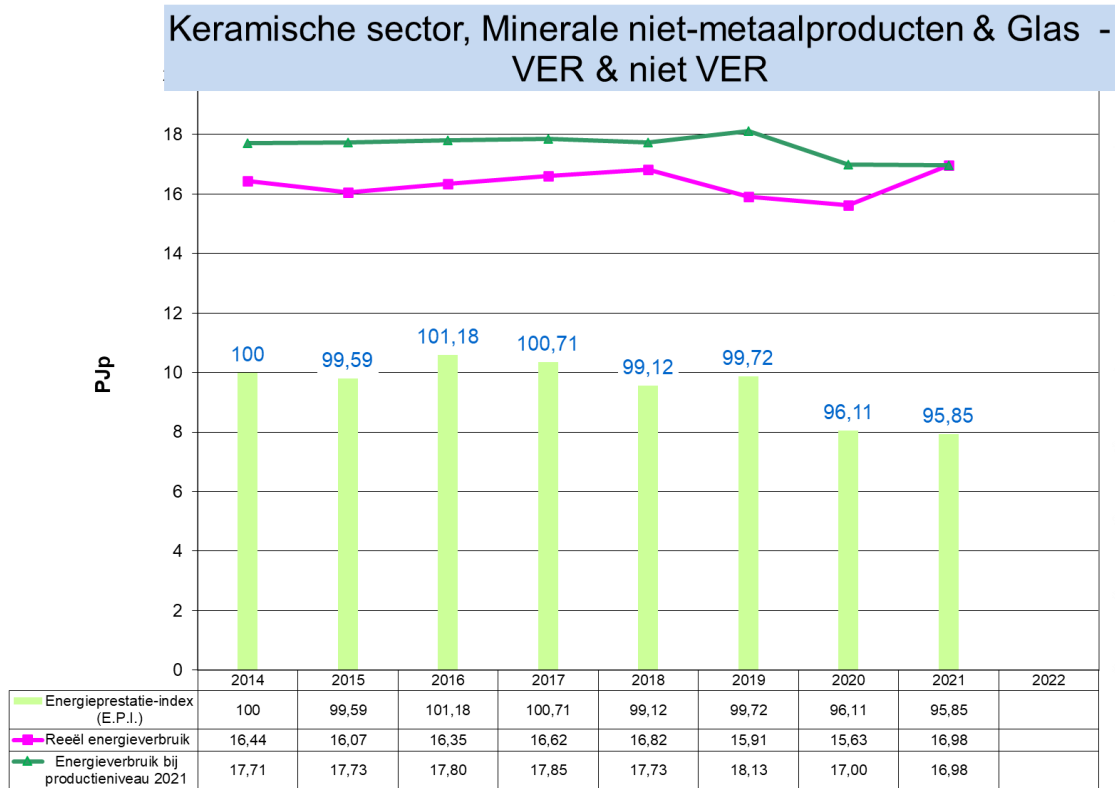
Grafiek 45: Evolutie 2014 – 2021 van het energieverbruik en de E.P.I. voor Keramische sector, Minerale niet-metaalproducten & Glas (VER en niet VER-bedrijven)
