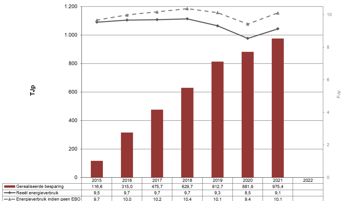
Grafiek 16: Gerealiseerde besparingen Non-ferro & Metaalverwerking (niet VER-bedrijven)
