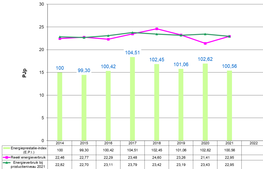
Grafiek 40: Evolutie 2014 – 2021 van het energieverbruik en de E.P.I. voor Non-ferro & Metaalverwerking (VER-bedrijven)
