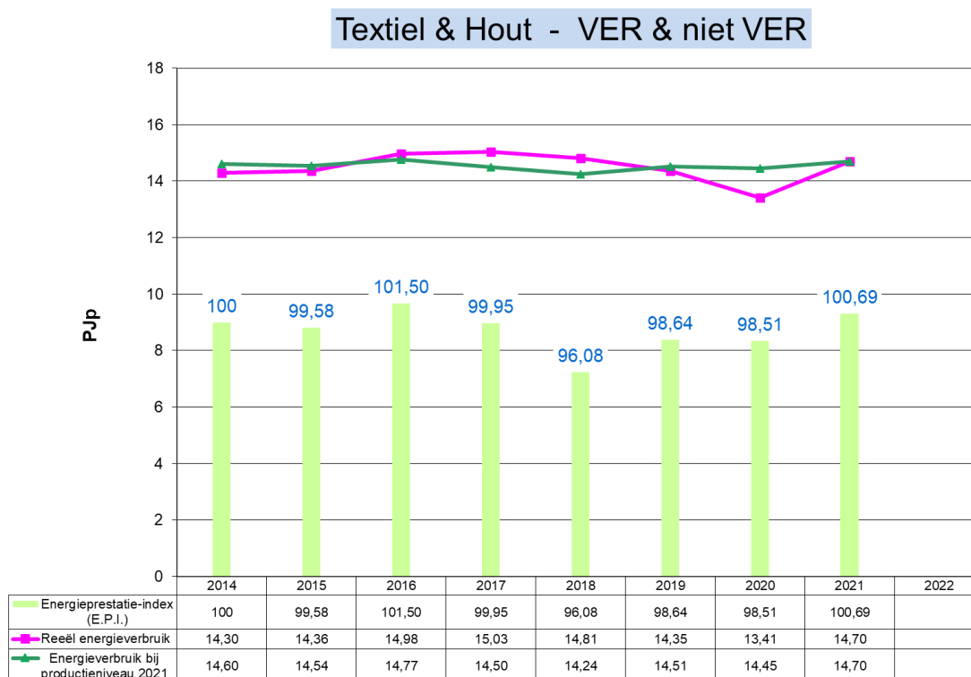
Grafiek 42: Evolutie 2014 – 2021 van het energieverbruik en de E.P.I. voor Textiel & Hout (VER en niet VER-bedrijven)
