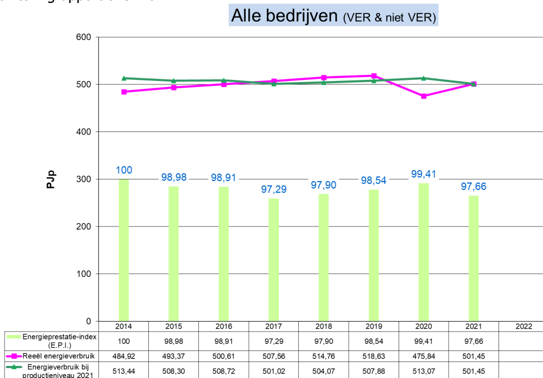
Grafiek 26: Evolutie 2014 – 2021 van het energieverbruik en de E.P.I. voor alle bedrijven
