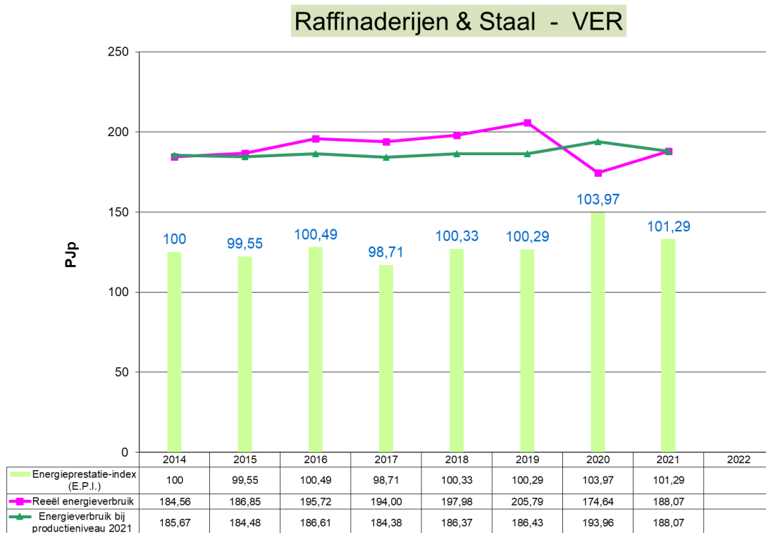
Grafiek 32: Evolutie 2014 – 2021 van het energieverbruik en de E.P.I. voor Raffinaderijen & Staal (VER-bedrijven)
