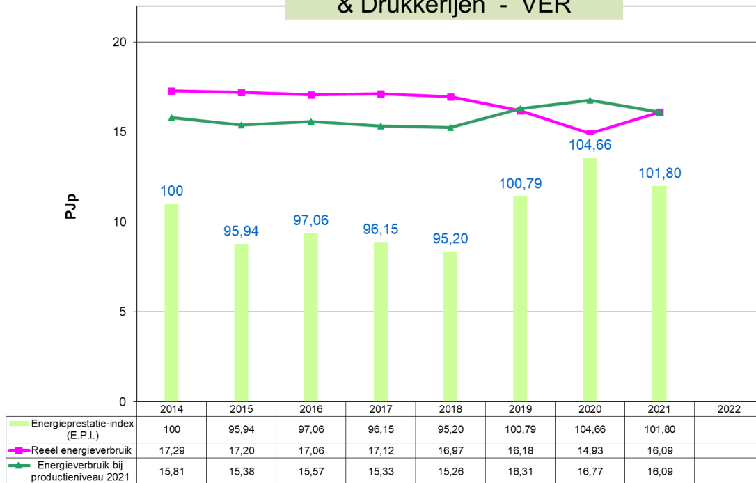
Grafiek 34: Evolutie 2014 – 2021 van het energieverbruik en de E.P.I. voor Papier, Papier- en kartonverwerking & Drukkerijen (VER-bedrijven)
