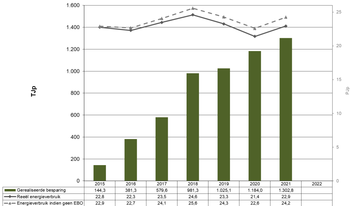
Grafiek 15: Gerealiseerde besparingen Non-ferro & Metaalverwerking (VER-bedrijven)
