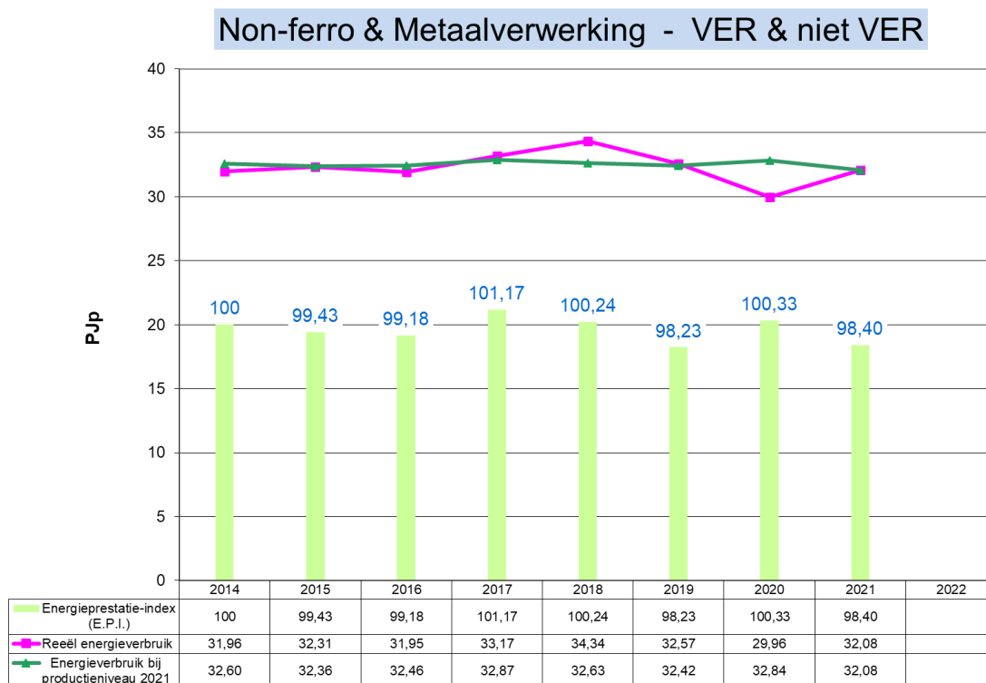
Grafiek 39: Evolutie 2014 – 2021 van het energieverbruik en de E.P.I. voor Non-ferro & Metaalverwerking (VER en niet VER-bedrijven)
