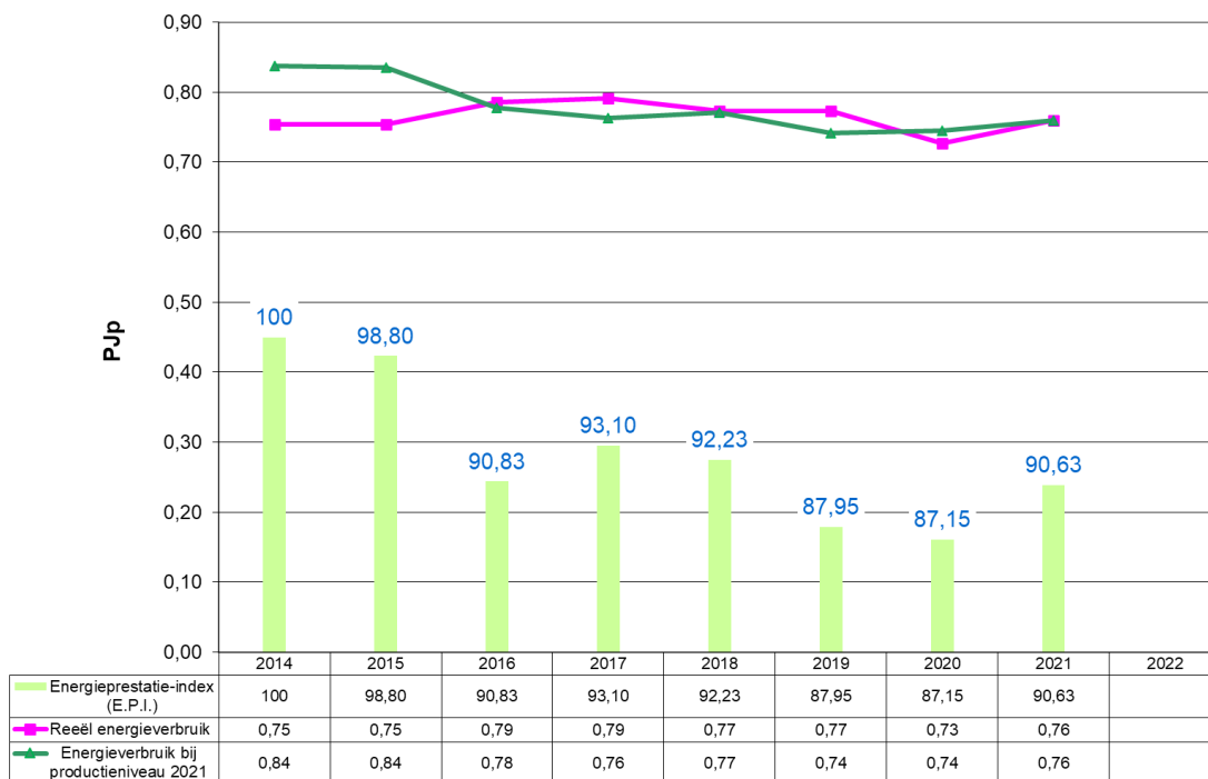
Grafiek 35: Evolutie 2014 – 2021 van het energieverbruik en de E.P.I. voor Papier, Papier- en kartonverwerking & Drukkerijen (niet VER-bedrijven)
