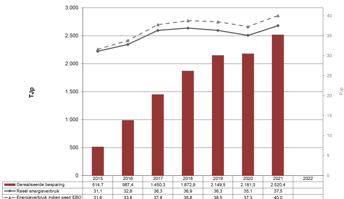
Grafiek 6: Gerealiseerde besparingen Chemie & Kunststoffen (niet VER-bedrijven)
