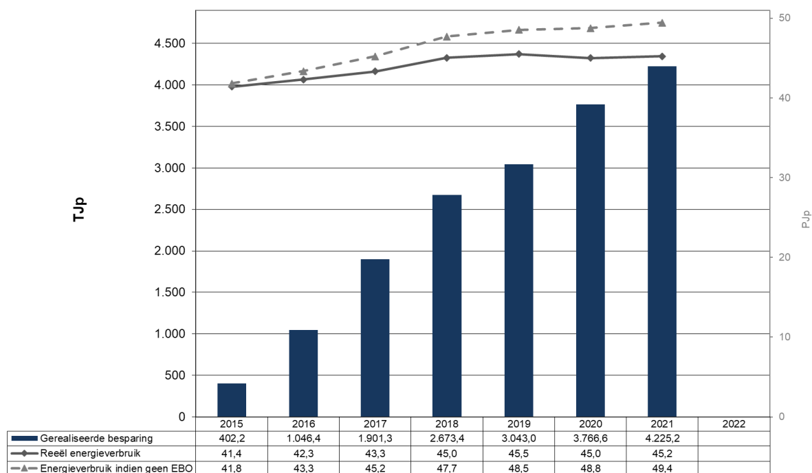
Grafiek 11: Gerealiseerde besparingen Voeding & Mengvoeders (VER en niet VER-bedrijven)
