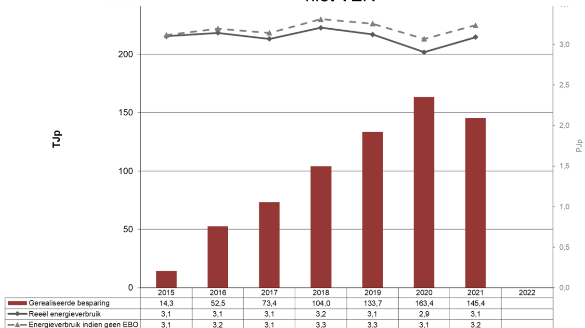
Grafiek 22: Gerealiseerde besparingen Keramische sector, Minerale niet-metaalproducten & Glas (niet VER-bedrijven)
