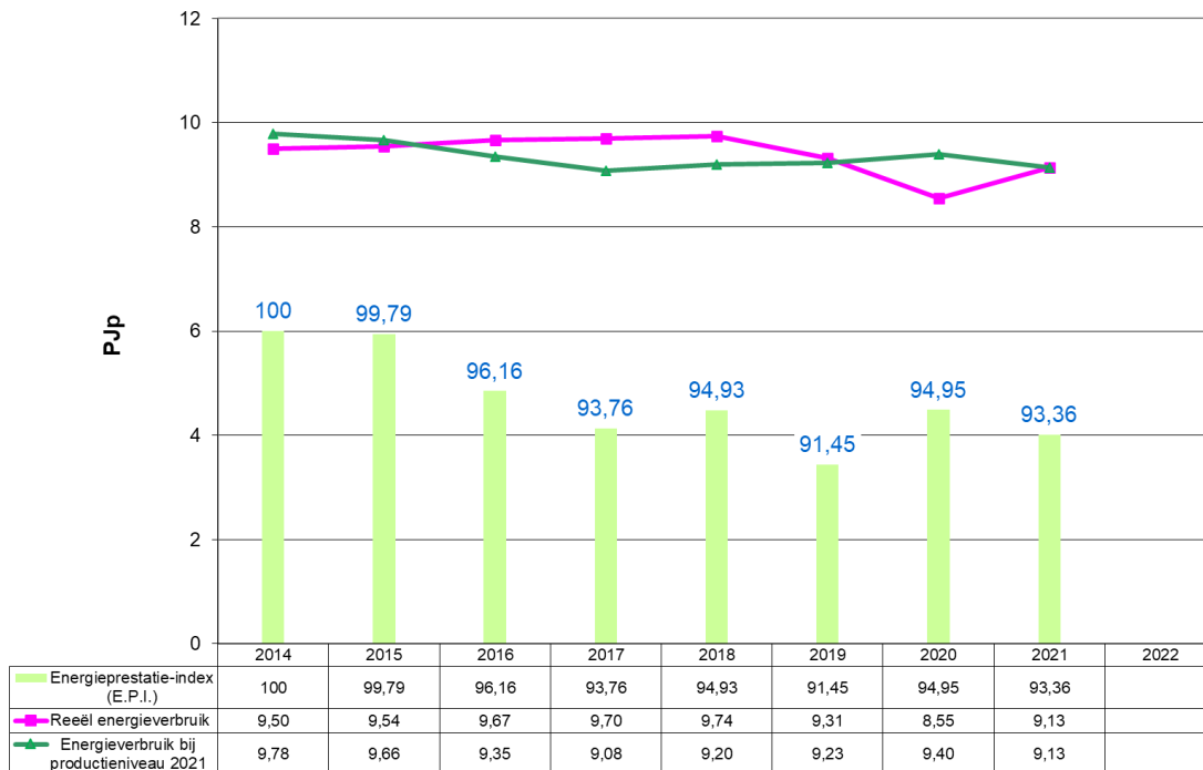
Grafiek 41: Evolutie 2014 – 2021 van het energieverbruik en de E.P.I. voor Non-ferro & Metaalverwerking (niet VER-bedrijven)
