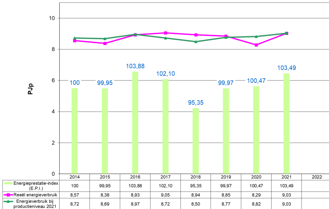
Grafiek 43: Evolutie 2014 – 2021 van het energieverbruik en de E.P.I. voor Textiel & Hout (VER-bedrijven)
