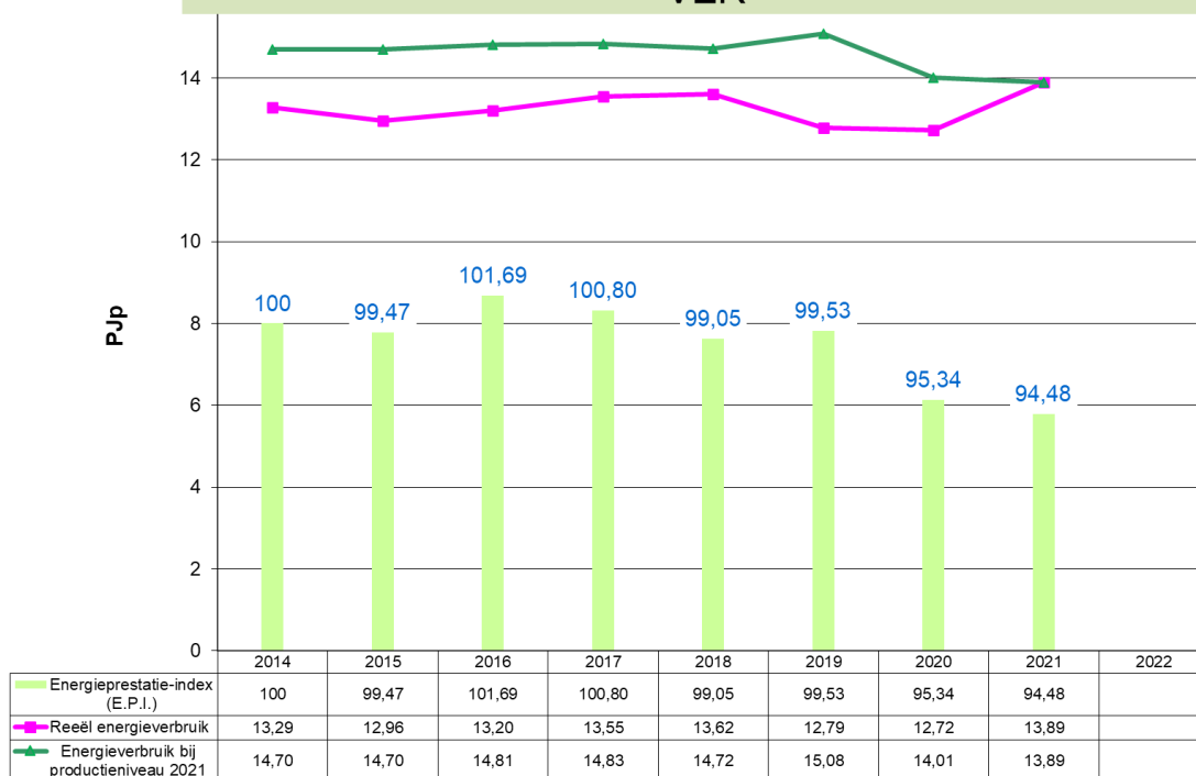
Grafiek 46: Evolutie 2014 – 2021 van het energieverbruik en de E.P.I. voor Keramische sector, Minerale niet-metaalproducten & Glas (VER-bedrijven)
