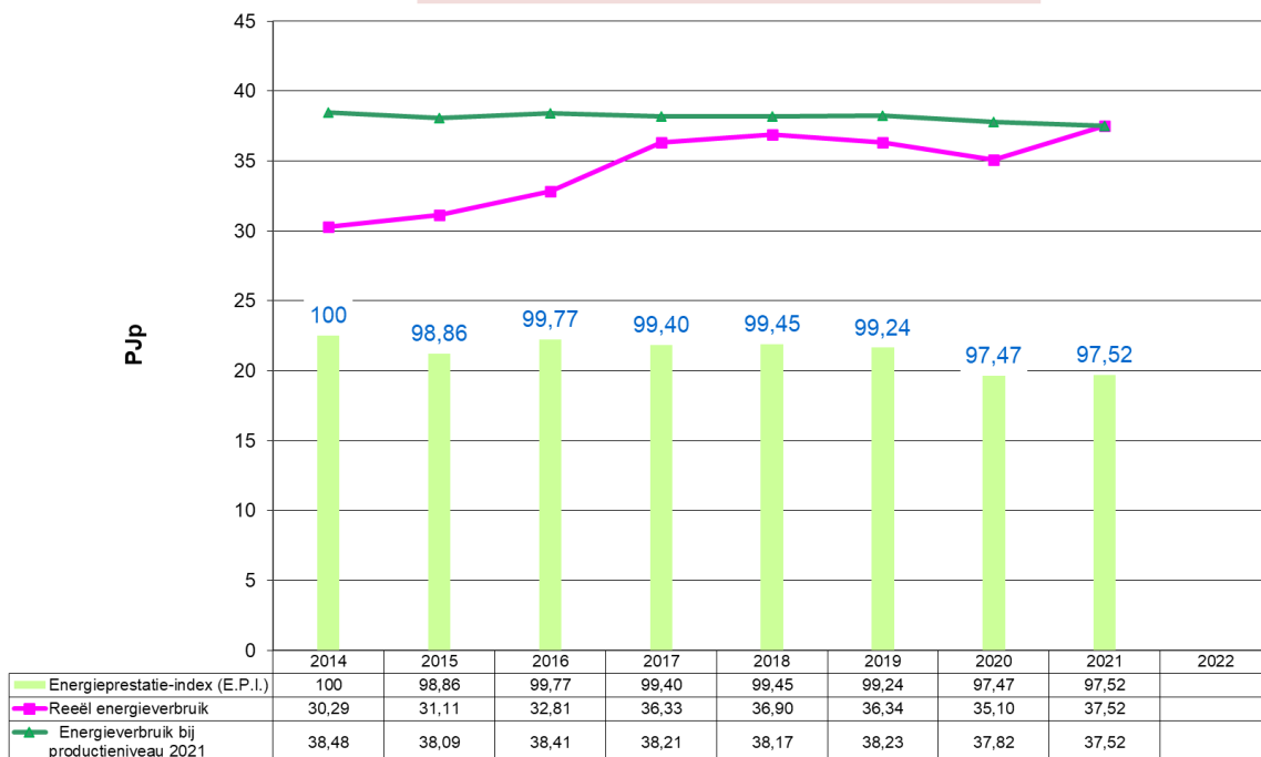
Grafiek 31: Evolutie 2014 – 2021 van het energieverbruik en de E.P.I. voor Chemie & Kunststoffen (niet VER-bedrijven)
