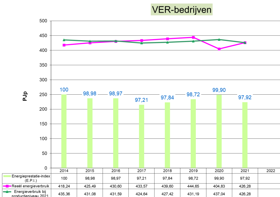
Grafiek 27: Evolutie 2014 – 2021 van het energieverbruik en de E.P.I. voor de VER-bedrijven
