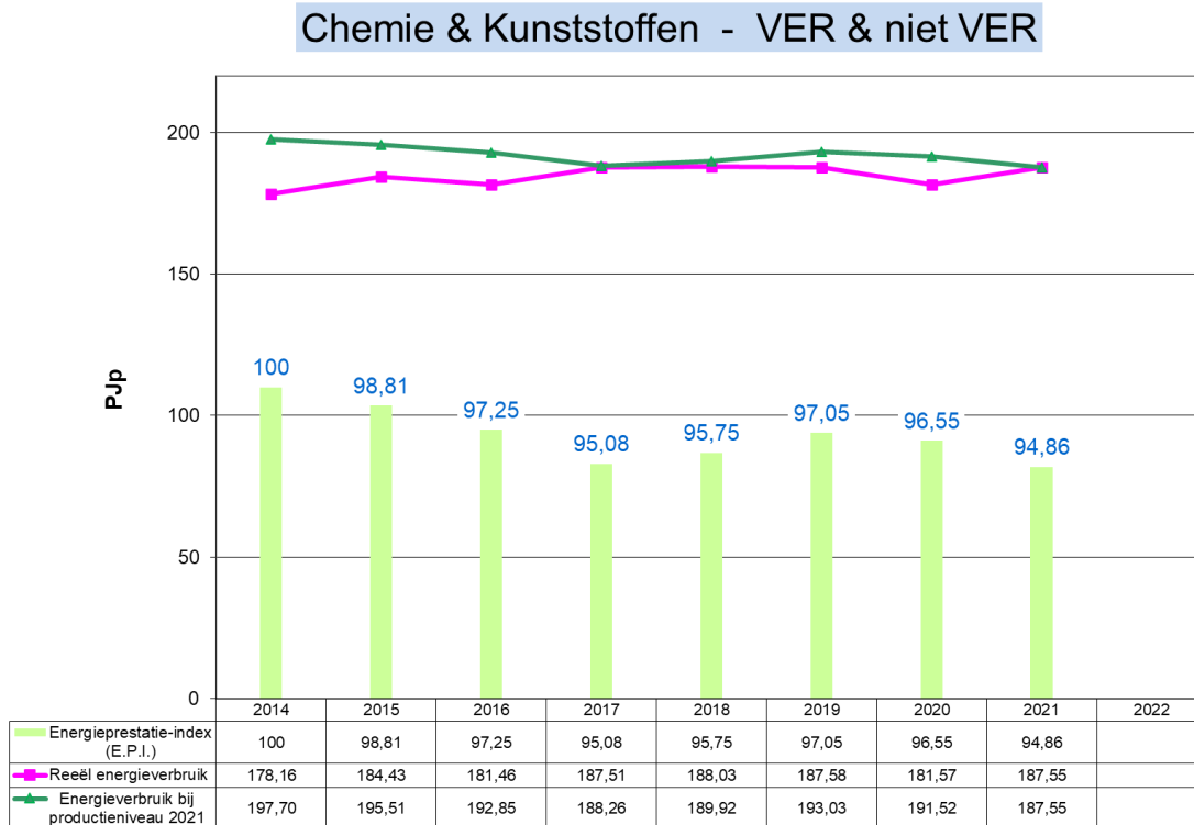
Grafiek 29: Evolutie 2014 – 2021 van het energieverbruik en de E.P.I. voor Chemie & Kunststoffen (VER en niet VER-bedrijven)
