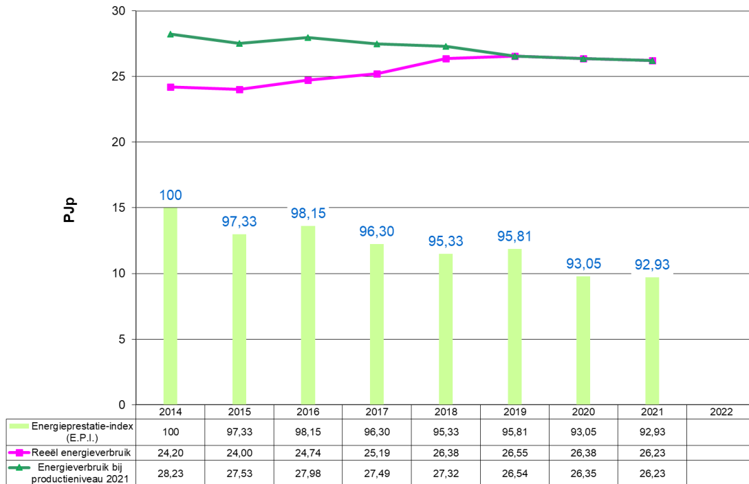
Grafiek 37: Evolutie 2014 – 2021 van het energieverbruik en de E.P.I. voor Voeding & Mengvoeders (VER-bedrijven)
