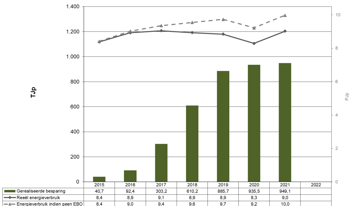
Grafiek 18: Gerealiseerde besparingen Textiel & Hout (VER en niet VER-bedrijven)
