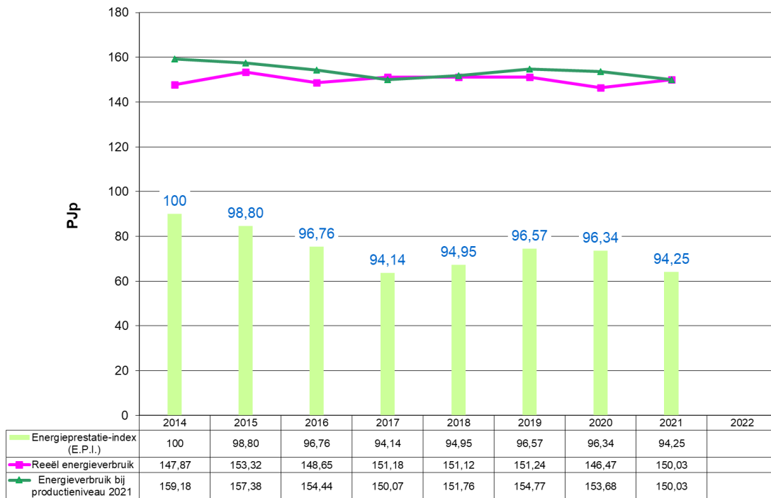
Grafiek 30: Evolutie 2014 – 2021 van het energieverbruik en de E.P.I. voor Chemie & Kunststoffen (VER-bedrijven)
