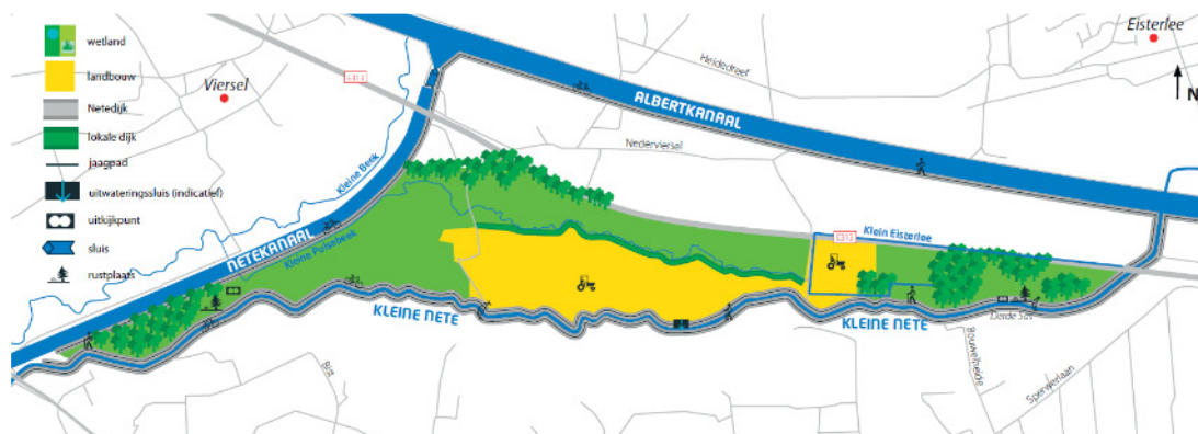
Figuur 2-5 Inrichtingsplan Sigmaproject Varenheuvel-Abroek
