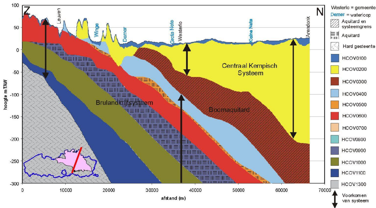
Figuur 2. Zuidwest-noordoost profiel door het Centraal Kempisch Stelsysteem en het Brulandkrijtsysteem
