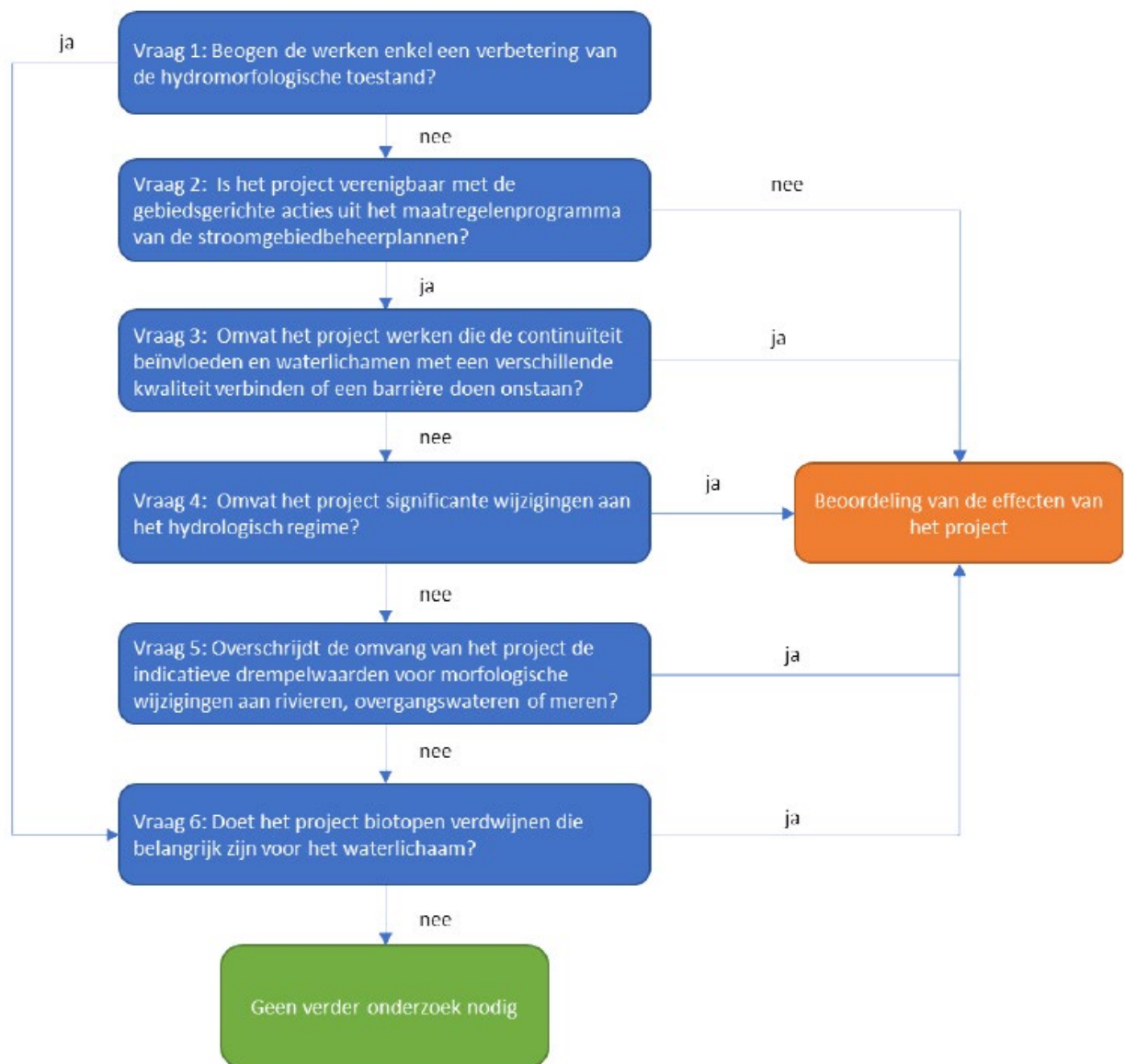
Figuur 9-7: Stroomschema toets voor verder onderzoek bij hydromorfologische wijzigingen (bron: CIW, 2019)
