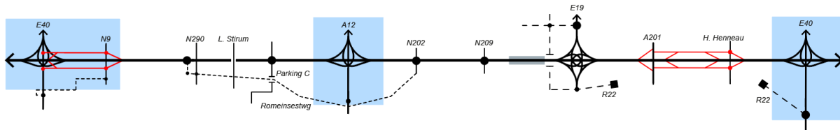
Figuur 156: Lijnschema Alternatief 1 met asymmetrische 3/4 knopen
