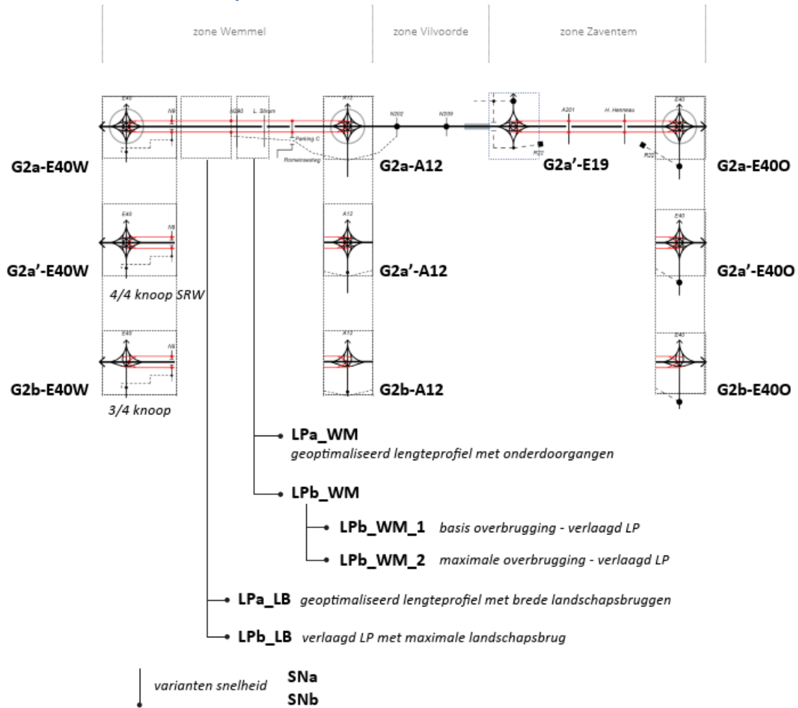
Figuur 167: Lijnschema's Alternatief 2 en zijn varianten loop 2
