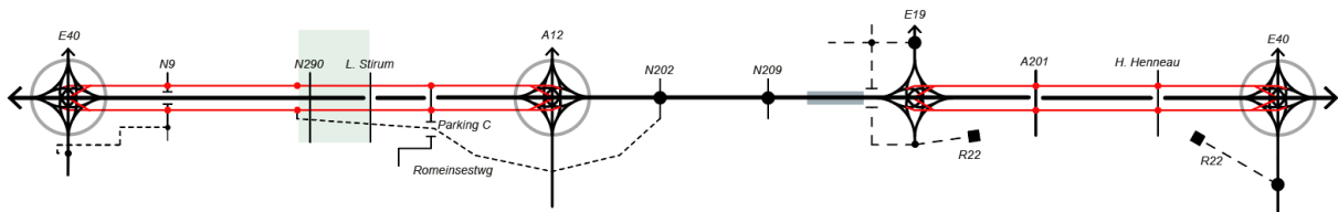
Figuur 173: Lijnschema alternatief loop 2 – G2a met LPb-WM-2
