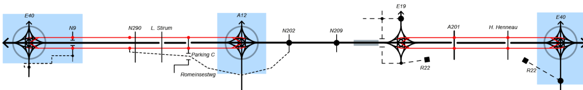
figuur 157: Lijnschema Alternatief 2 met symmetrische 4/4 knopen op SRW en DRW
