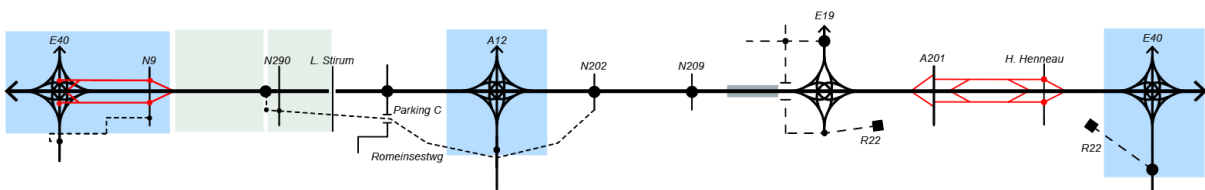
Figuur 162: Lijnschema alternatief G1a
