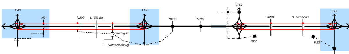
Figuur 170: Lijnschema alternatief loop 2 – G2b
