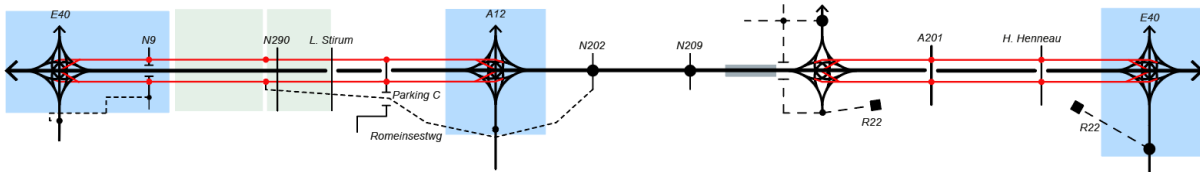
Figuur 154: Lijnschema Alternatief 2 met variabele elementen
