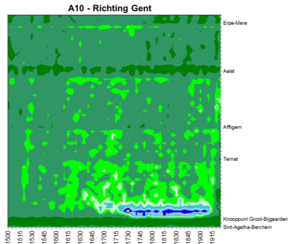
Figuur 46 - XT-diagram situatie 2013 - A10/E40 richting Gent avondspits (bron: Microsimulatiemodel hoofdwegennet Brussel, MOW - cel verkeersmodellen)
