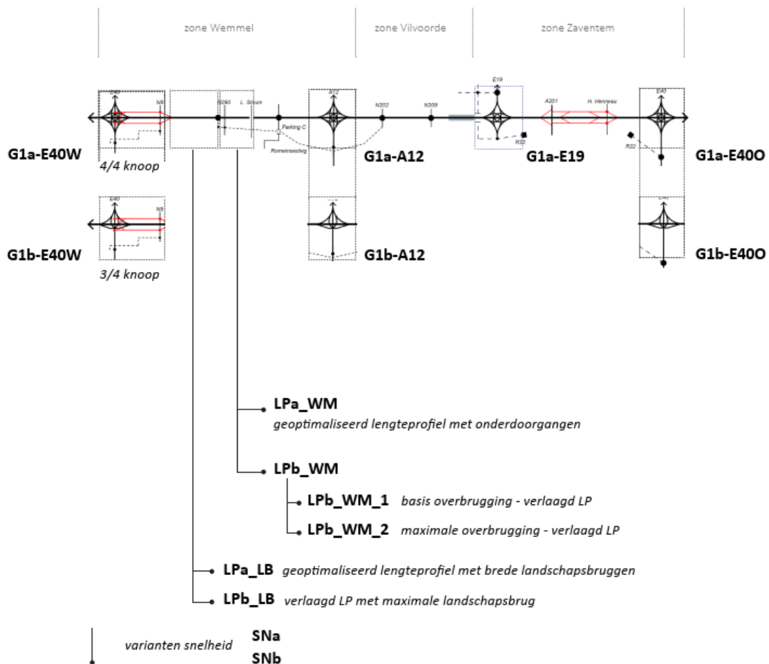
Figuur 160: Lijnschema's Alternatief 1 en zijn varianten loop 2
