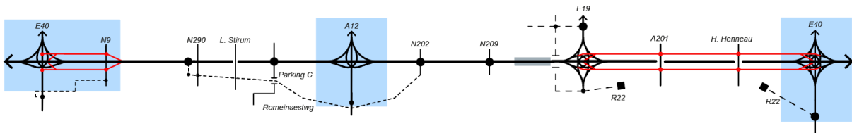
Figuur 176: Lijnschema alternatief 3 ba loop 2 – G1b/G1b/G2a’
