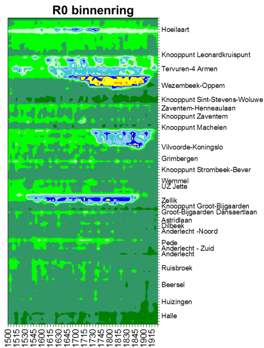
Figuur 44 - XT-diagram situatie 2013 - R0 binnenring avondspits (bron: Microsimulatiemodel hoofdwegennet Brussel, MOW - cel verkeersmodellen)
