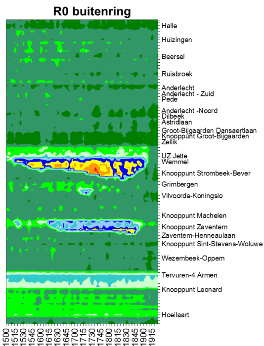
Figuur 45 - XT-diagram situatie 2013 - R0 buitenring avondspits (bron: Microsimulatiemodel hoofdwegennet Brussel, MOW - cel verkeersmodellen)
