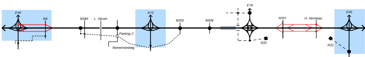
Figuur 163: Lijnschema alternatief G1b
