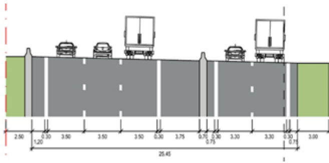
Figuur 151: Typedwarsprofiel Alternatief 2 loop 2
