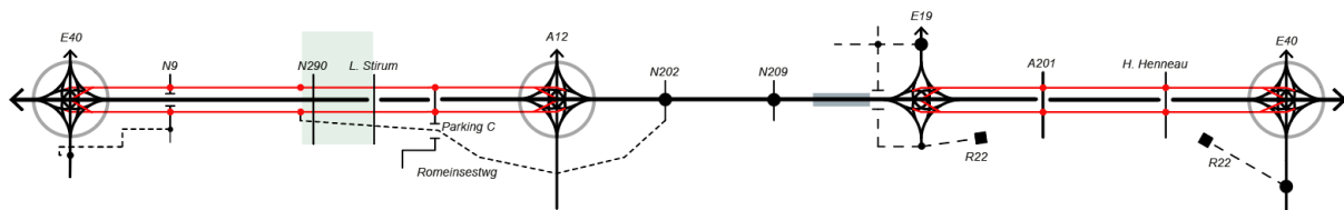
Figuur 172: Lijnschema alternatief loop 2 – G2a met LPb-WM-1
