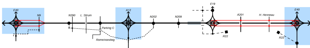
Figuur 175: Lijnschema alternatief 3 a loop 2 – G1a/G1a/G2a'
