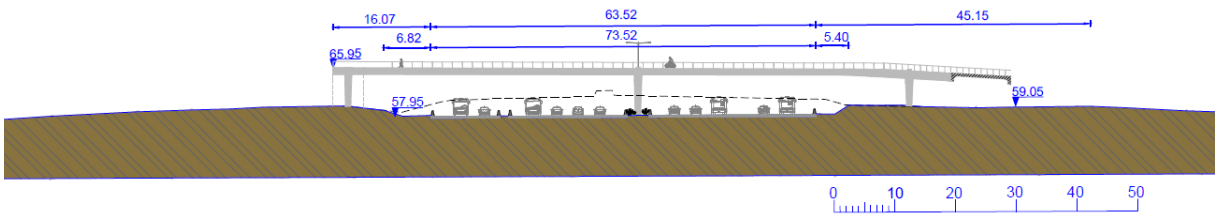
Figuur 30: Dwarsprofiel A - G1 LPb_LB
