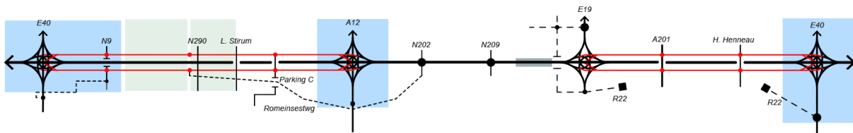
Figuur 130: Lijnschema alternatief 2
