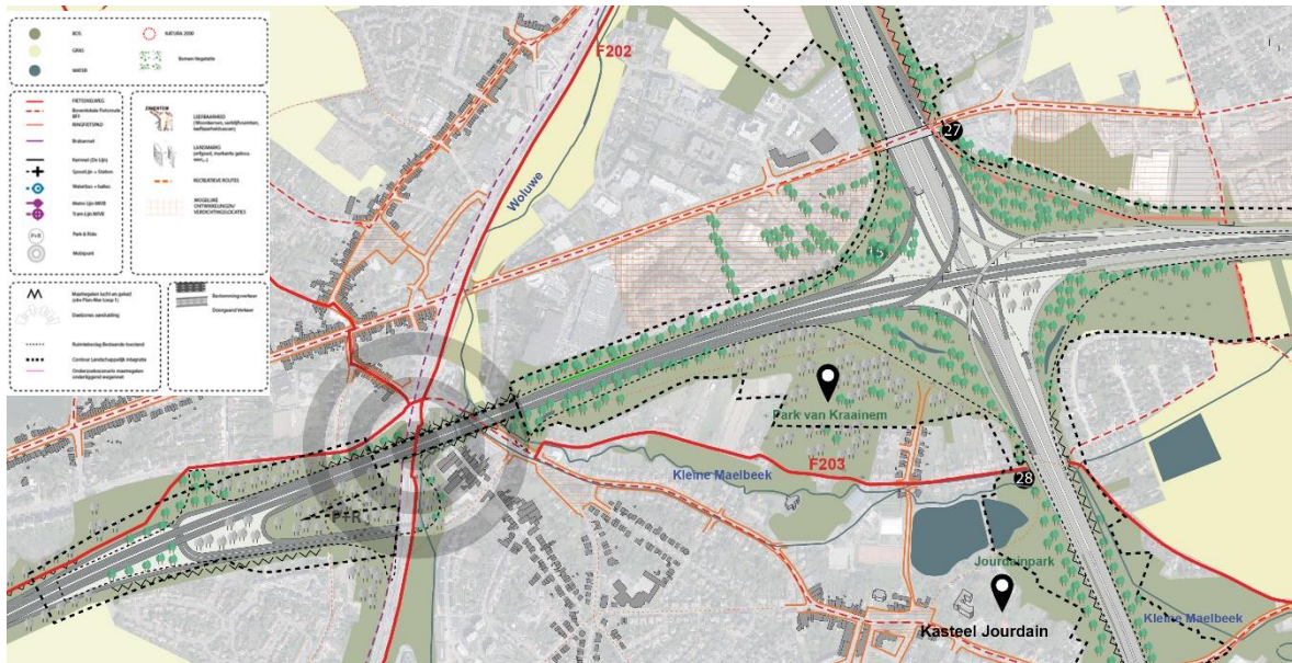
Figuur 122: Verkeerswisselaar R0/E40 Sint-Stevens-Woluwe variant G2a (Loop 2)
