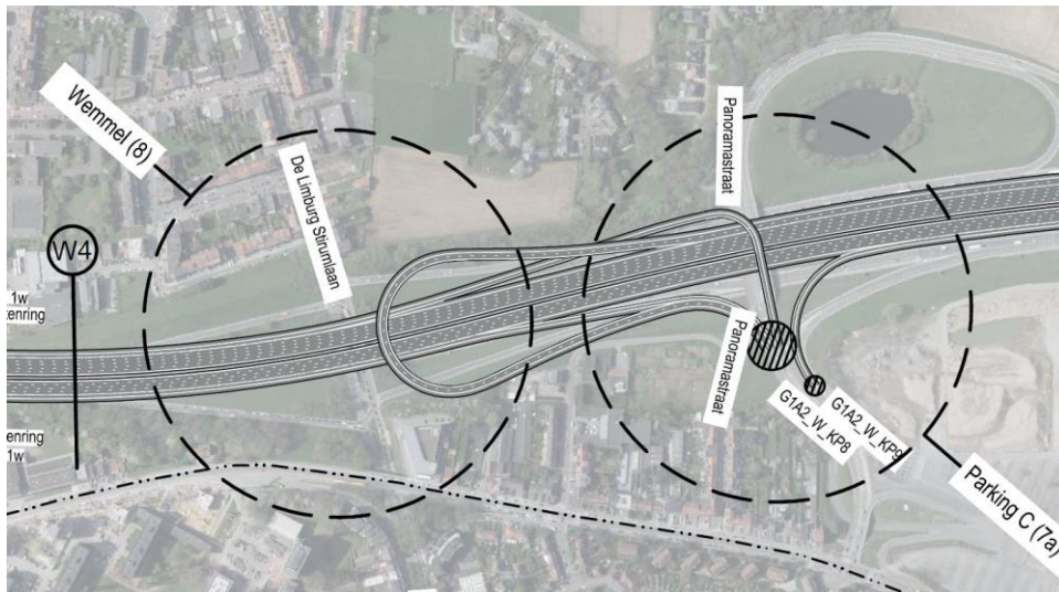
Figuur 74: Aansluitingscomplex 7a – Parking C in G1A2 – Loop 1
