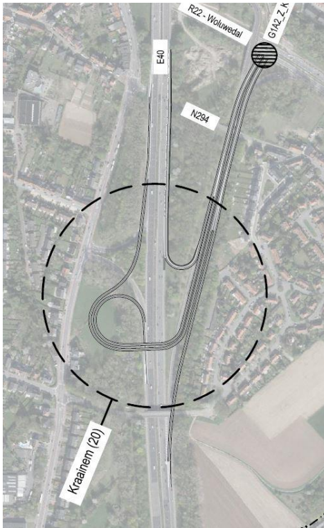
Figuur 81: Aansluitingscomplex 20 Kraainem in G1A2 – Loop 1
