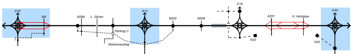
figuur 105: Lijnschema alternatief 1 met symmetrische 4/4 knoopen (G1a)
