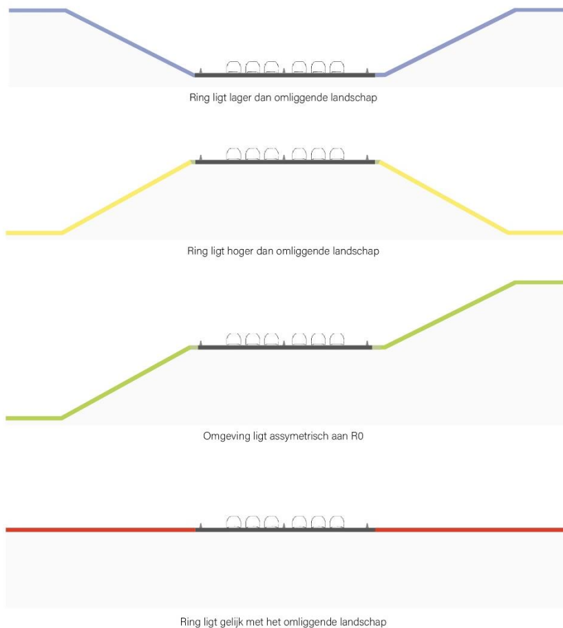
Figuur 85: Overzicht ligging R0-Noord t.o.v. omliggende maaiveld - bestaande toestand
