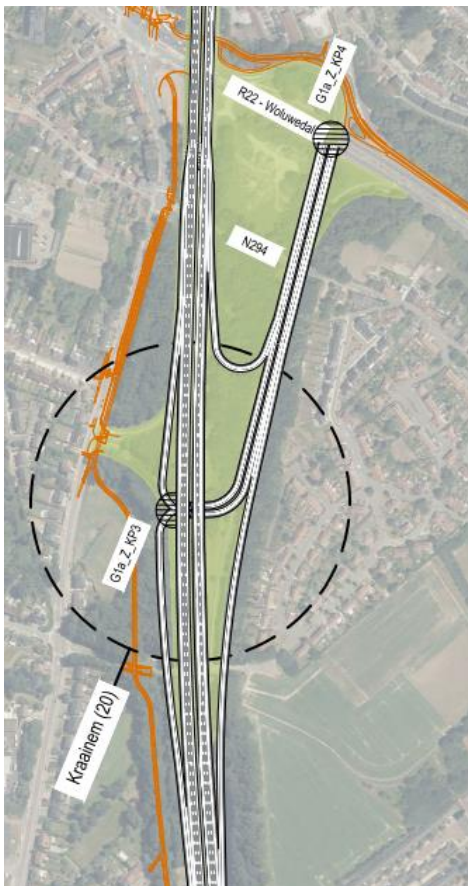
Figuur 82: Aansluitingscomplex 20 Kraainem in G1 – Loop 2
