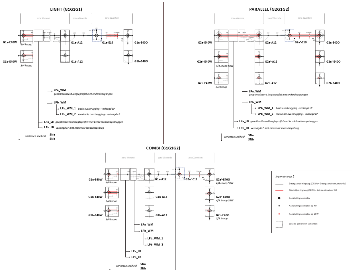
Figuur 153: Overzicht (lijnschema's) alternatieven en varianten Loop 2
