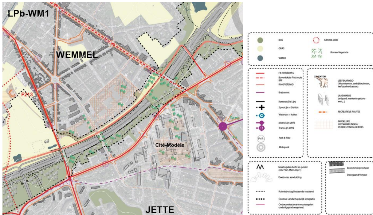
Figuur 37: Ruimtelijke uitwerking verlaagd lengteprofiel met basis overbrugging zone Wemmel-Jette – Loop 2 (LPb_WM1)
