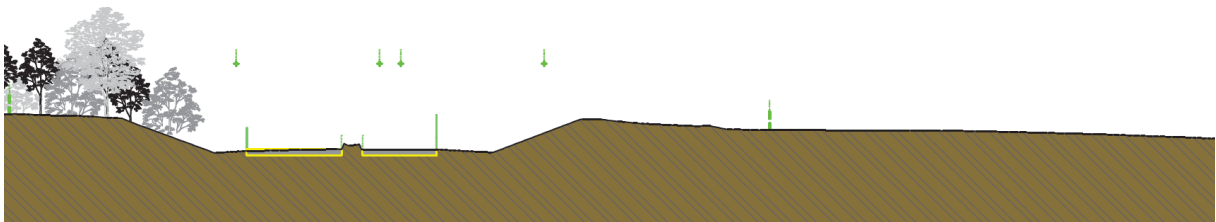
Figuur 31: Dwarsprofiel B - bestaande toestand
