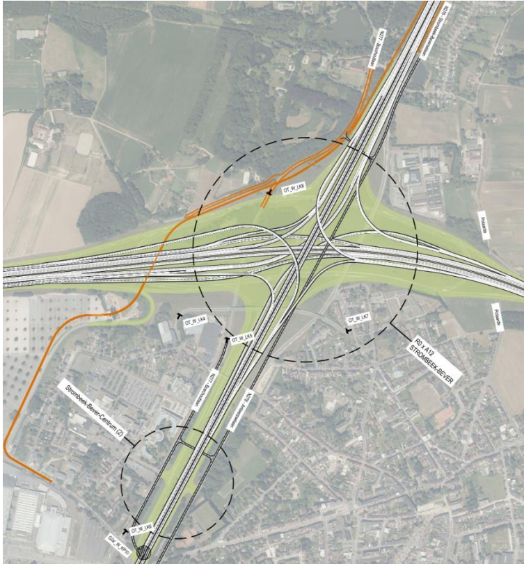
Figuur 65: Verkeerswisselaar/ knoop A12 Strombeek-Bever variant a' in G2 – Loop 2 → variant 4/4 knoop SRW
