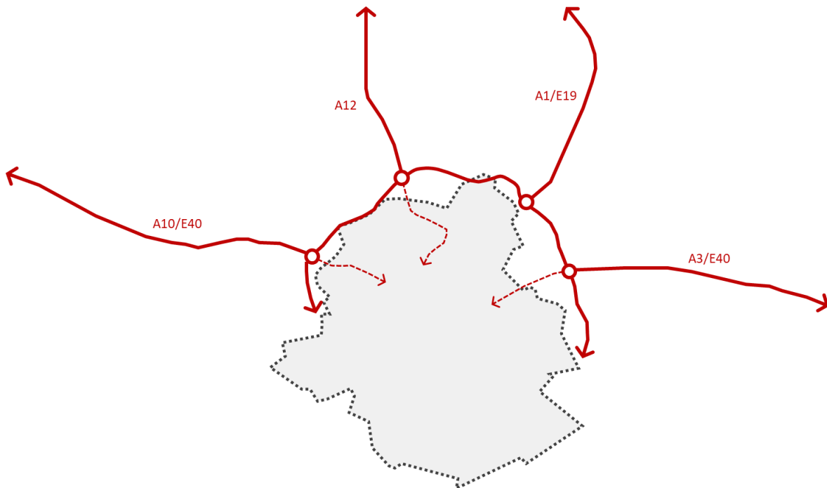
Figuur 44: Verkeerswisselaars/ -knoten realiseren de verbinding tussen de toeleidende radiale snelwegen (E40/A10-GB, A12, E19, E40/A3-SSW) en de R0-Noord
