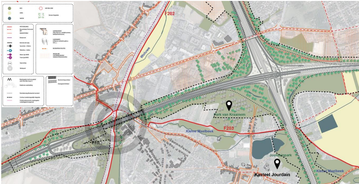
Figuur 124: Verkeerswisselaar R0/E40 Sint-Stevens-Woluwe variant G2b (Loop 2)
