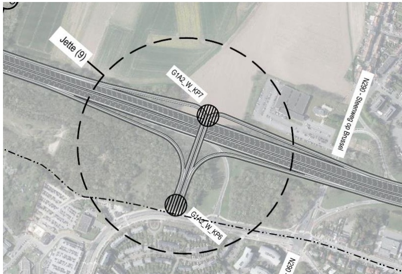
Figuur 72: Aansluitingscomplex 9 Jette/N290 in G1A2 – Loop 1
