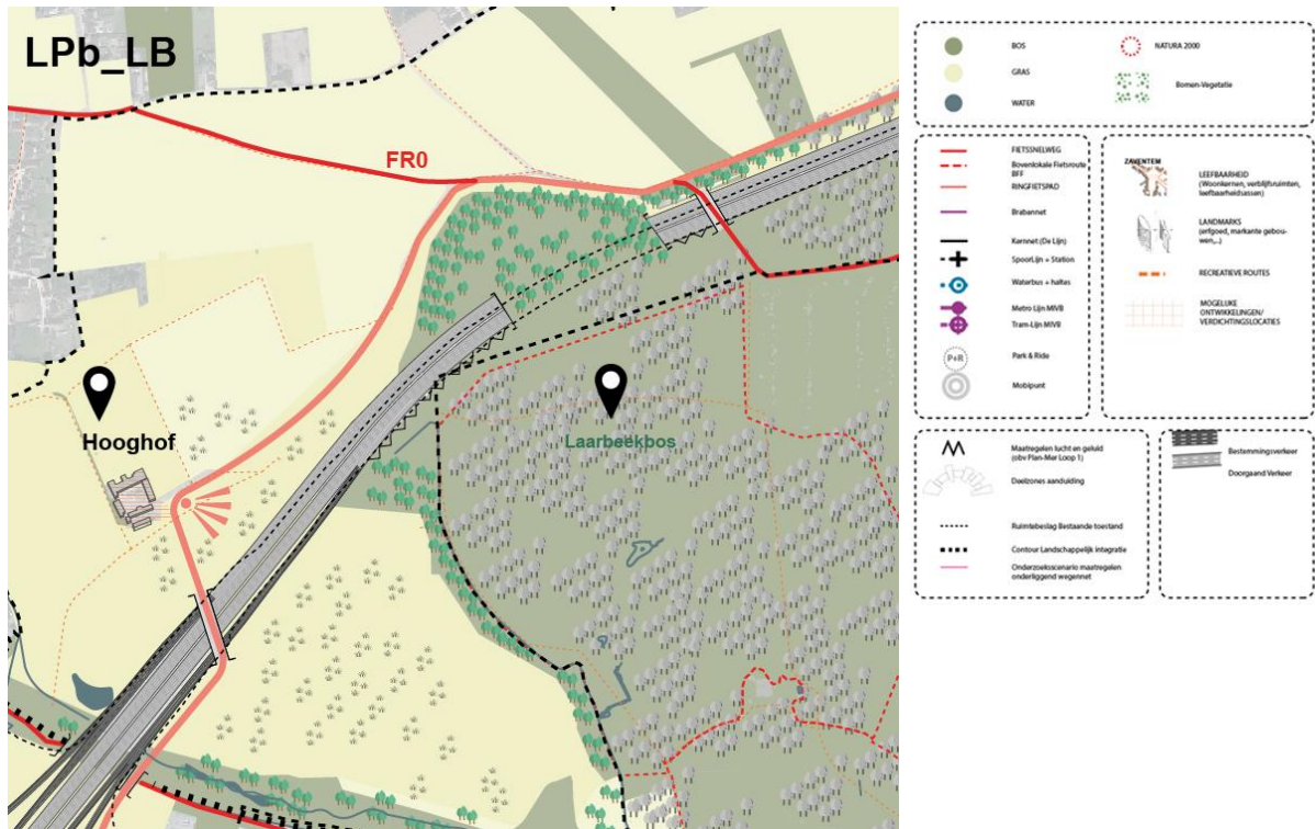
Figuur 126: Geoptimaliseerd lengteprofiel b met één maximale landschapsbrug (LPb LB) deelzone Laarbeekbos (illustratie voor alternatief 1)
