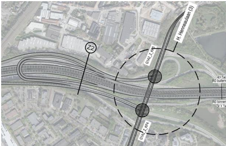
Figuur 79: Aansluitingscomplex 3 – H. Henneaulaan in G1A2 – Loop 1
