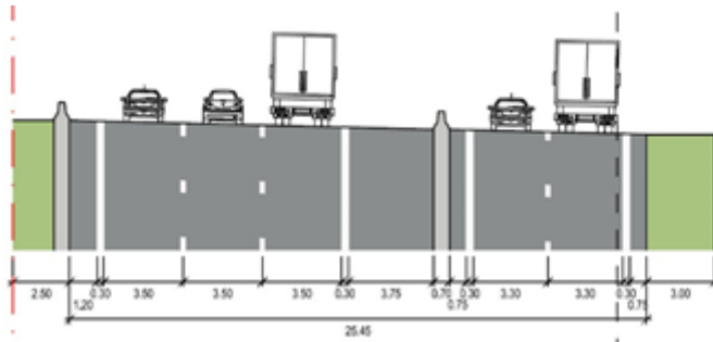
Figuur 16: Principe profiel G2 - Loop 2: met één rijvlak en fysieke scheiding tussen DRW en SRW
