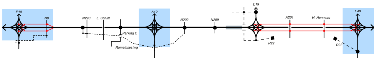
Figuur 150: Lijnschema alternatief 3 a Loop 2 – G1a/G1a/G2a'
