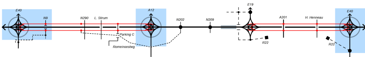
figuur 113: Lijnschema alternatief 2 met symmetrische 4/4 knopen op SRW en DRW (G2a)
