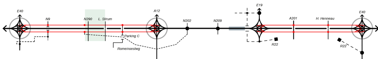
Figuur 148: Lijnschema alternatief 2 Loop 2 – G2a met LPb-WM-1
