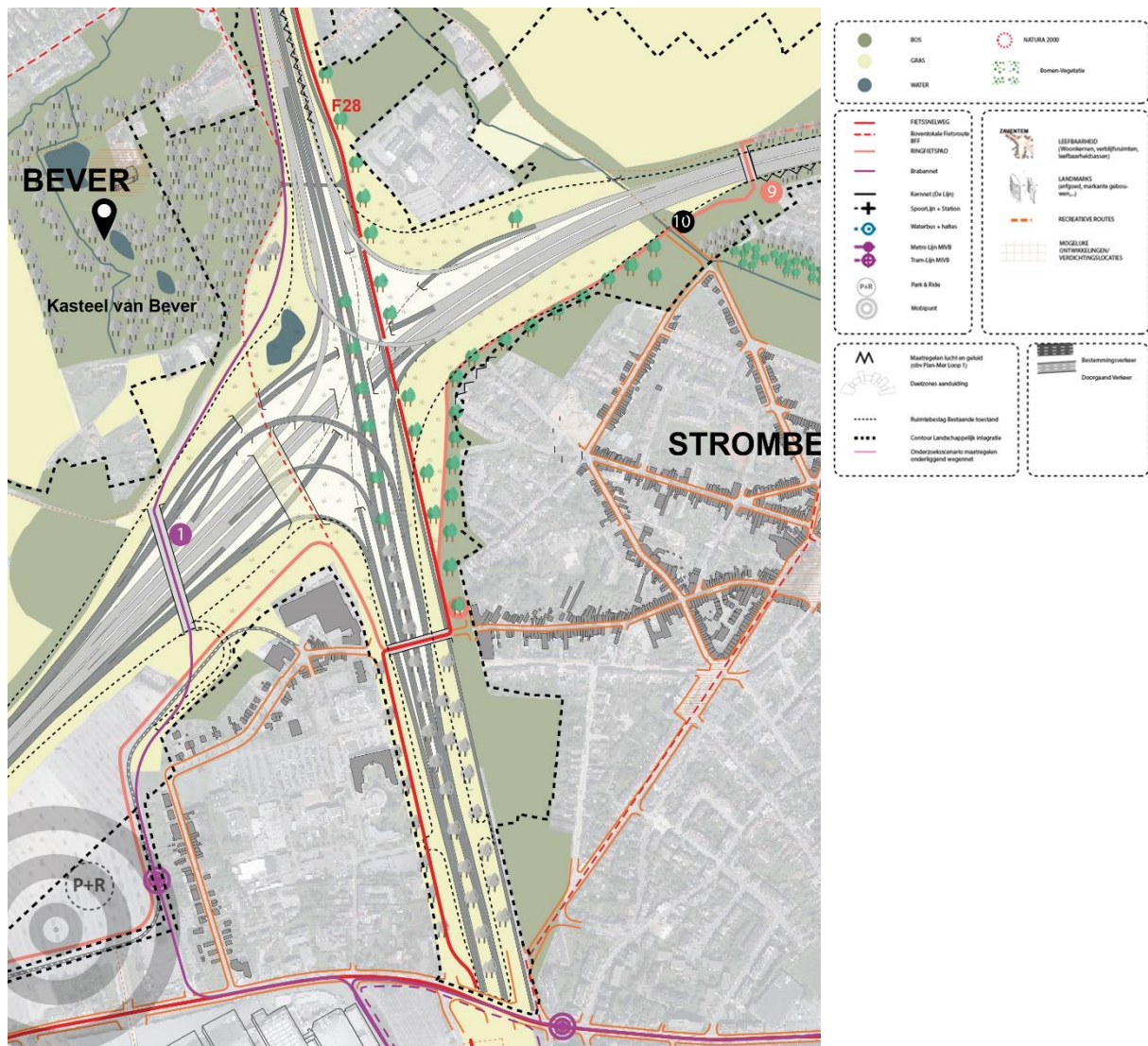
Figuur 119: Verkeerswisselaar R0/A12 Strombeek-Bever variant G2a (Loop 2)
