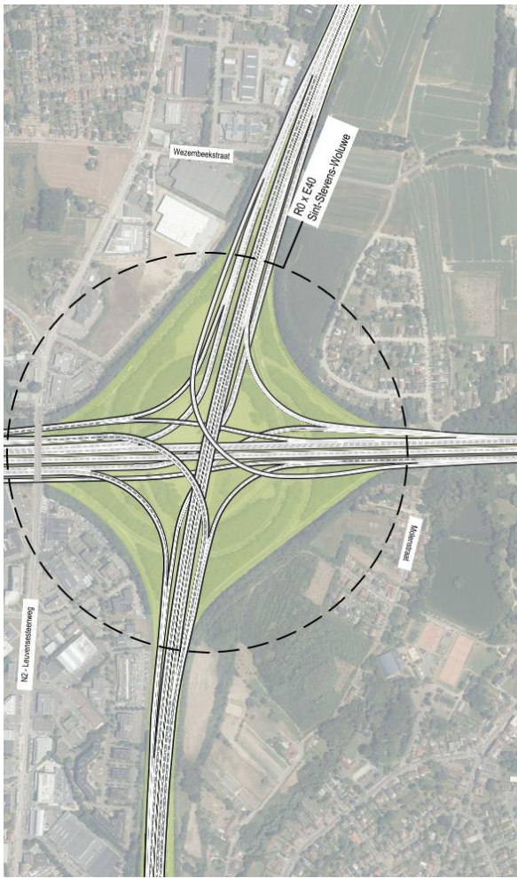
Figuur 69: VW R0/E40 Sint-Stevens-Woluwe variant a in G2 – Loop 2 → 4/4 sterknop SRW en DRW
