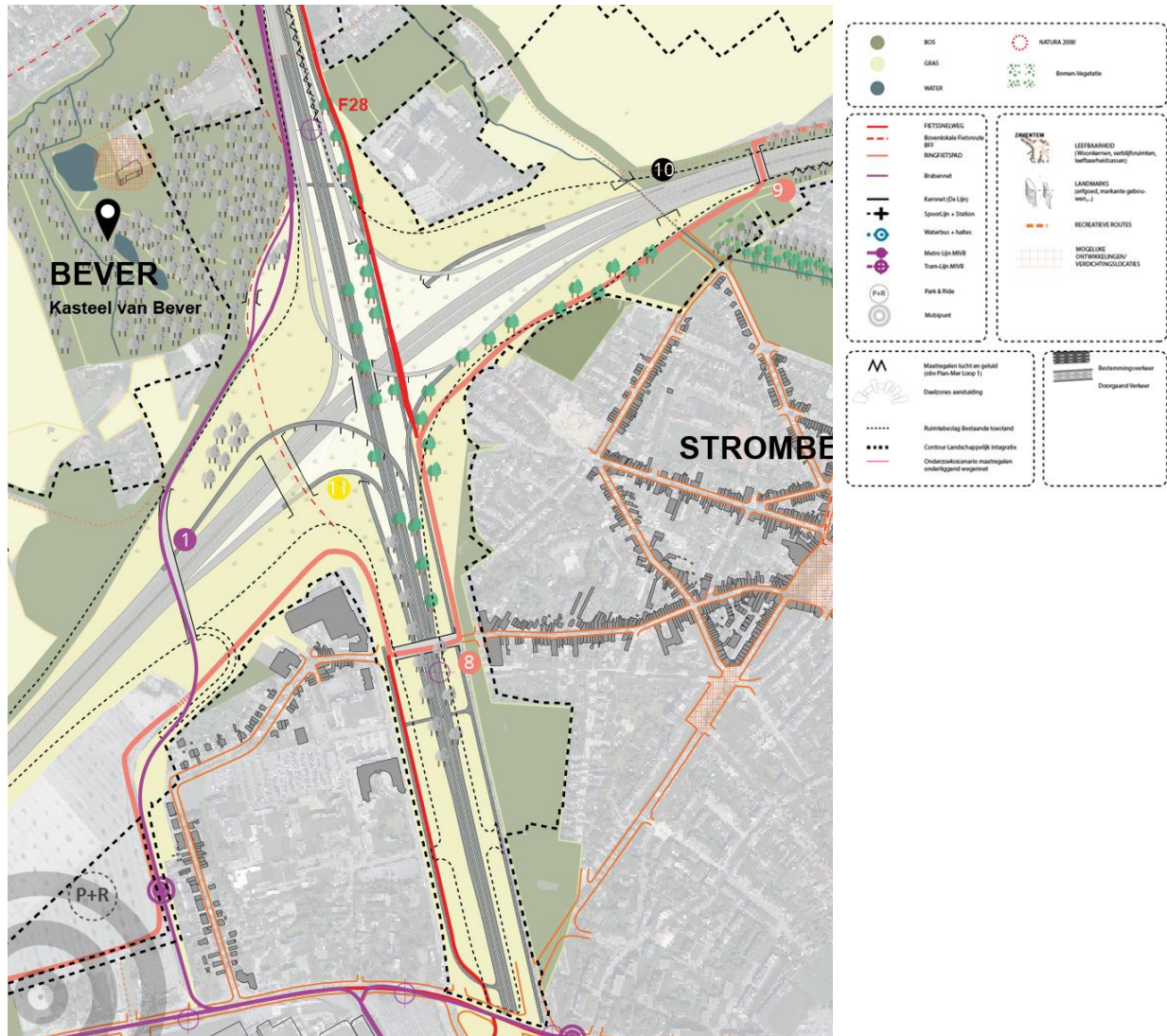
Figuur 109: Verkeerswisselaar R0/A12 Strombeek-Bever variant G1a (Loop 2)
