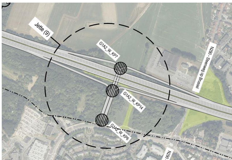
Figuur 73: Aansluitingscomplex 9 Jette/N290 in G1 – Loop 2
