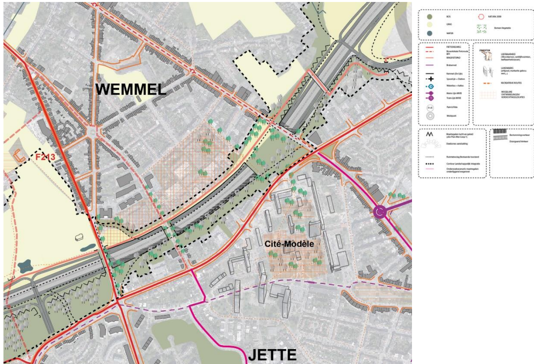
Figuur 128: Verlaagd lengteprofiel b met overbrugging van de R0-Noord (LPb_WM1) deelzone Wemmel-Jette (illustratie voor alternatief 2)
