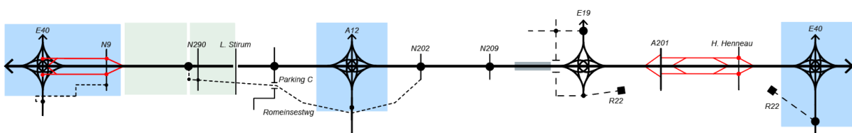
Figuur 103: Lijnschema alternatief 1 met variabele elementen
