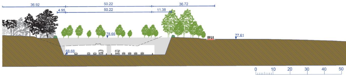
Figuur 26: Dwarsprofiel BB - G1 LPa_LB
