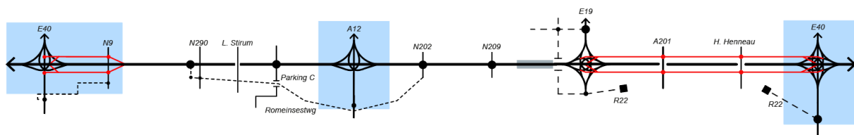
Figuur 151: Lijnschema alternatief 3 ba Loop 2 – G1b/G1b/G2a'
