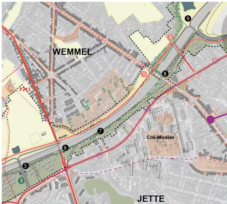
Figuur 35: Ruimtelijke uitwerking geoptimaliseerd lengteprofiel a met onderdoorgangen zone Wemmel-Jette – Loop 2 (LPa_WM)
