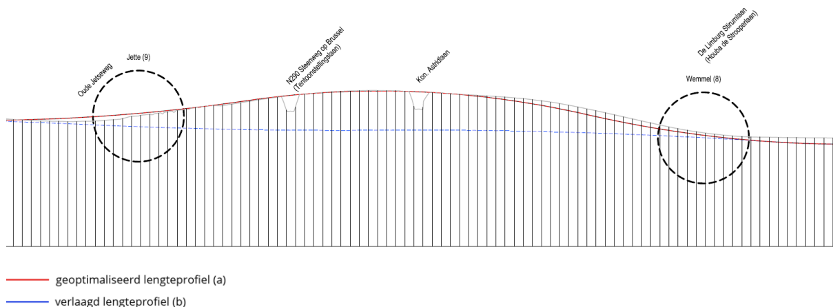
Figuur 33: Onderzoek lengteprofiel deelzone Wemmel-Jette (lengteprofiel 5x verschaald is t.o.v. hoogte (Y-as))
