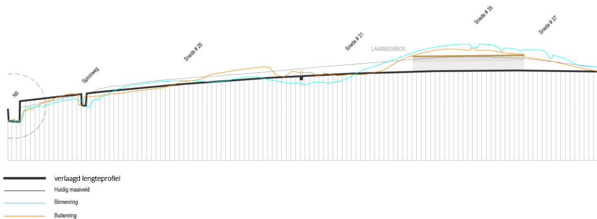
Figuur 27: Verlaagd lengteprofiel met één maximale landschapsbrug (Loop 2) (lengteprofiel 5x verschaald t.o.v. hoogte Y-as)
