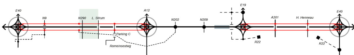
Figuur 149: Lijnschema alternatief 2 Loop 2 – G2a met LPb-WM-2
