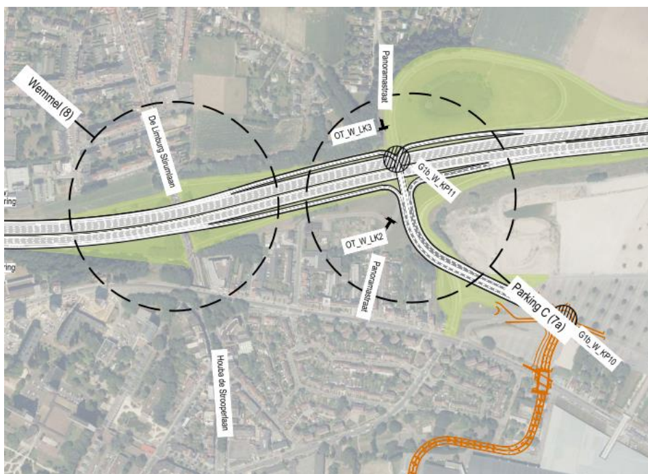
Figuur 75: Aansluitingscomplex 7a – Parking C in G1 – Loop 2 (oranje is referentietoestand)
