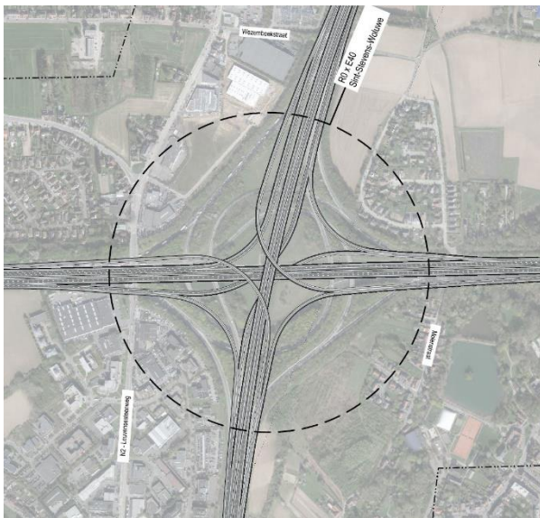
Figuur 56: Verkeerswisselaar/ knoop E40 Sint-Stevens-Woluwe in G1A2 – Loop 1 met een 4/4 knoop
