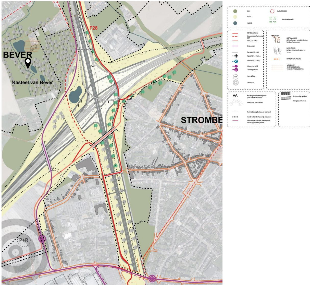
Figuur 121: Verkeerswisselaar R0/A12 Strombeek-Bever variant G2b (Loop 2)
