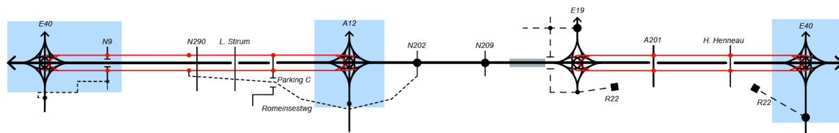
Figuur 114: Lijnschema alternatief 2 met symmetrische 4/4 knopen op SRW (G2a')
