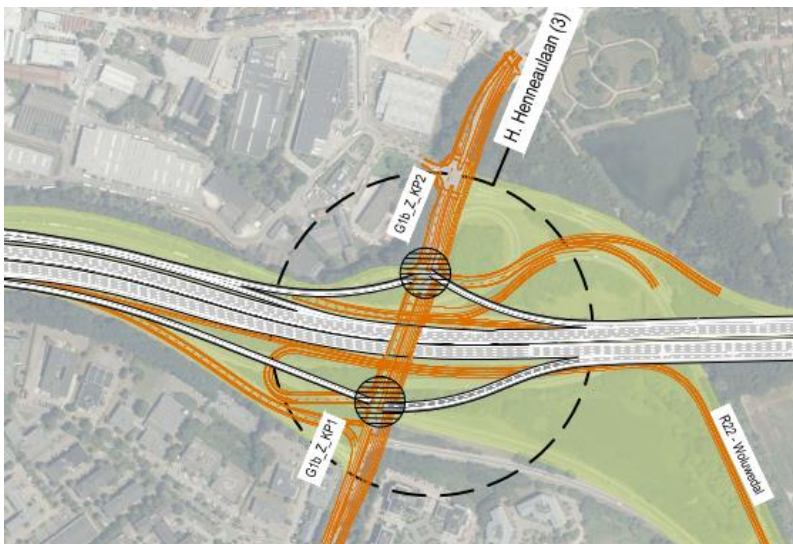
Figuur 80: Aansluitingscomplex 3– H. Henneaulaan in G1 – Loop 2 (oranje is referentietoestand)
