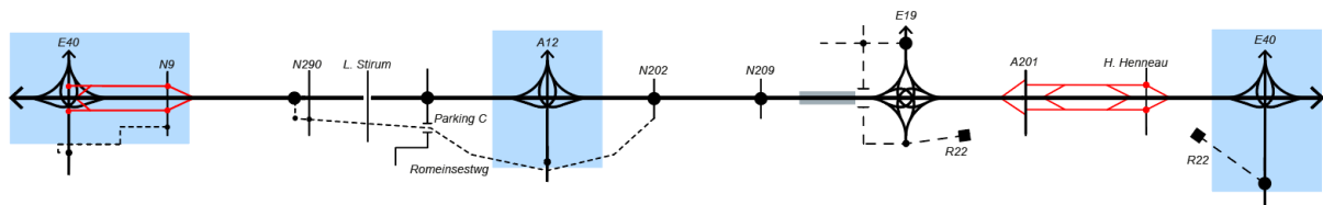
Figuur 106: Lijnschema alternatief 1 met asymmetrische 3/4 knoopen (G1b)
