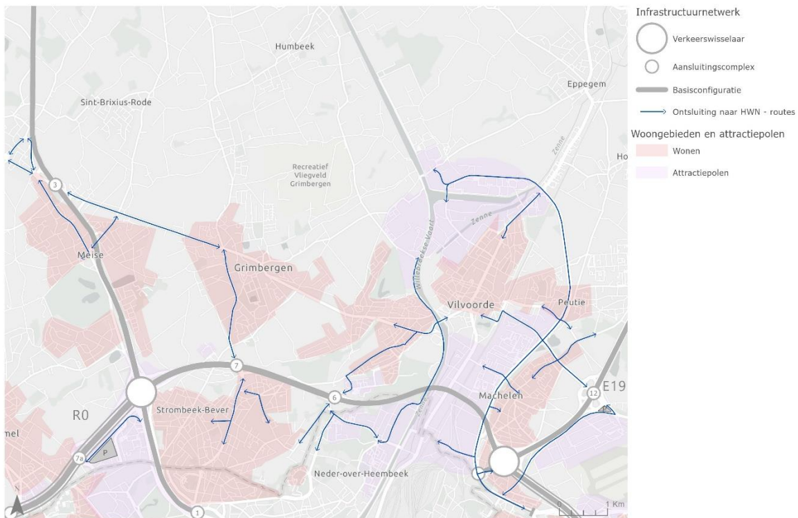
Figuur 99: Schematische weergave ontsluitingsstructuur zone Vilvoorde (G2a)
