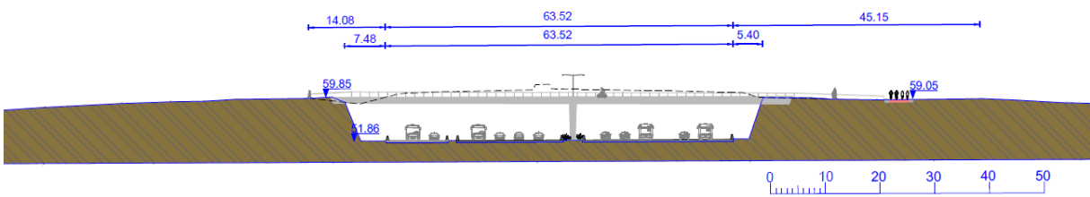
Figuur 24: dwarsprofiel AA – G1 LPa_LB
