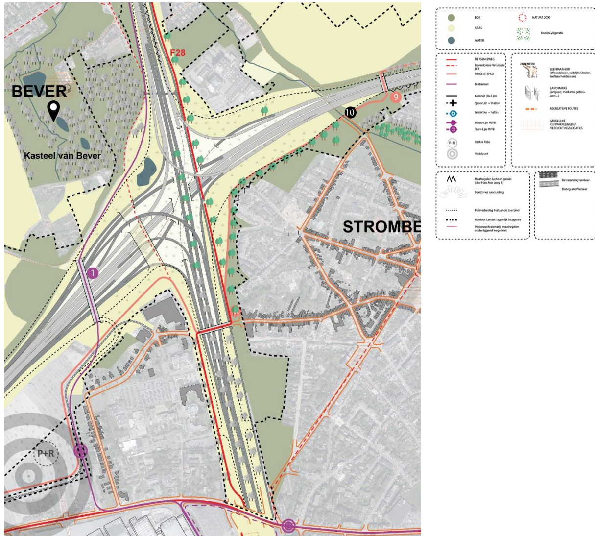
Figuur 120: Verkeerswisselaar R0/A12 Strombeek-Bever variant G2a' (Loop 2)
