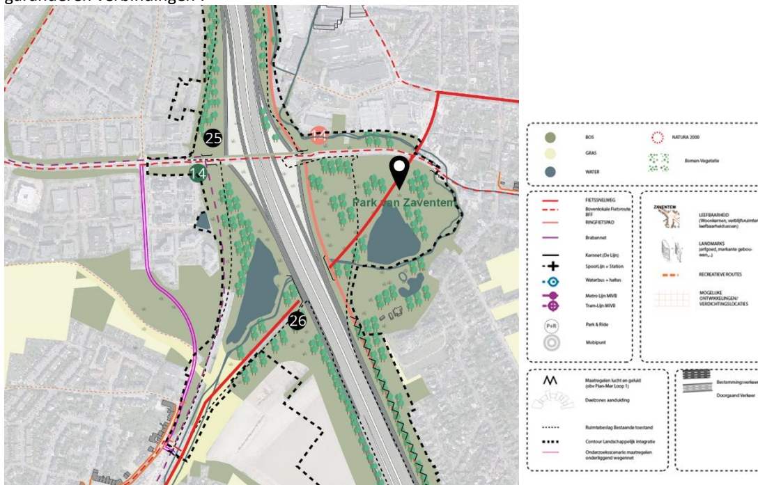
Figuur 43: Ruimtelijke uitwerking aansluitingscomplex H. Henneaulaan Loop 2 - landschappelijke verbinding ter hoogte van Woluwevallei (zone Zaventem)
