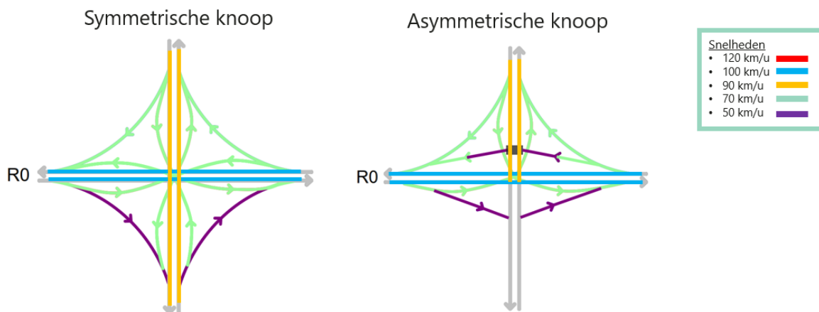
Figuur 47: principiële weergave snelheidsregime in de knopen – toeleidende radiale snelwegen zijn verder te harmoniseren (grijs)
