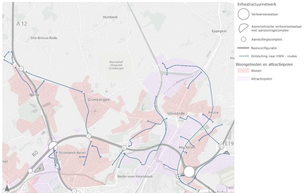
Figuur 98: Schematische weergave ontsluitingsstructuur zone Vilvoorde (G1a, G1b, G2a', G2b)
