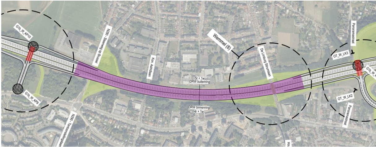
Figuur 38: Tunnelvoorschriften rijkwaterstraat toegepast op deelzone Wommel-Jette (paarse zone) (referentie R1)
