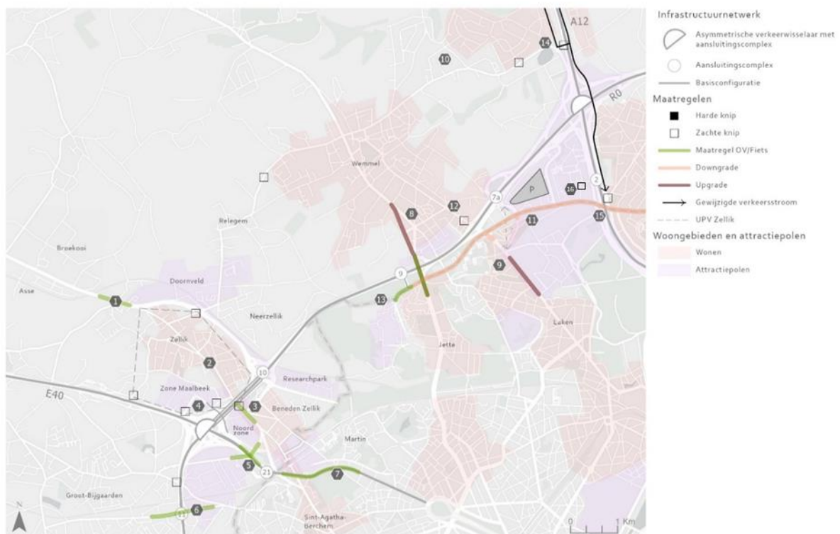
Figuur 135: Zone Wemmel -aanduiding maatregelen onderliggend wegennet
