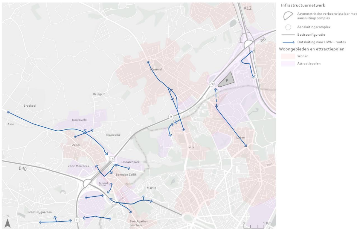
Figuur 96: Schematische weergave ontsluitingsstructuur zone Wommel (G1a, G1b, G2a', G2b – zijnde de alternatief 1 en alternatief 2 (behalve G2a))
