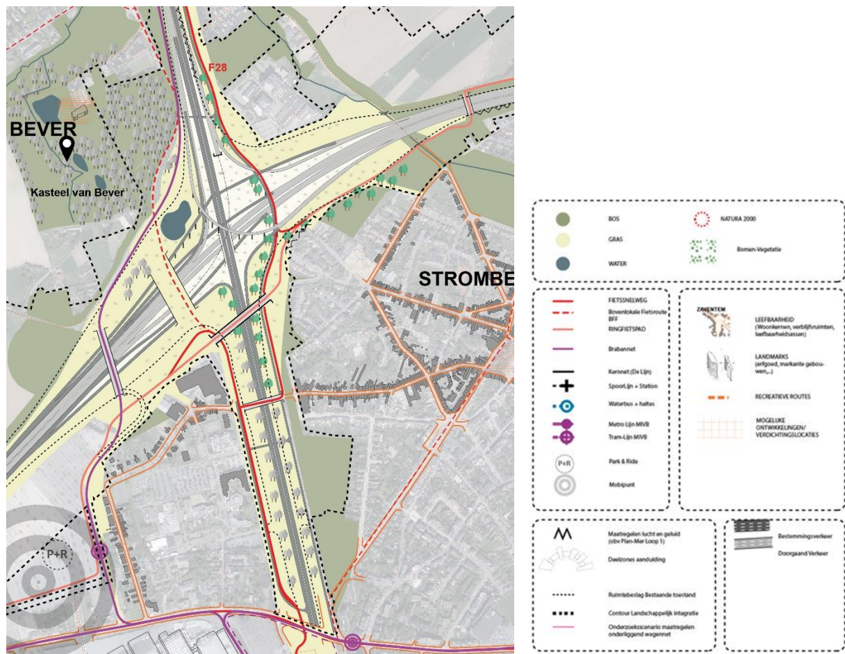
Figuur 41: Ruimtelijke uitwerking A12-knoop Loop 2 – landschapsbrug ten westen van de knoop (G2b)
