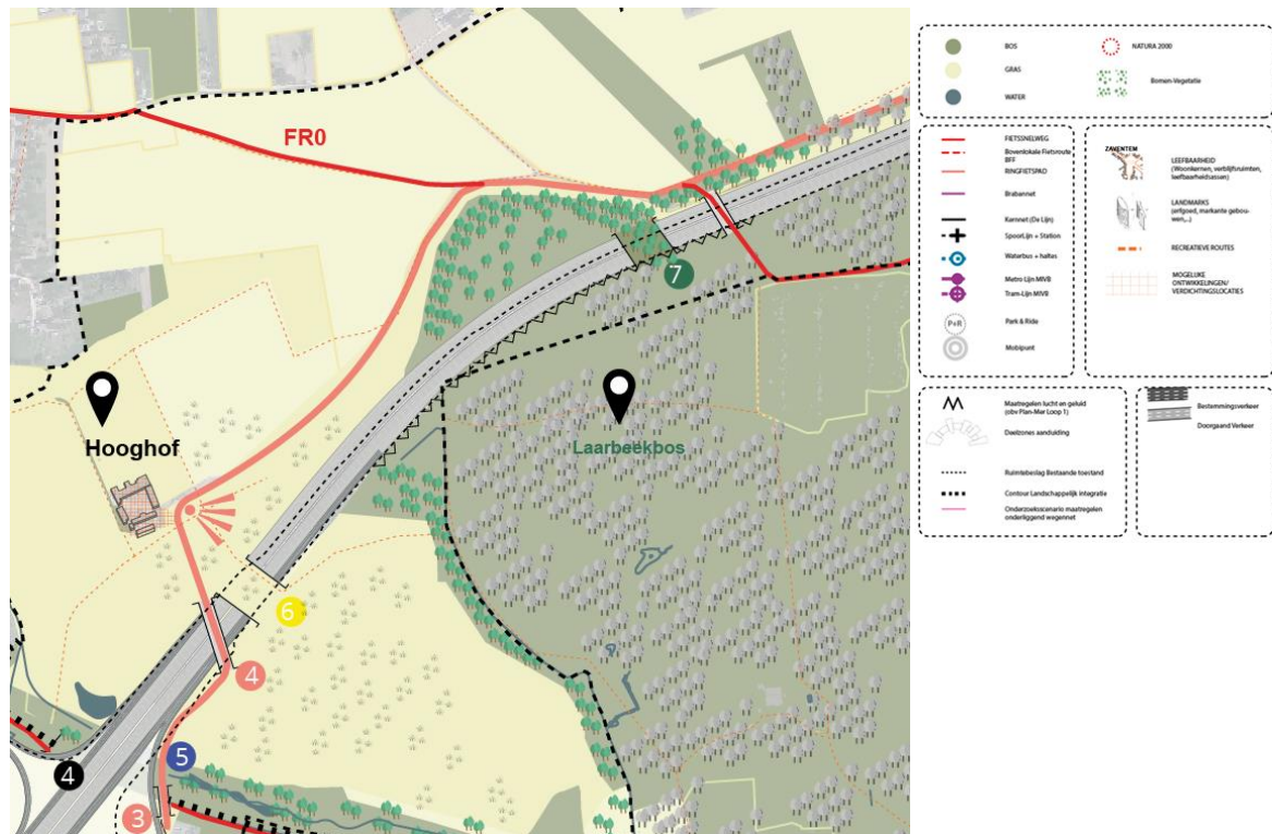
Figuur 125: Geoptimaliseerd lengteprofiel a met twee landschapsbruggen (LPa LB) deelzone Laarbeekbos (illustratie voor alternatief 1)
