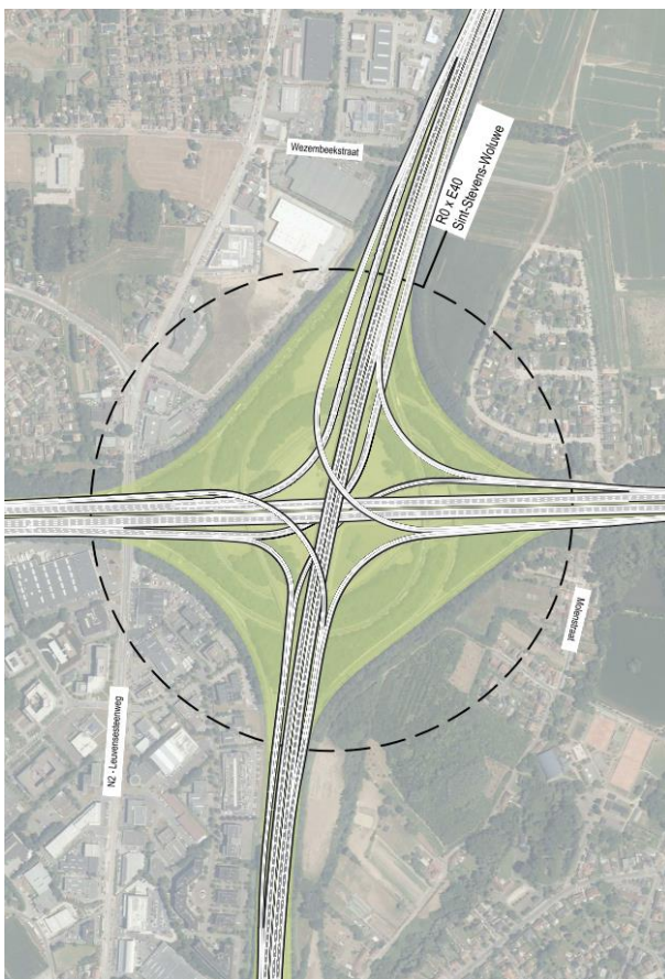
Figuur 57: Verkeerswisselaar/ knoop E40 Sint-Stevens-Woluwe variant a in G1 – Loop 2 → 4/4 sterknop
