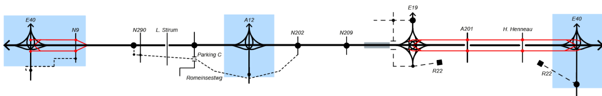
Figuur 152: Lijnschema alternatief 3 b Loop 2 – G1b/G1b/G2b
