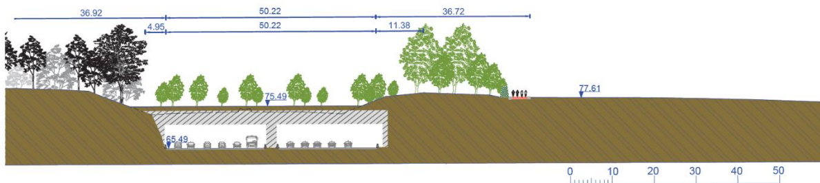
Figuur 32: Dwarsprofiel B- G1 LPb_LB
