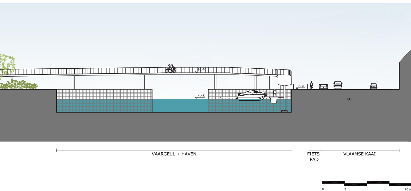
Snede 1 - opwaarts van spoorbrug
