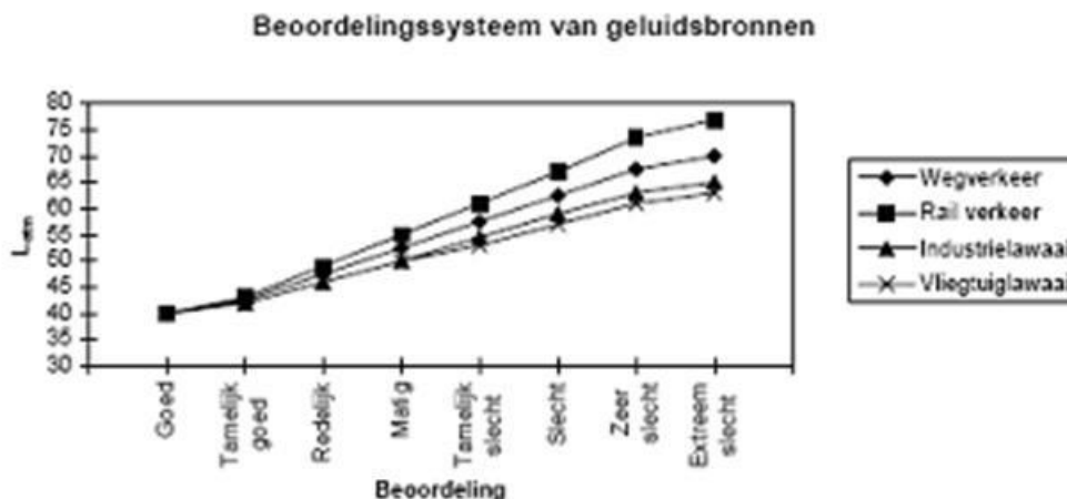
Figuur 7-54 Beoordeling van geluidsbronnen
