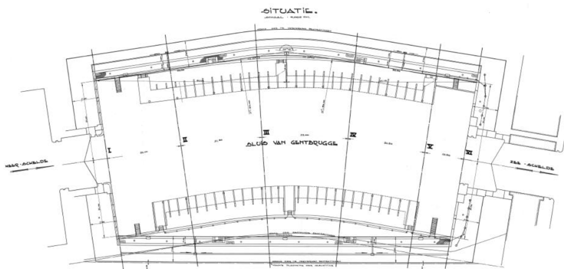
Figuur 7-81 Grondplan van de sluis voor de aanpassingen (opmeting 1979)
