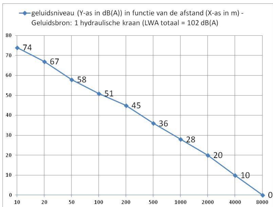
Figuur 7-53 Maximaal te verwachten geluidsniveaus tijdens de baggerwerken
