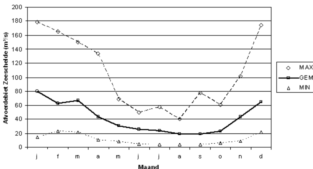
Figuur 7-16 Afvoerdebiet Zeeschelde te Melle (op maandbasis, 1987-2005) (Bron: Waterbouwkundig Labo)
