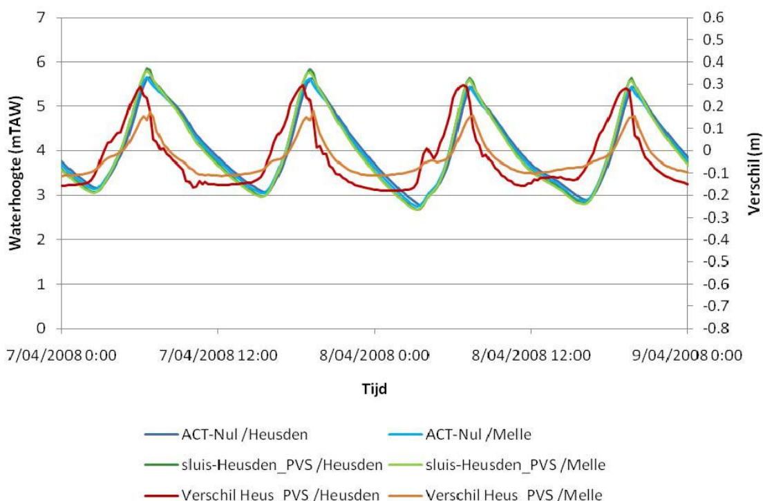
Figuur 7-29 Waterpeilen ter hoogte van Heusden en Melle voor de actuele situatie en voor het scenario met de sluis ter hoogte van Heusden en profiel "passagiersvaart-scenario" gecombineerd met de waterpeilverschillen tussen de 2 situaties, voor 2 dagen begin april 2008
