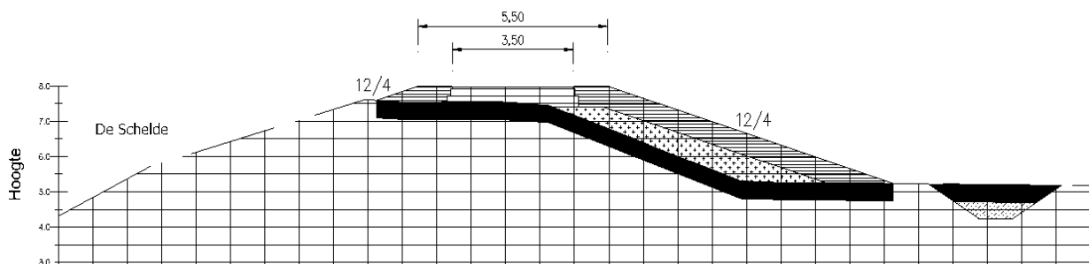
Figuur 5-6 Typeprofiel ophoging dijken tot Sigmahoogte
