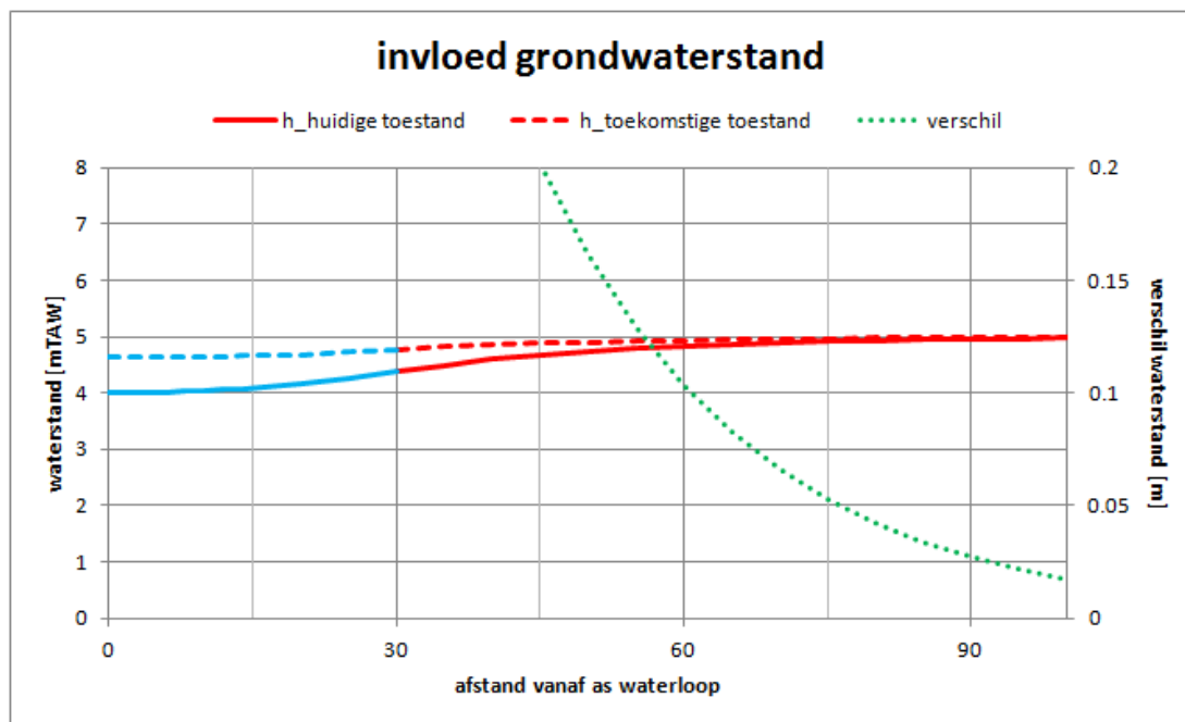
Figuur 7-40 Wijziging grondwaterstand ten opzichte van de afstand tot de as van de Schelde in het planalternatief (doorlatendheid 1 m/d)
