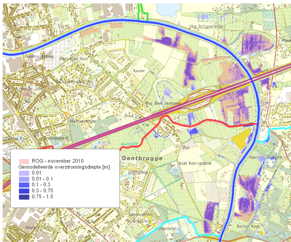
Figuur 7-18 Vergelijking ROG 2010 – modelresultaten
