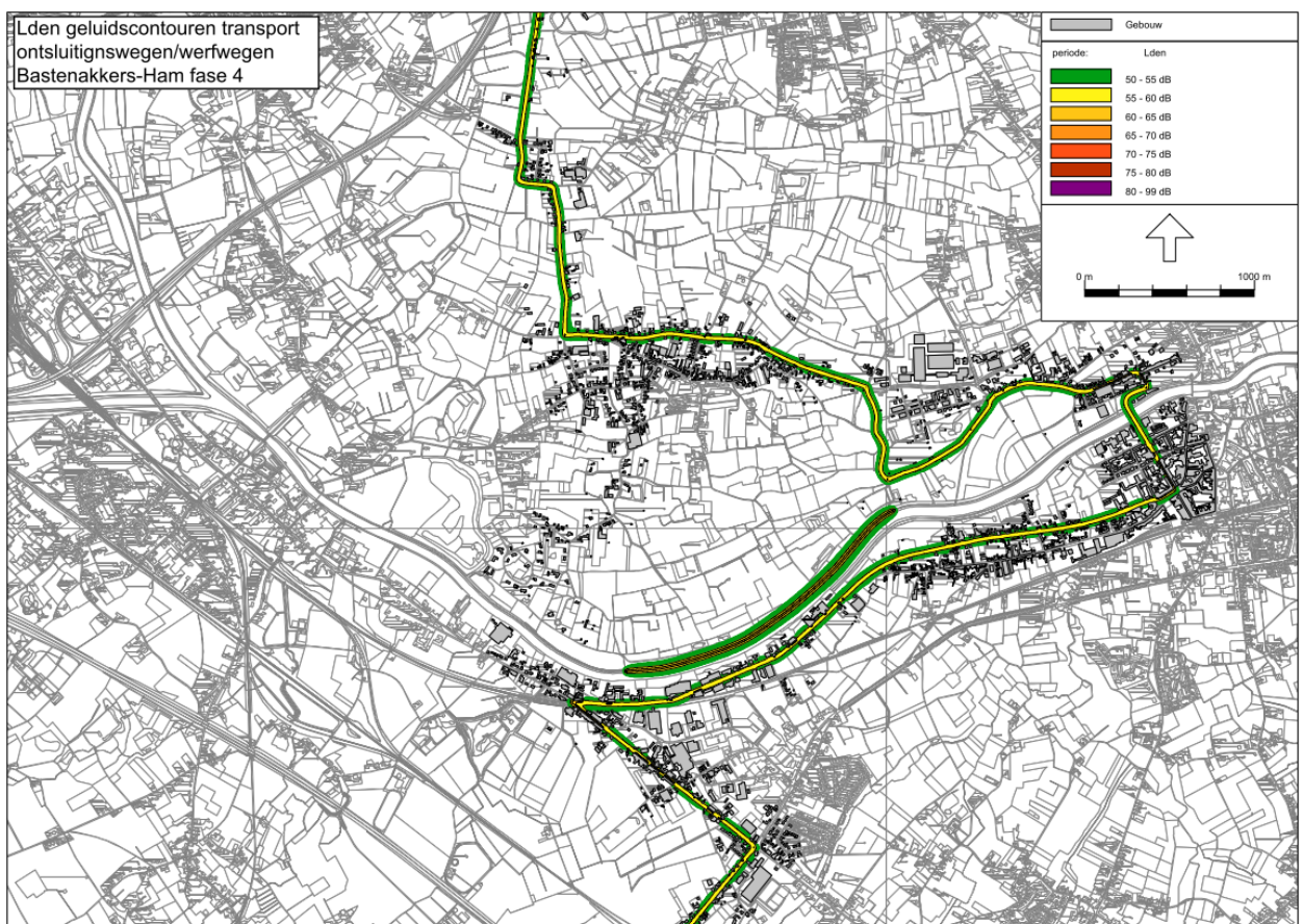
Figuur 7-50 Geluidscontouren voor het transport langs werfwegen en ontsluitingswegen
