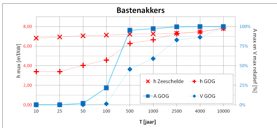
Figuur 7-37 Verwachte maximale waterstanden en percentage relatief overstroomt oppervlakte (A) en volume (V) binnen GOG Bastenakkers volgens verschillende retourperioden
