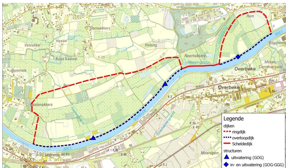
Figuur 4-11 Situering ringdijken en overlooptdijken Bastenakkers-Ham (variant 1 zie §5.3.3)
