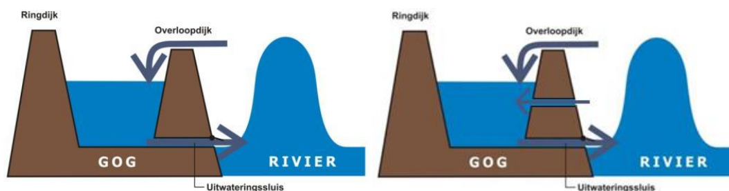
Figuur 4-12 Werkingsprincipe GOG (links) en GOG-GGG (rechts)
