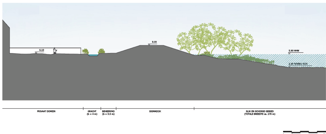
Figuur 4-3 Situering ringdijk en getijdennatuur voormalige zandwinningsput Melle
