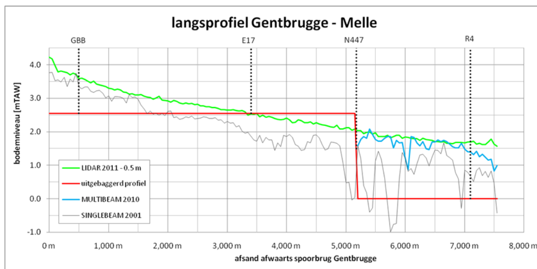
Figuur 4-7 Bestaand (groen, blauw en grijze lijn) en toekomstig langsprofiel (rode lijn) van de Zeeschelde tussen Gentbrugge en Melle
