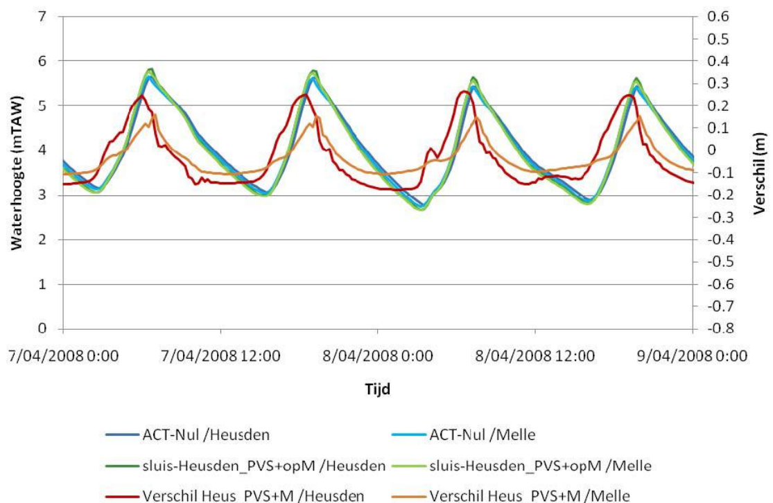
Figuur 7-31 Waterpeilen ter hoogte van Heusden en Melle voor de actuele situatie en voor het scenario met de sluis ter hoogte van Heusden en profiel “passagiersvaart-scenario” en de ontpoldering in Melle gecombineerd met de waterpeilverschillen tussen de 2 situaties, voor 2 dagen begin april 2008
