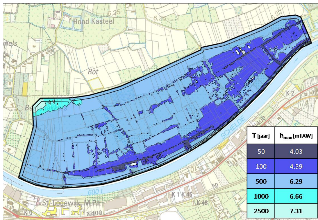
Figuur 4-20 Overstroomde gebieden binnen GOG Bastenakkers volgens verschillende retourperioden (variant 2, zie §5.3.3)
