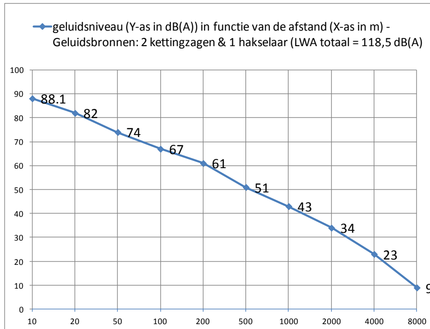
Figuur 7-51 Maximaal te verwachten geluidsniveaus tijdens rooiwerken
