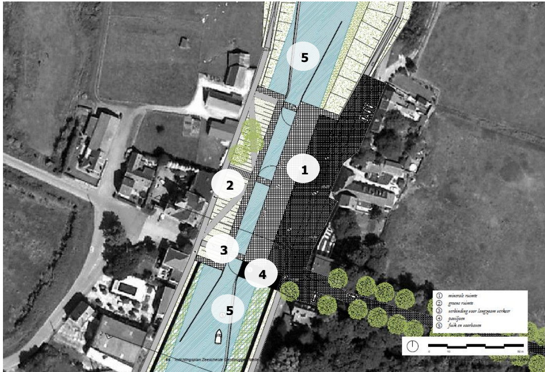
Figuur 4-16 Inrichtingsplan sluis in Heusden
