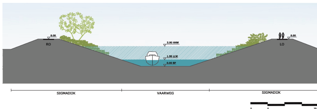
Figuur 7-74 Inrichtingsplan voor Zeeschelde tussen nieuwe sluis te Heusden en Melle (Ringvaart)
