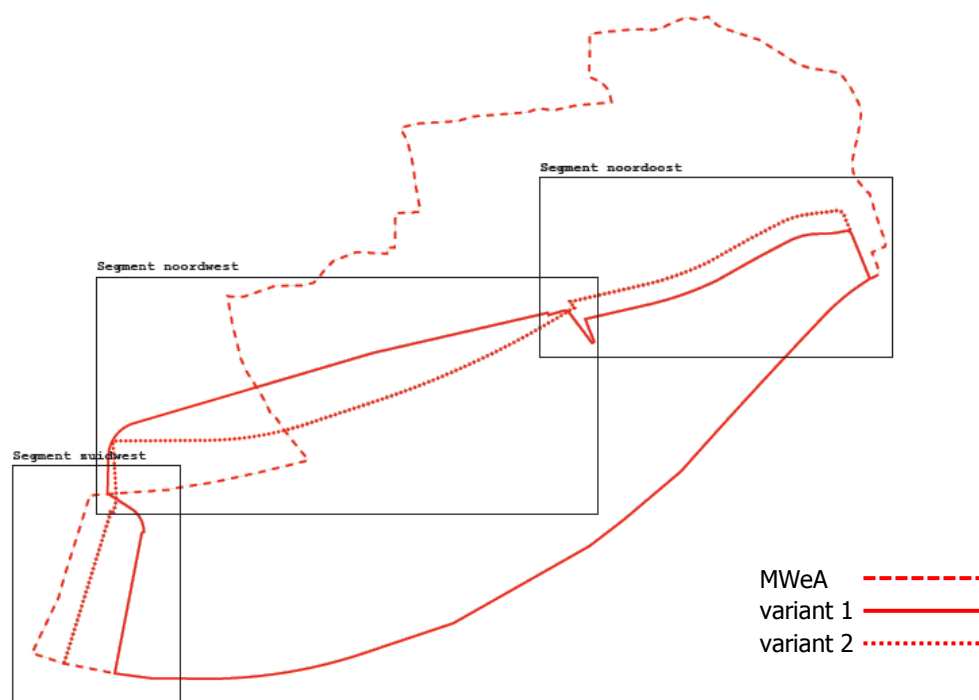
Figuur 5-5 Uitvoeringsvarianten tracé ringdijk GOG Bastenakkers (MWeA ter referentie)
