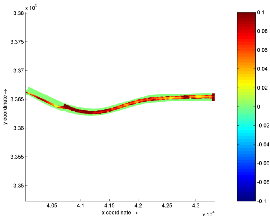
Figuur 7-44 Sedimentatie/erosie (m/jaar na 1 jaar simulatie) in Ringvaart in huidige toestand (boven) en bij sluis incl. baggeren (onder), wanneer gestart wordt met geen beschikbaar sediment op de bodem van de Ringvaart
