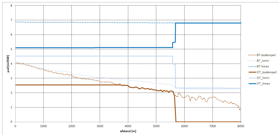
Figuur 7-35 Langsprofiel van ZGM met minimaal en maximaal waterpeil voor de overstromingsgebeurtenis van november 2010. Vergelijking huidige toestand (BT) en geplande situatie, met sluis (OT)
