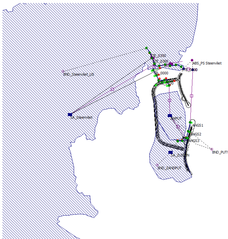
Figuur 7-27 Modelschematisatie afwatering omgeving voormalige zandput.
