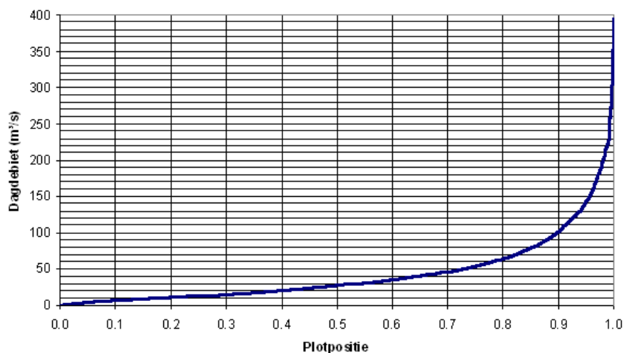
Figuur 7-15 Percentielwaarden voor de afvoer op de Zeeschelde te Melle (1987-2005)(Bron: Waterbouwkundig Labo)
