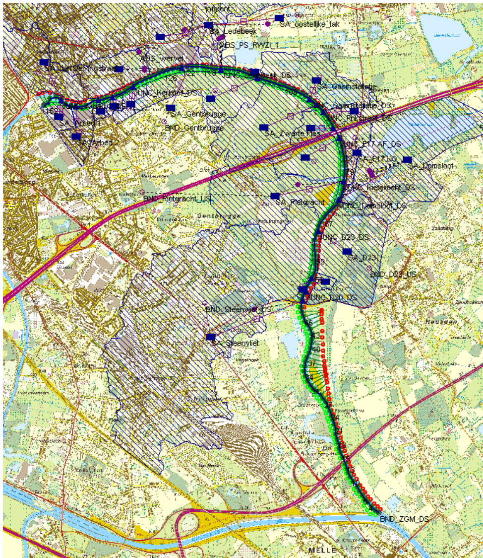
Figuur 7-26 Model Scheldemeander Gentbrugge – Melle.
