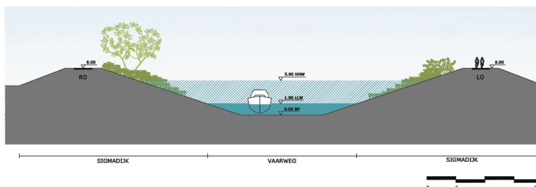
Figuur 8-19 Inrichtingsplan voor Zeeschelde tussen nieuwe sluis te Heusden en Melle (Ringvaart)
