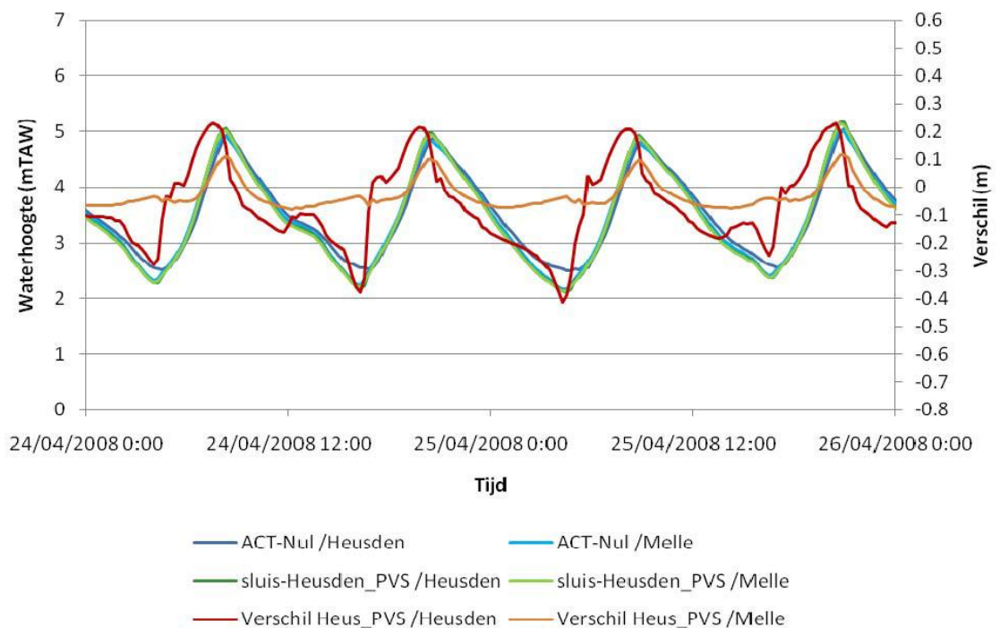
Figuur 7-30 Waterpeilen ter hoogte van Heusden en Melle voor de actuele situatie en voor het scenario met de sluis ter hoogte van Heusden en profiel “passagiersvaart-scenario” gecombineerd met de waterpeilverschillen tussen de 2 situaties, voor 2 dagen eind april 2008
