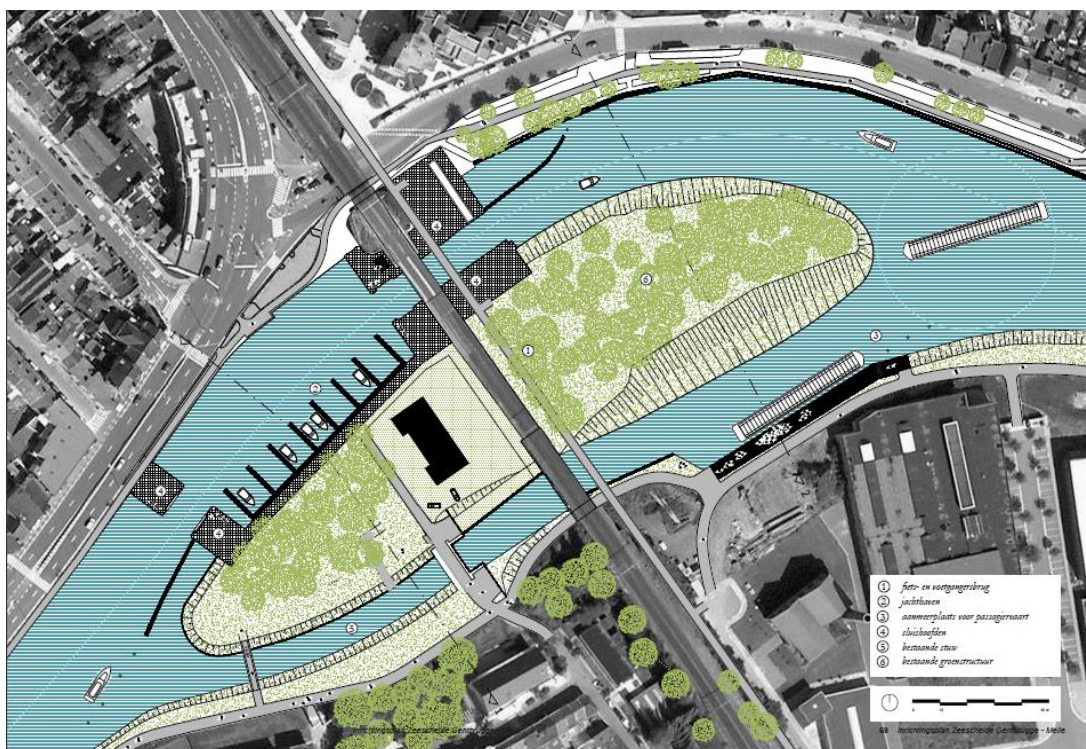
Figuur 8-15 Inrichtingsplan voor de omgeving van de Callenssluis in Gentbrugge
