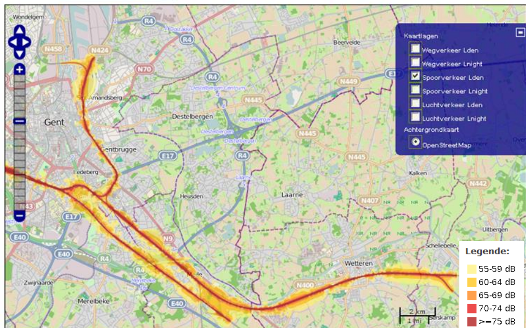
Figuur 7-47 Spoorverkeerslawaai – geluidsindicator Lden (bron LNE: printscreen viewer 'goedgekeurde geluidskarten – deelgebieden: Gent en oostelijke randgebieden')
