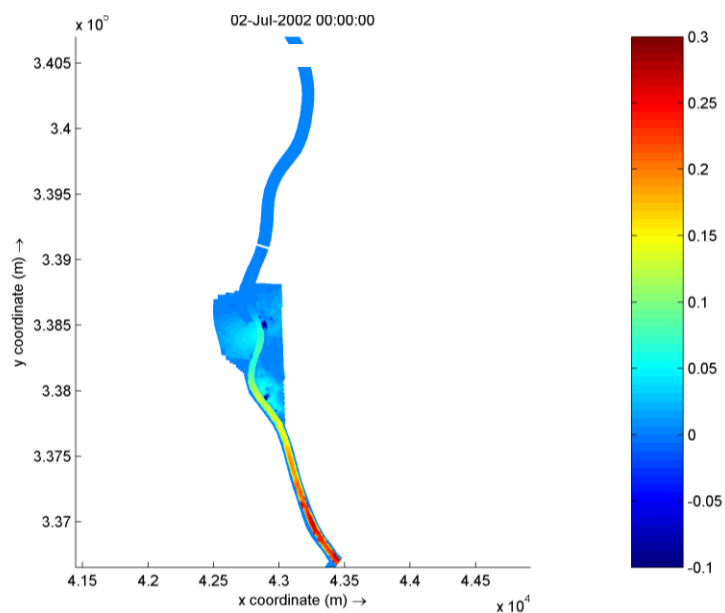
Figuur 7-43 Gemodelleerde sedimentatie/erosie in m/j in planalternatief (IMDC, 2011b). Positieve waarden zijn sedimentatie, negatieve waarden geven erosie weer.
