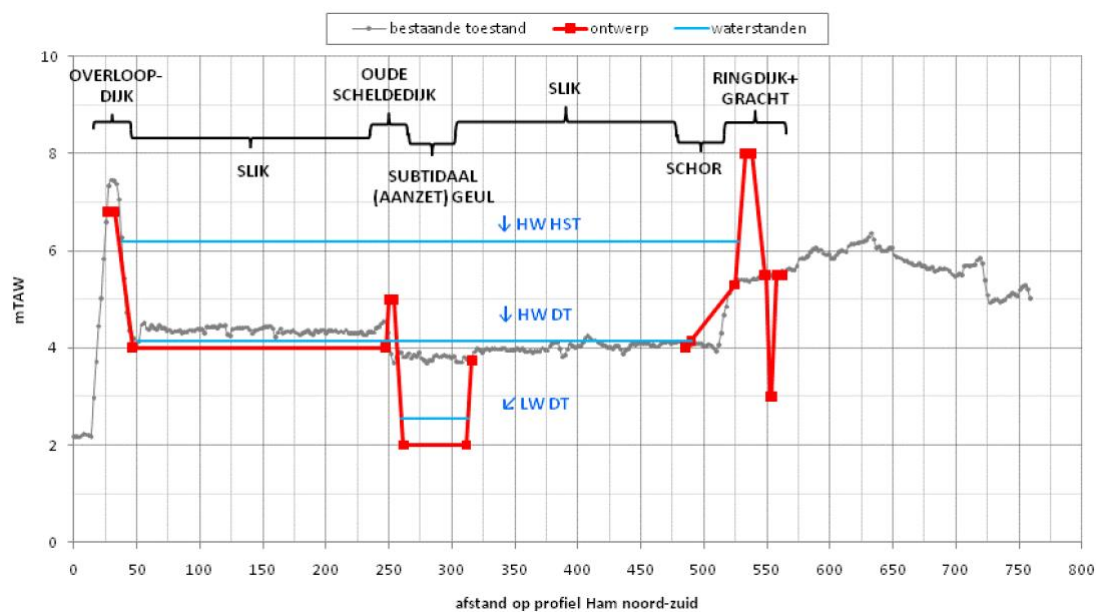
Figuur 4-23 Dwarsprofiel deelgebied Ham
