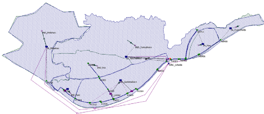
Figuur 7-28 Hydrodynamisch model Bastenakkers-Ham bestaande toestand
