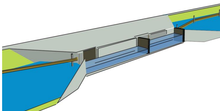
Figuur 4-8 Simulatie van een sluis met tussendeur
