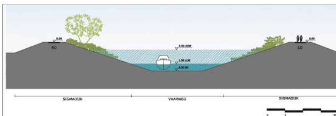
Figuur 9-11 Profielschets Zeeschelde nul+ alternatief - basis
