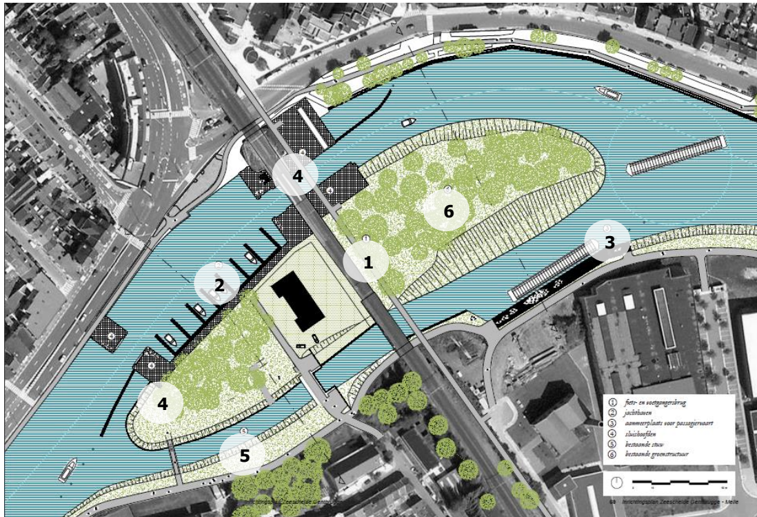
Figuur 4-15 Inrichtingsplan eiland in Gentbrugge
