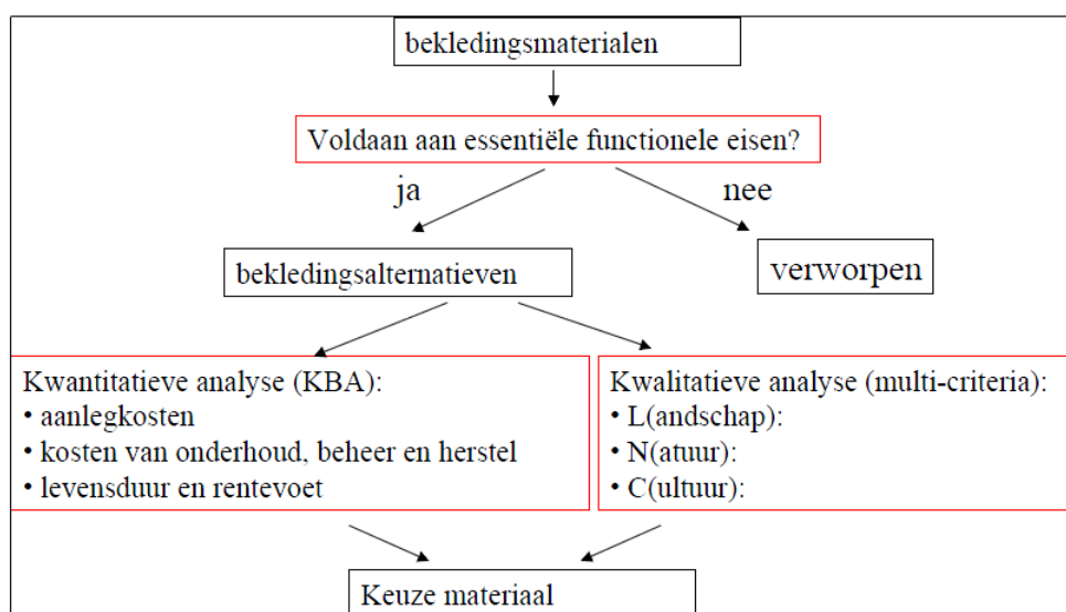
Figuur 7-12 Grafische voorstelling van de gebruikte methode voor de keuze van de dijkbekleding
