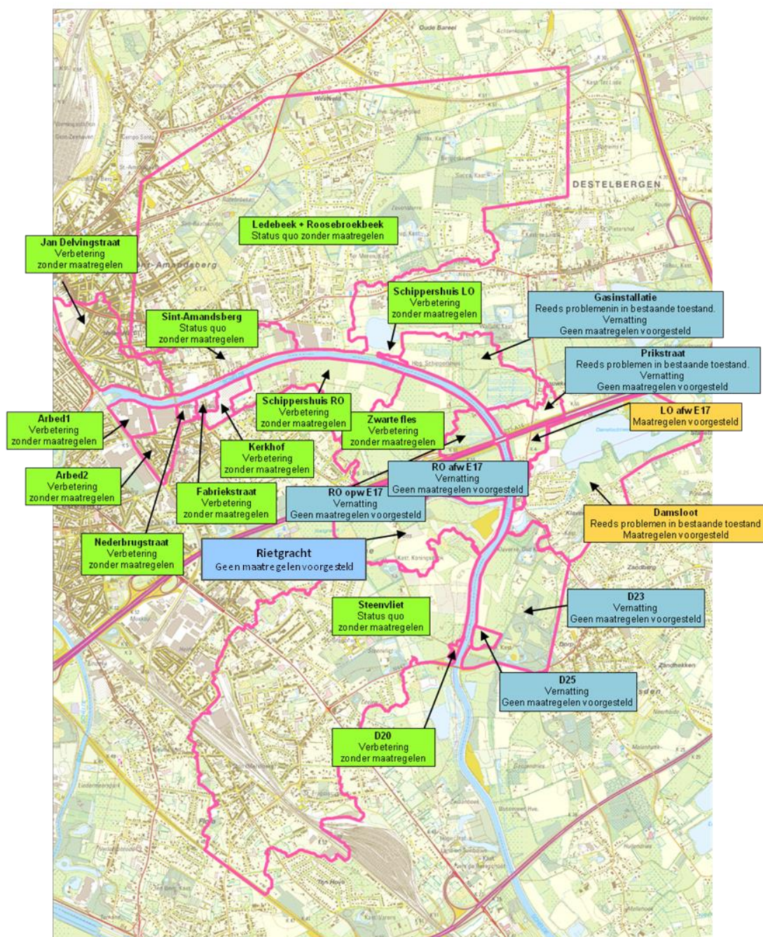
Figuur 7-36 Effecten op de afwatering van de deelgebieden ten gevolge van de sluis (zonder bijkomende maatregelen), ontwerpcriterium = geen bijkomende wateroverlast
