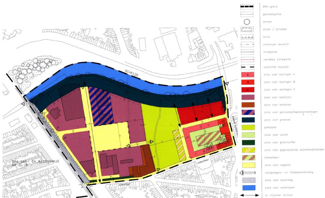
Figuur 2-4 Grafisch Plan BPA Arbed Noord
