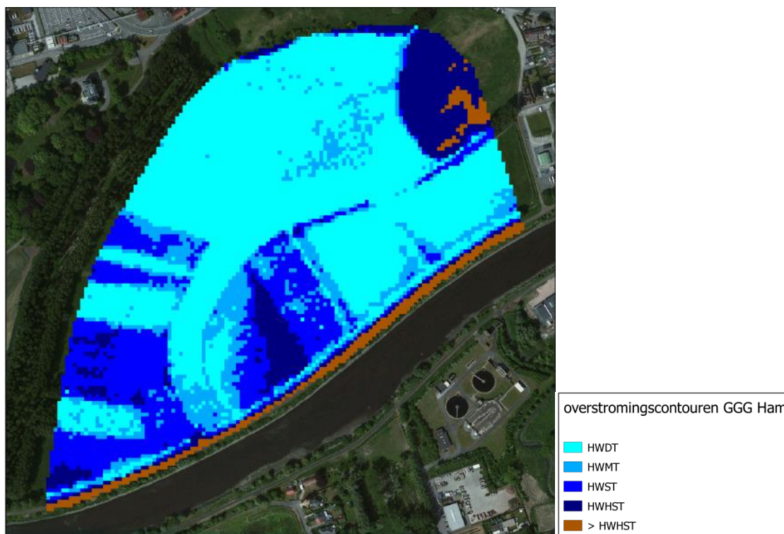
Figuur 4-22 Overstroomde gebieden binnen GOG-GGG Ham volgens verschillende retourperioden
