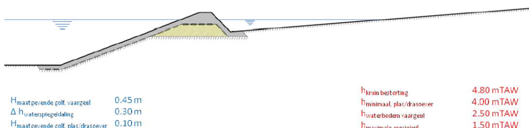
Figuur 4-5 Schematisch voorontwerp plas/dras oever met vooroeverdamm
