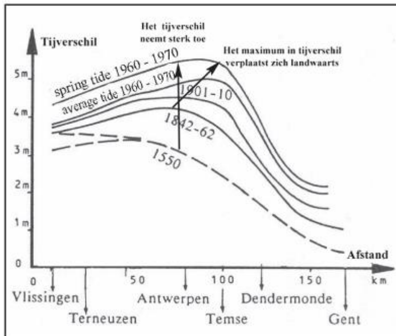
Figuur 7-17 Evolutie van het tijverschil van 1550 tot 1970. De pijlen geven aan hoe in de buurt van Antwerpen het tijverschil toeneemt en het maximum in tijverschil zich landwaarts verplaatst (bron: Coen, 1988).
