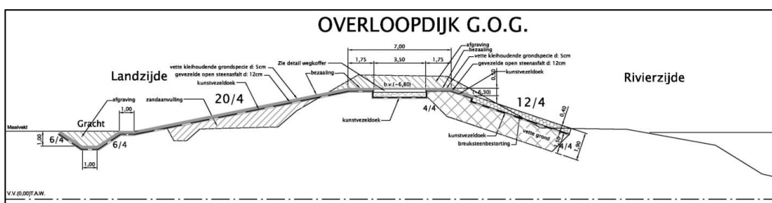
Figuur 8-23 Standaardprofiel overloopdijk van een GOG
