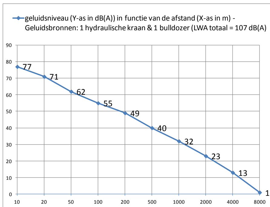
Figuur 7-52 Maximaal te verwachten geluidsniveaus tijdens grondverzetwerken
