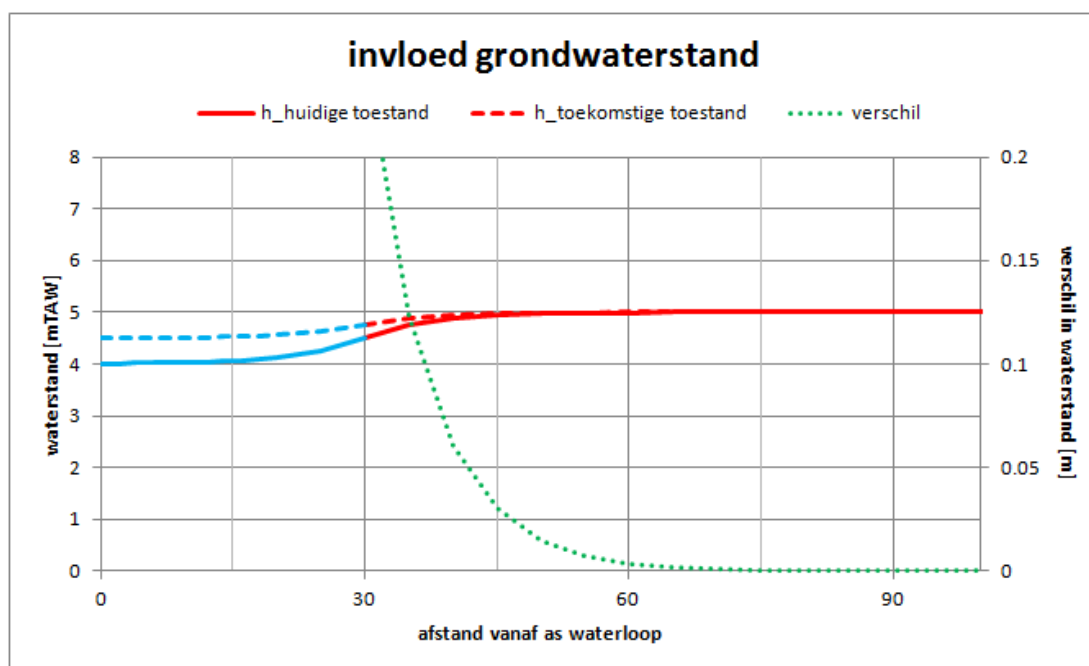
Figuur 7-41 Wijziging grondwaterstand ten opzichte van de afstand tot de as van de Schelde in het planalternatief (doorlatendheid 0,1 m/d)
