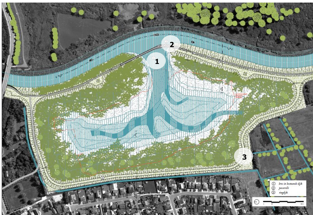
Figuur 4-17 Inrichtingsplan aangetakte voormalige zandwinningsput van Melle
