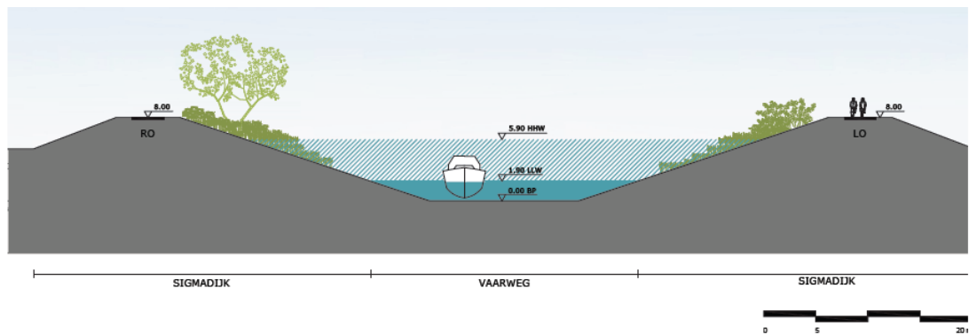
Figuur 4-2 Profiel getijafhankelijk deel Zeeschelde
