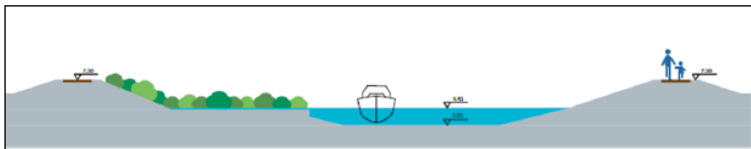
Figuur 8-17 Profiel van de Schelde stroomopwaarts de nieuwe sluis
