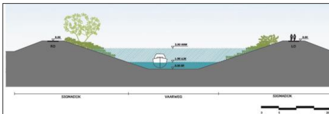
Figuur 9-13 Inrichtingsplan voor Schelde tussen Heusdenbrug en Melle (ringvaart)
