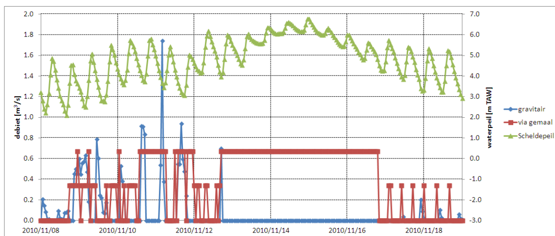
Figuur 7-23 Debietafvoer richting Schelde voor de event van november 2010
