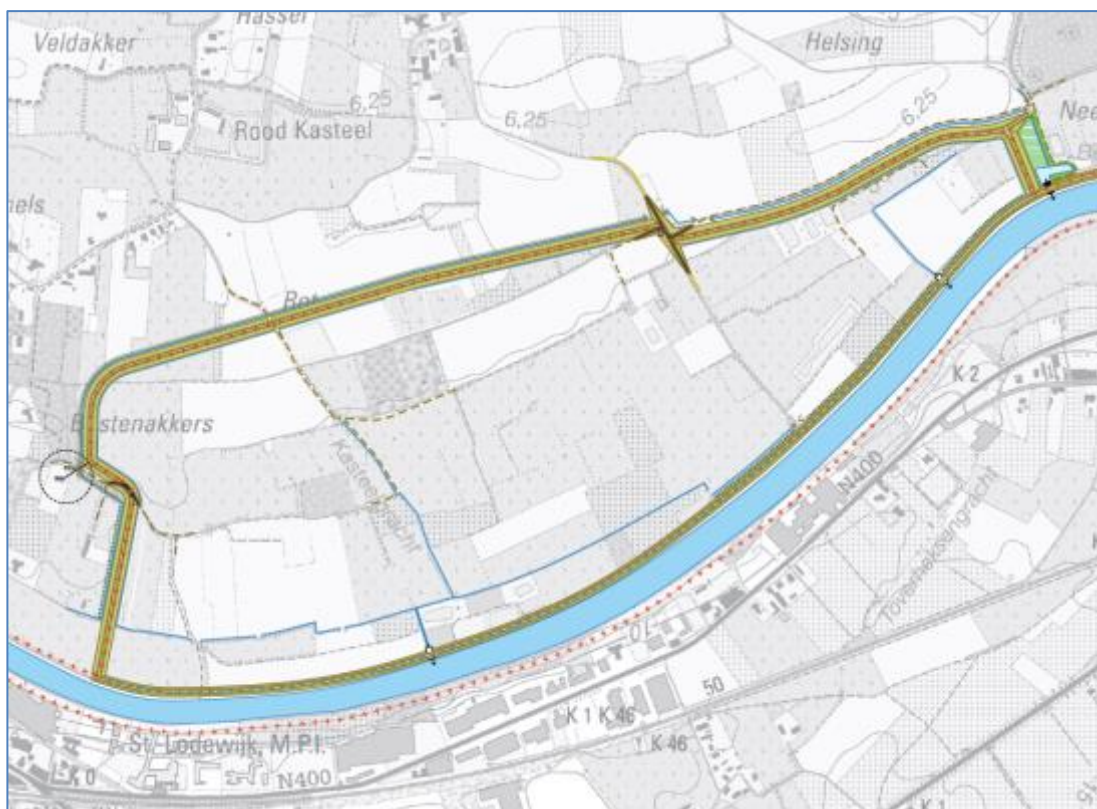
Figuur 8-22 Inrichtingsplan voor het plangebied Bastenakkers met situering kruising wegen over ringdijk
