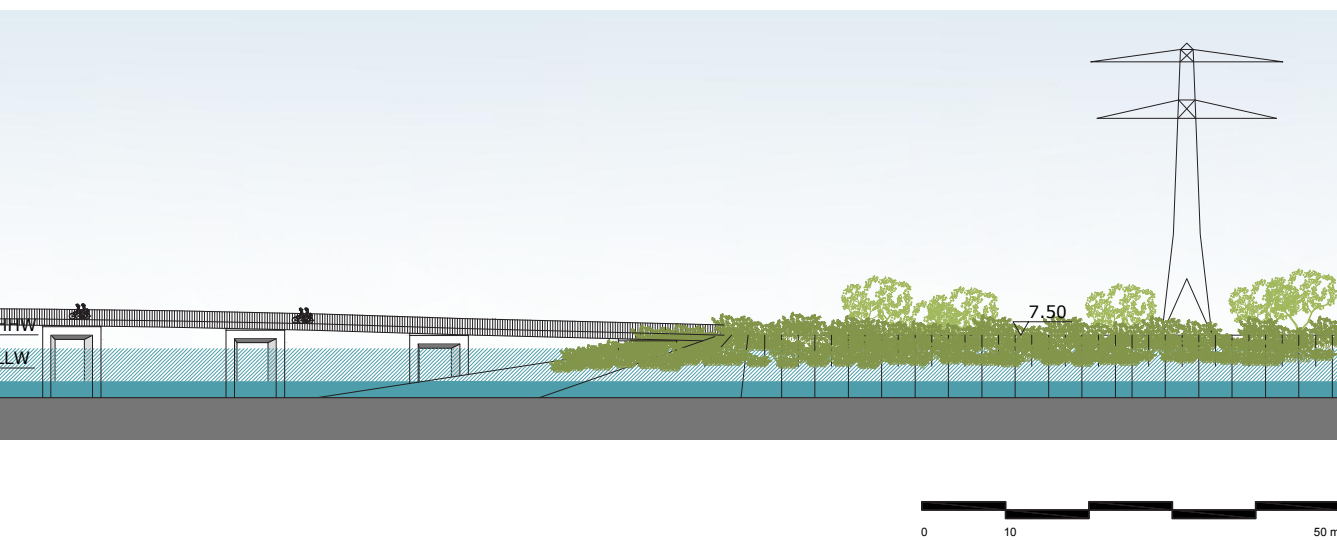
Snede 3 - aanzicht van de passerelle ter hoogte van de bres
