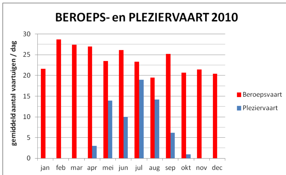
Figuur 3-1 Gemiddeld aantal beroeps- en pleziervaartuigen per dag per maand in 2010 (W&Z, 2013)
