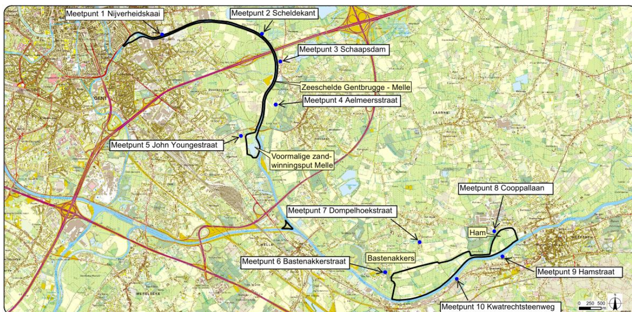
Figuur 7-49 Aanduiding ambulante meetpunten (topokaart)
