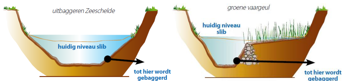
Figuur 5-3 Mogelijke opties herstellen bevaarbaarheid Zeeschelde Gentbrugge-Melle
