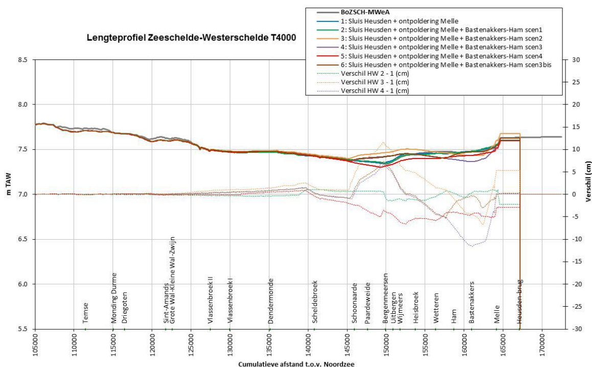
Figuur 7-34 Lengteprofiel Boven-Zeeschelde met maximale waterstanden voor het MWeA-scenario, het referentiescenario met inplanting van de sluis in Heusden in combinatie met ontpoldering te Melle en enkele scenario's voor inrichting van GOG Bastenakkers, GOG ham en GOG Heisbroek bij een terugkeerperiode van 4000 jaar
