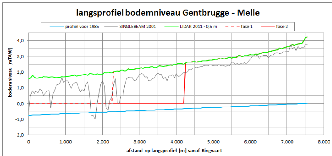
Figuur 7-11 Wijziging langsprofiel thalweg Zeeschelde tussen Gentbrugge en Melle bij onderhoudsbaggerwerken ZGM fase 1 en ZGM fase 2 (Bron: IMDC, 2011a)
