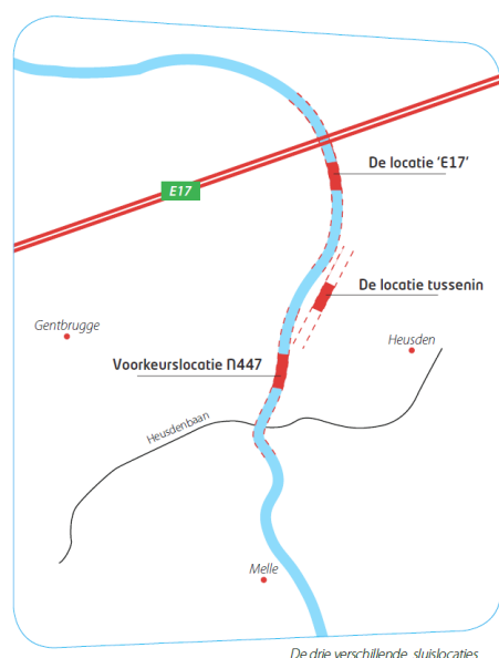
Figuur 5-4 Mogelijke sluislocaties nieuwe sluis Heusden
