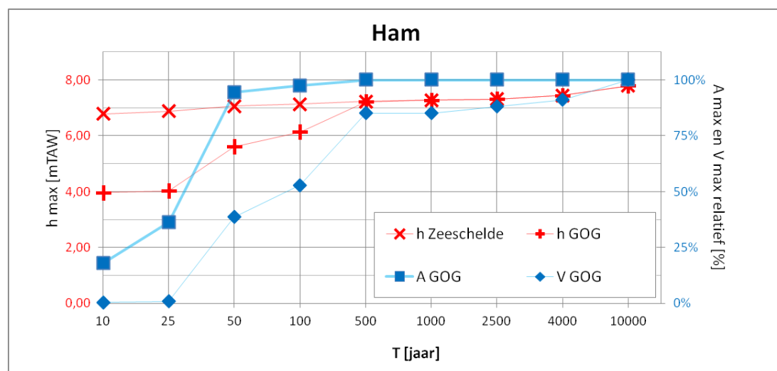
Figuur 7-38 Verwachte maximale waterstanden en percentage relatief overstromde oppervlakte (A) en volume (V) binnen GOG-GGG Ham volgens verschillende retourperioden
