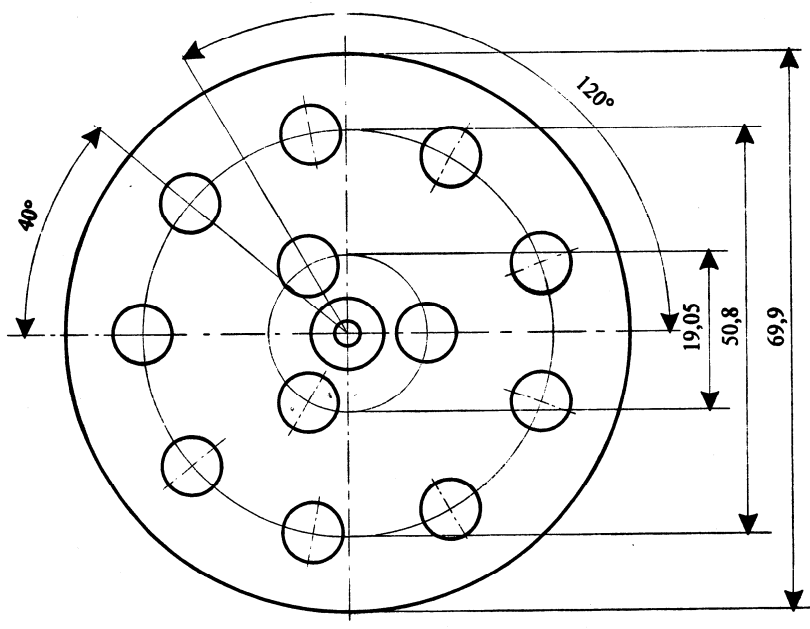
Figuur 1 Penetrometer
