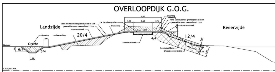
Figuur 8-23 Standaardprofiel overlooptdijk van een GOG
