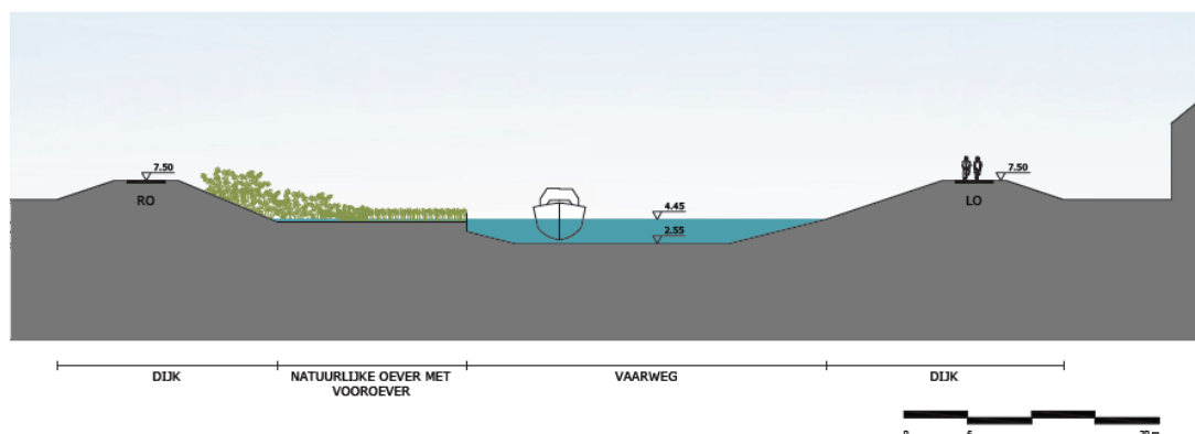
Figuur 4-4 Profiel niet-getijafhankelijk deel Zeeschelde
