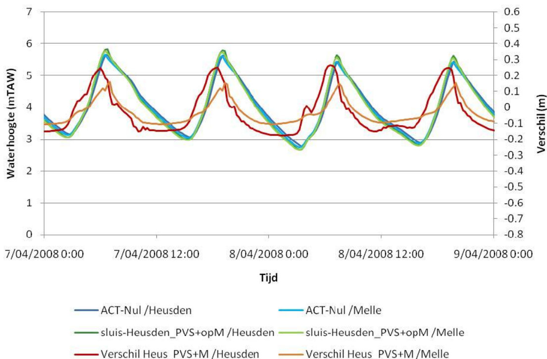
Figuur 7-31 Waterpeilen ter hoogte van Heusden en Melle voor de actuele situatie en voor het scenario met de sluis ter hoogte van Heusden en profiel “passagiersvaart-scenario” en de ontpoldering in Melle gecombineerd met de waterpeilverschillen tussen de 2 situaties, voor 2 dagen begin april 2008
