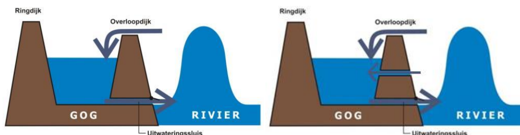
Figuur 4-12 Werkingsprincipe GOG (links) en GOG-GGG (rechts)
