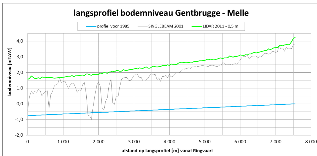
Figuur 7-7 Evolutie langspaniel talweg Zeeschelde tussen Gentbrugge en Melle (Bron: IMDC, 2011a)
