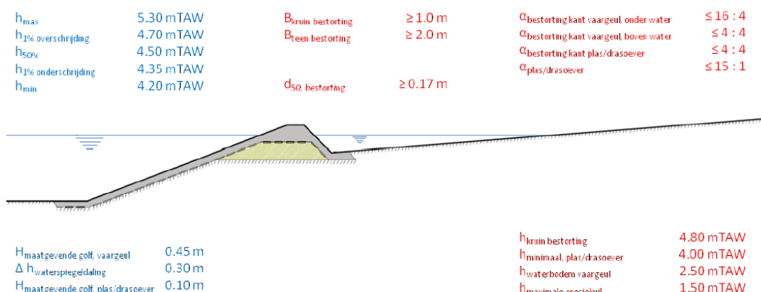
Figuur 4-5 Schematisch voorontwerp plas/dras oever met vooroeverdam
