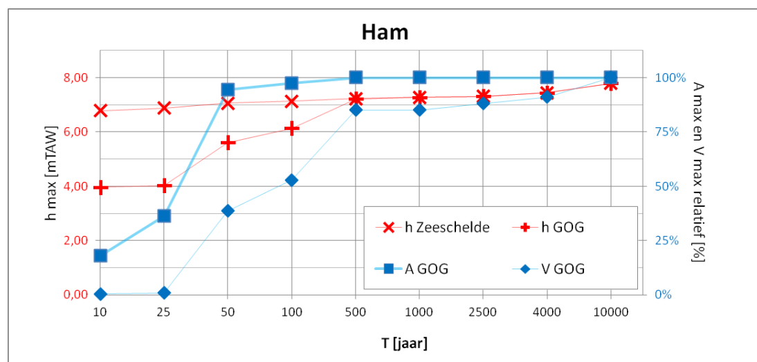
Figuur 7-38 Verwachte maximale waterstanden en percentage relatief overstroomde oppervlakte (A) en volume (V) binnen GOG-GGG Ham volgens verschillende retourperioden
