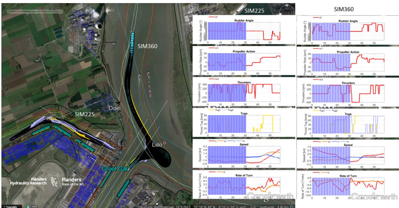
Figuur 12 - Gekoppelde simulatie VP9_3004: minuut 1 tot 30
