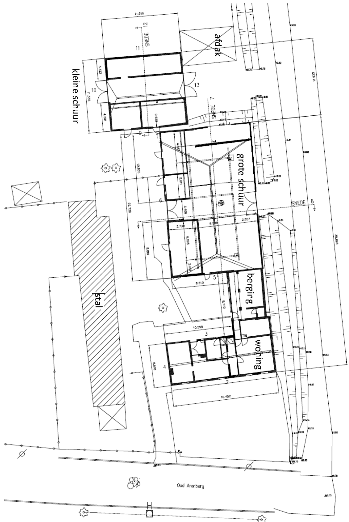
Figuur 297 Oud Arenberg 111: inplantingsplan (eigen opmeting)
