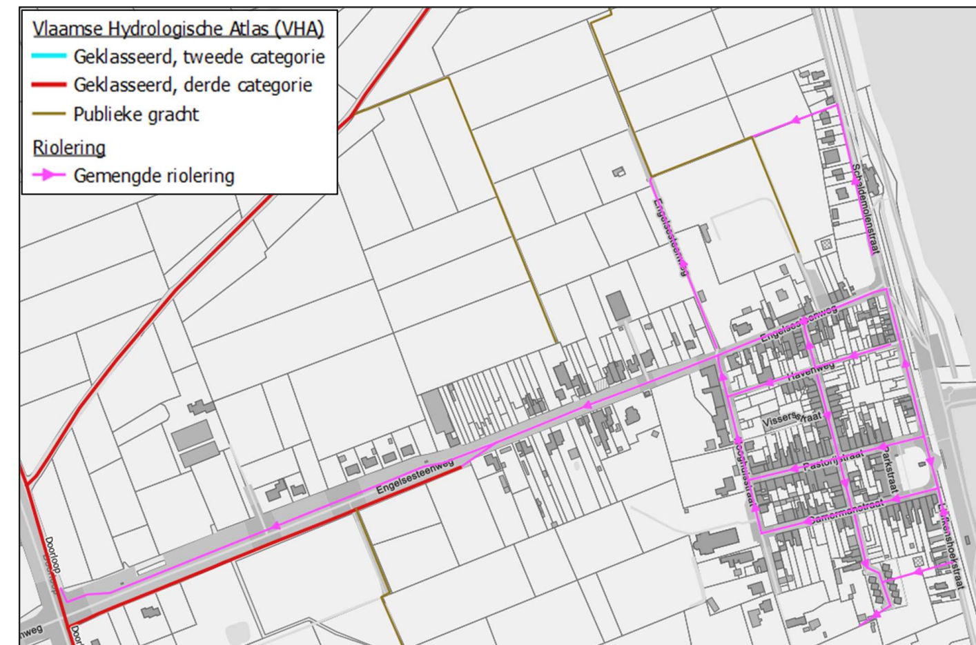
figuur 2. Overzicht van het rioleringsstelsel in Doel, gebaseerd op het TRP van 1982
