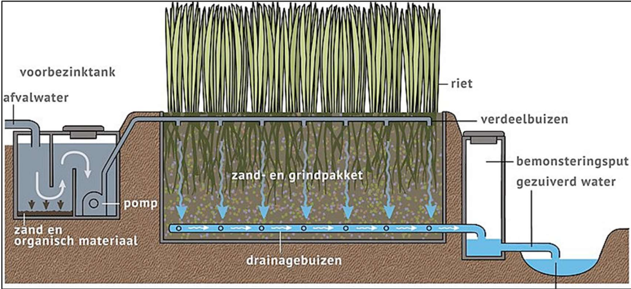
figuur 16. Principetekening van een percolatie(riet)veld
