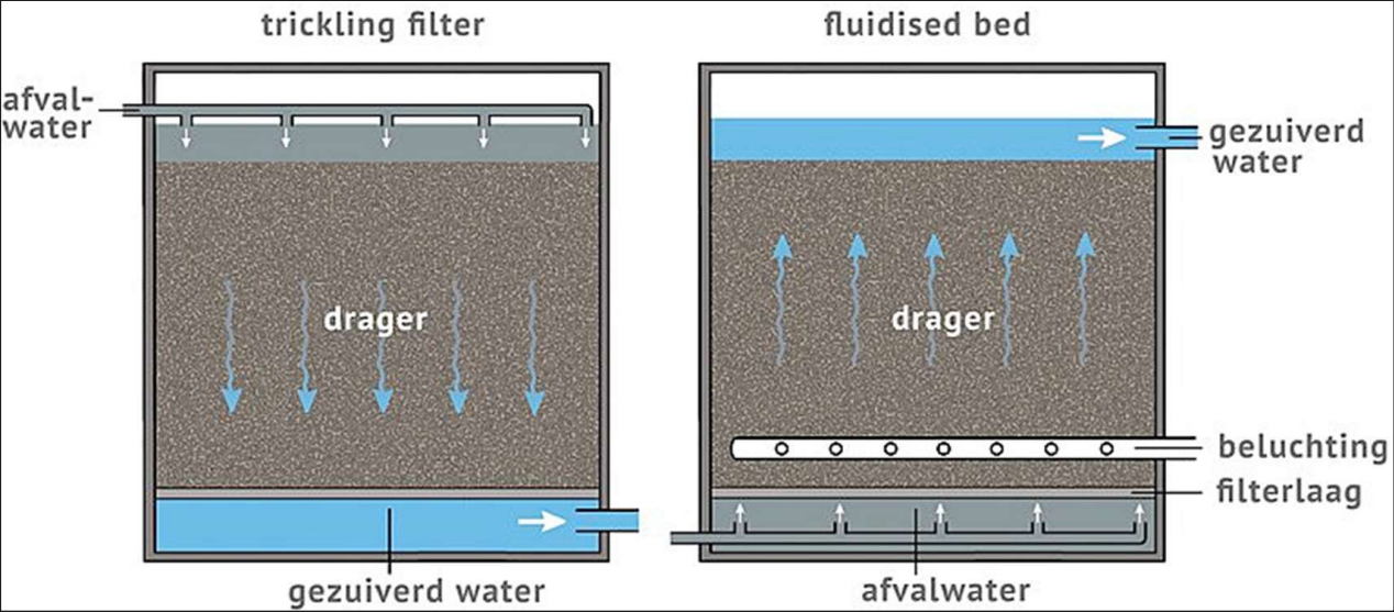
figuur 15. Principeschets van een Submerged Aërated Filter © Saniwijzer
