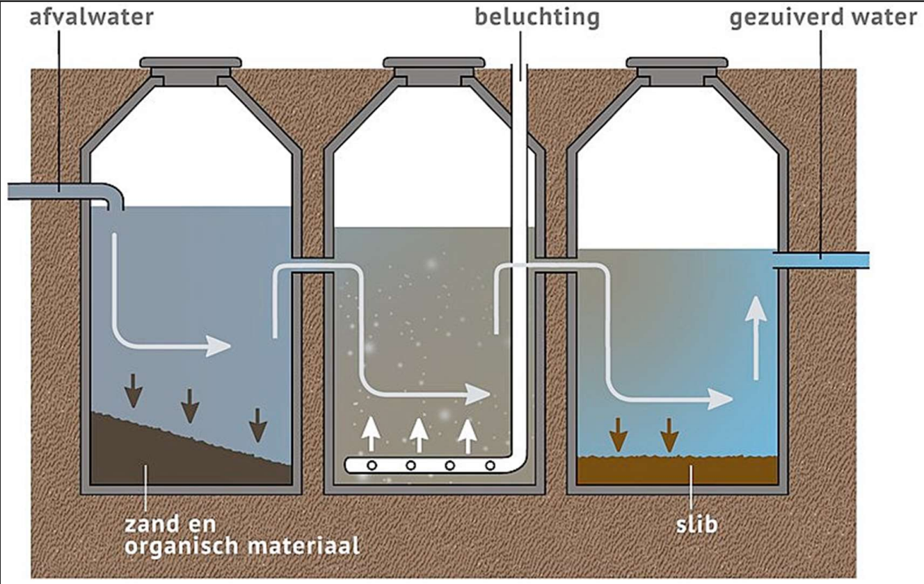
figuur 13. Principeschets van een actiefslibstelsysteem © Saniwijzer
