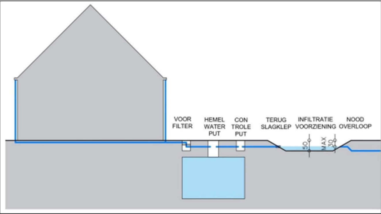
figuur 25. Principetekening voor beheer van het hemelwater op een privaat perceel © Coördinatiecommissie Integraal Waterbeleid
