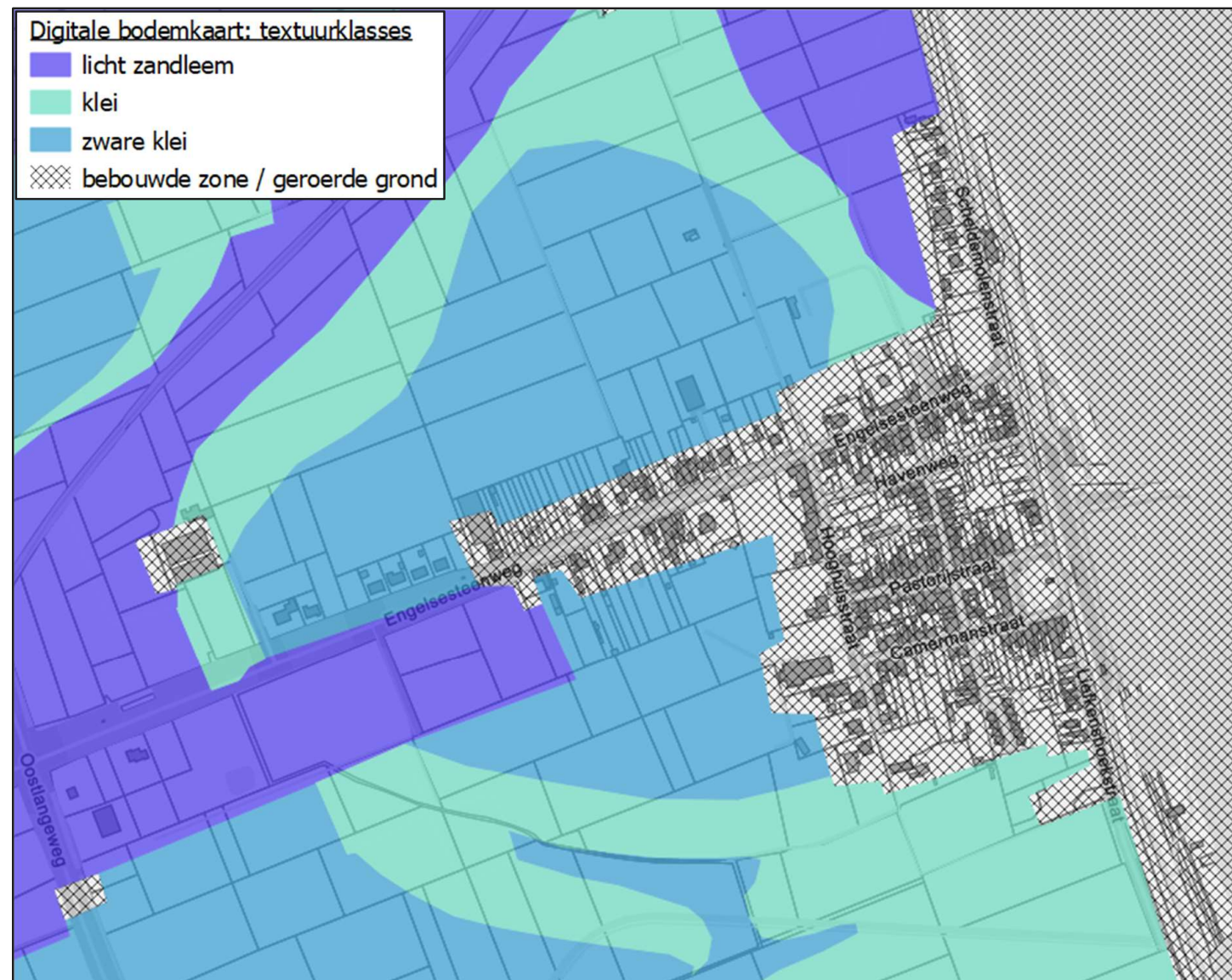
figuur 4. Textuurklassen van de bodem van Doel © Databank Ondergrond Vlaanderen
