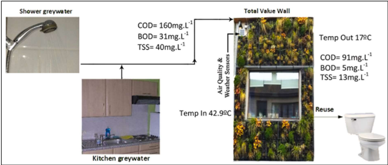
figuur 24. Visualisatie van de werking van een filterende groene gevel © Vlakwa
