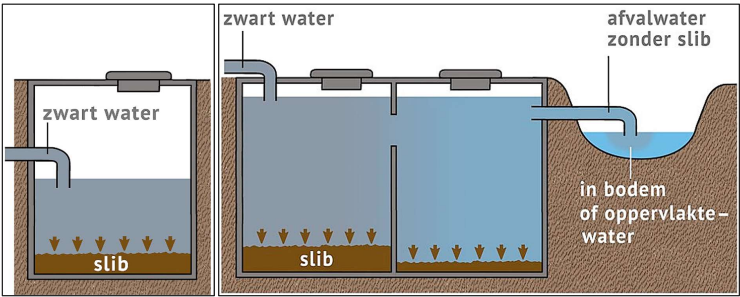
figuur 12. Links een beerput zonder overloop, rechts een septische put met meerdere compartimenten en een overloop © Saniwijzer
