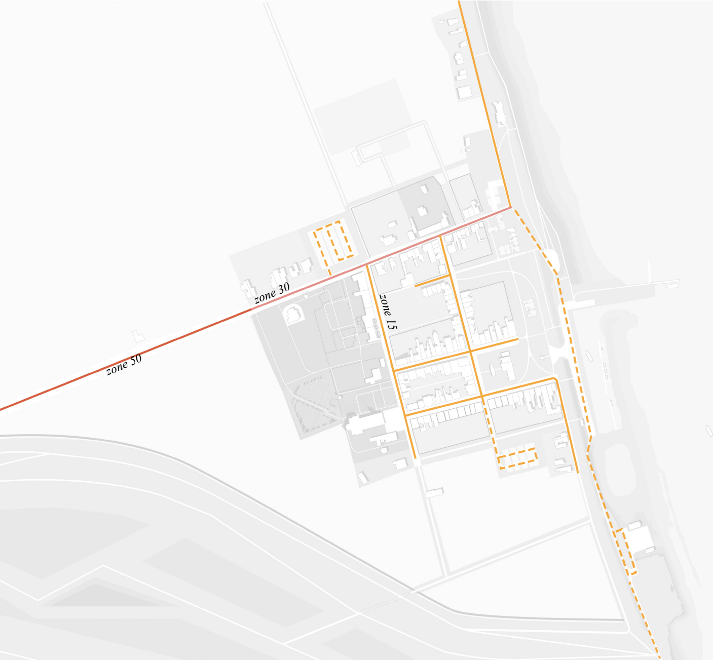
figuur 42 Voorgestelde autosnelheden in zone 50, 30 en 15.
