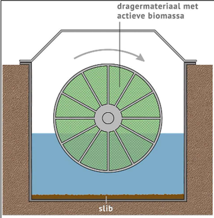
figuur 14. Principetekening van een Rotating Biological Contactor © Saniwijzer
