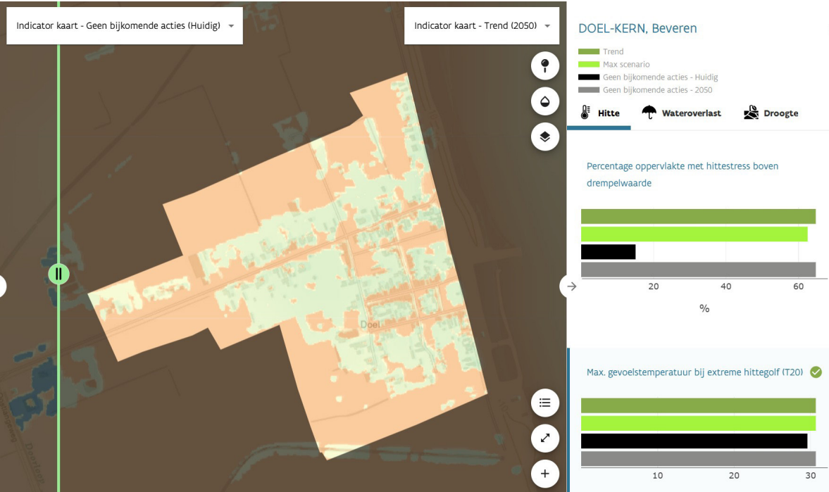
figuur 39 Percentage oppervlakte hittestress boven de drempelwaarde (bron: PLAN-tool: verken adaptatiemaatregelen - VMM - Vlaanderen).
