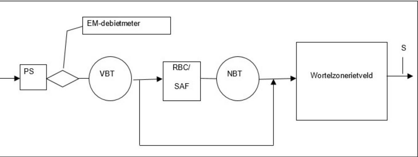
figuur 17. Schematische voorstelling van het hybride zuiveringsconcept © Aquafin
