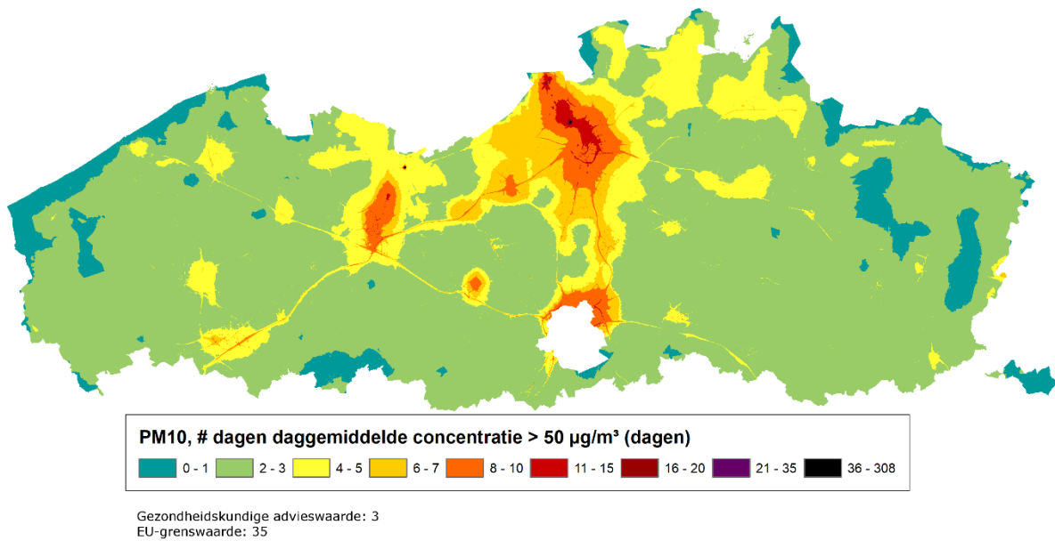
Figuur 21: Gemodelleerd aantal dagen met een daggemiddelde concentratie > 50 \mu\text{g}/\text{m}^3 PM 10 in 2030 volgens het scenario zonder bijkomend beleid zoals berekend met het AURORA-RIO-IFDM-OSPM-model
