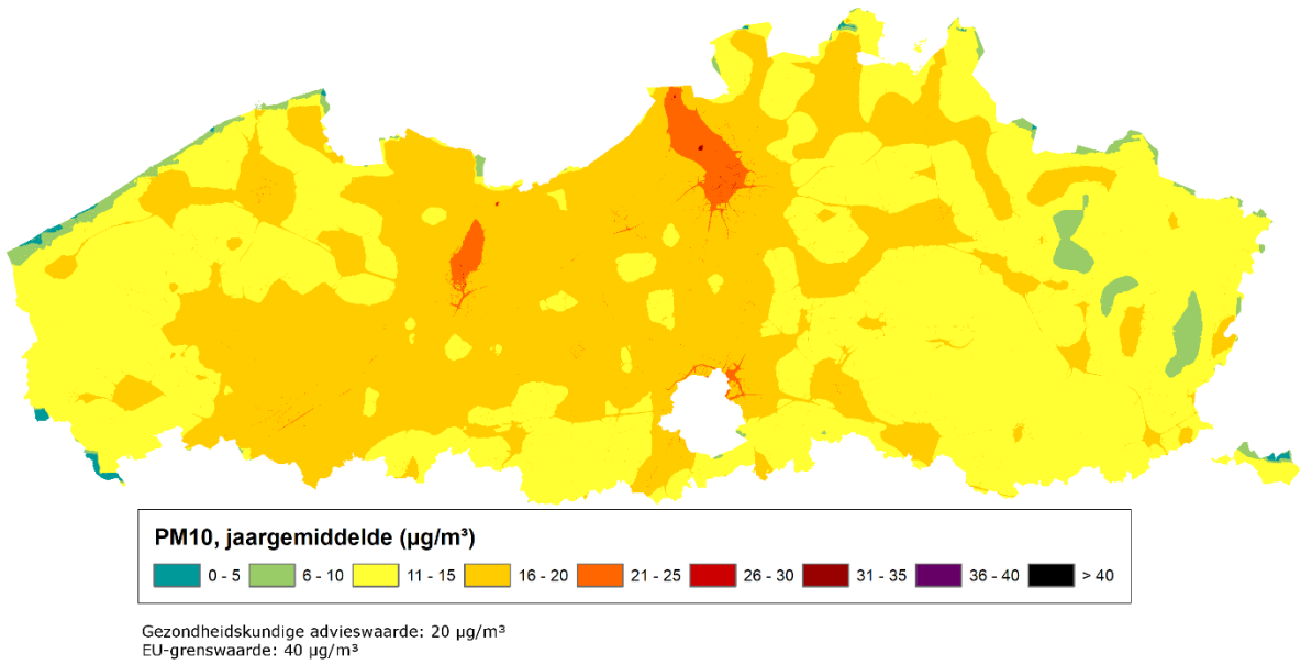
Figuur 20: Gemodelleerde jaargemiddelde PM 10 -concentratie in 2030 volgens het scenario zonder bijkomend beleid zoals berekend met het AURORA-RIO-IFDM-OSPM-model
