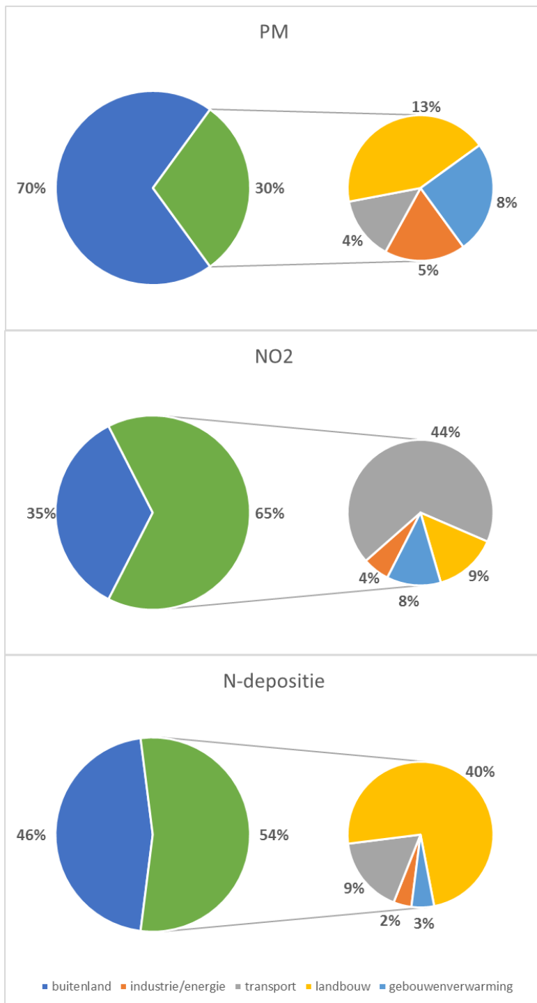
Figuur 1: Bijdrage van emissies uit het buitenland en van emissies van de Vlaamse sectoren in de concentraties van PM en NO 2 en in de N-depositie
