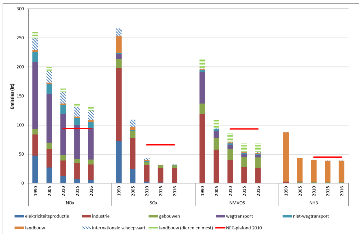
Figuur 3: Evolutie van de emissies van \text{NO}_x , \text{SO}_x , NMVOS en \text{NH}_3 over de periode 1990–2016 en vergelijking met de NEC-plafonds
