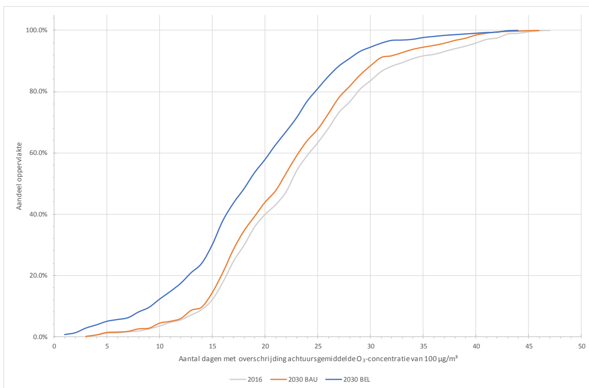
Figuur 57: Gesommeerde oppervlakte (als percentage van het totale Vlaamse grondgebied) van het aantal dagen met overschrijding van een achtuurgemiddelde O_3 -concentratie van 100 \mu\text{g}/\text{m}^3 in 2016, in 2030 onder het scenario zonder bijkomende maatregelen en in 2030 onder het scenario met bijkomende maatregelen.
