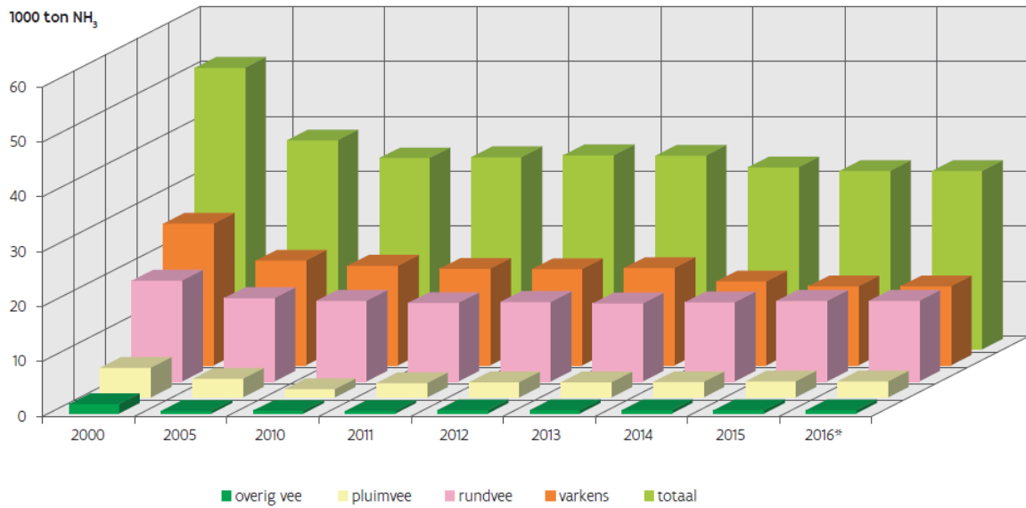
Figuur 32: Evolutie van de NH 3 -emissie (kt) door de verschillende diersoorten in Vlaanderen, over de periode 2000–2016 (* stand van zaken 30 september 2017)
