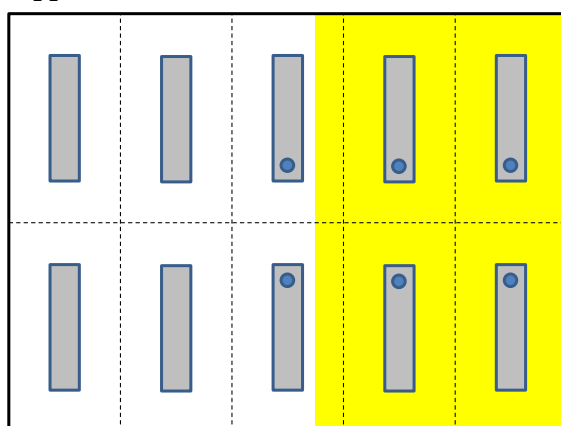
Figuur [2]: Configuratie waarbij niet alle armaturen worden bediend door eenzelfde dimsysteem - de daglichtoppervlakte ligt volledig binnen de gebruiksoppervlakte die bediend wordt door het systeem
